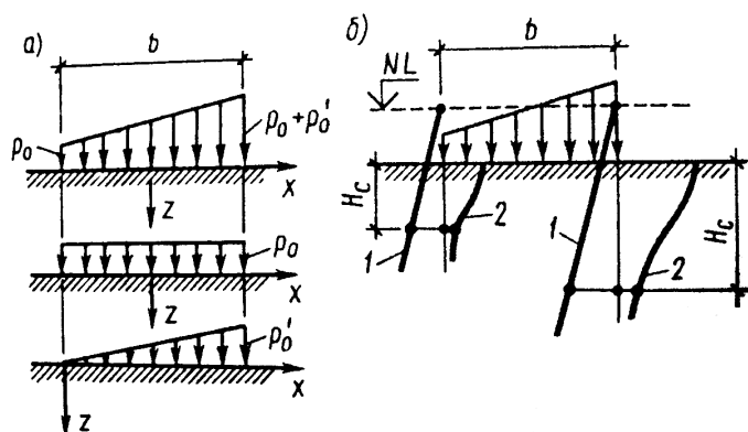
5.3-rasm. Notekis cho‘kislarni aniqlash uchun hisobiy sxemalar.
