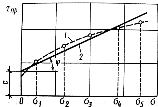
2.11-rasm. Changsimon-loyli grunt namunalarning siljishga qarshilik grafigi:
