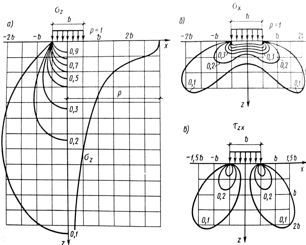
3.7-rasm. Tekis masala holati uchun zo'riqlarning izo chiziqlari va yuklangan tasma o'qi bo'ylab vertikal siquvchi zo'riqlar epyurasi.
