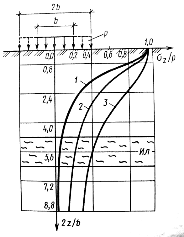
3.10-rasm. Poydevor ostining shakli va yuzasiga qarab \sigma_z zo'riqlarining poydevor o'qi bo'ylab taqsimlanish xususiyati.
