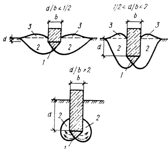
4.2-rasm. Poydevor ostining nisbiy chuqurligi har xil boʻlgan holda zaminda chegaraviy muvozanat sohalarining shakllanishi:
