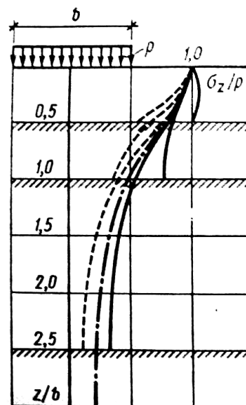
3.11-rasm. To'shama qatlam har xil chuqurlikda joylashgan holda \sigma_z zo'riqlarining poydevor o'qi bo'ylab taqsimlanish xususiyati.
