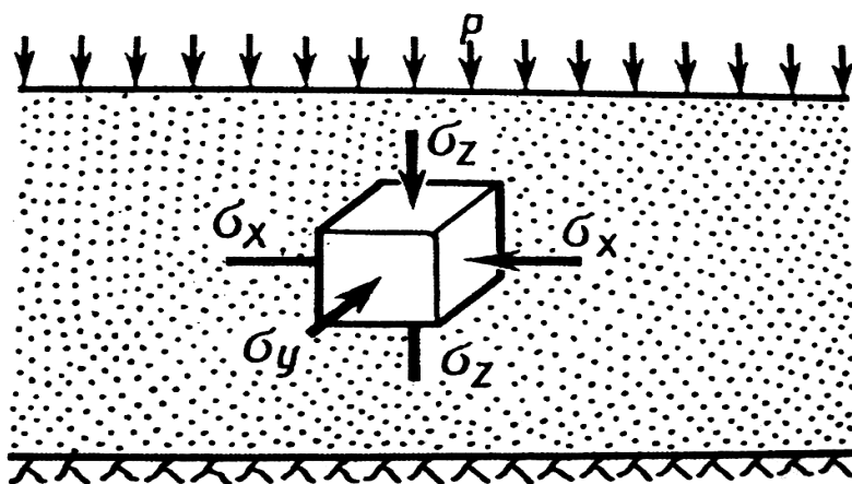
2.6-rasm. Ta'sir ostida grunt elementidagi zo'riqlashlar sxemasinamunasi.
