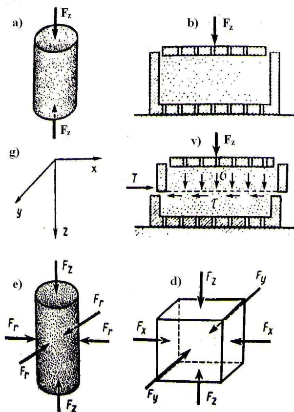
2.1-rasm. Grunt namunalari sinashning asosiy sxemalari:
