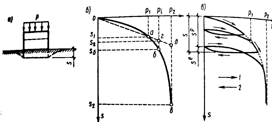
1.3-rasm. Qolip cho‘kishi tajribasi (a) va uning yuklanishda (b) va yuklanish-yuksizlanishda qolipcho‘kishining ost bo‘ylab uzatiluvchi bosim p ga bog‘liqlik grafiklari:
