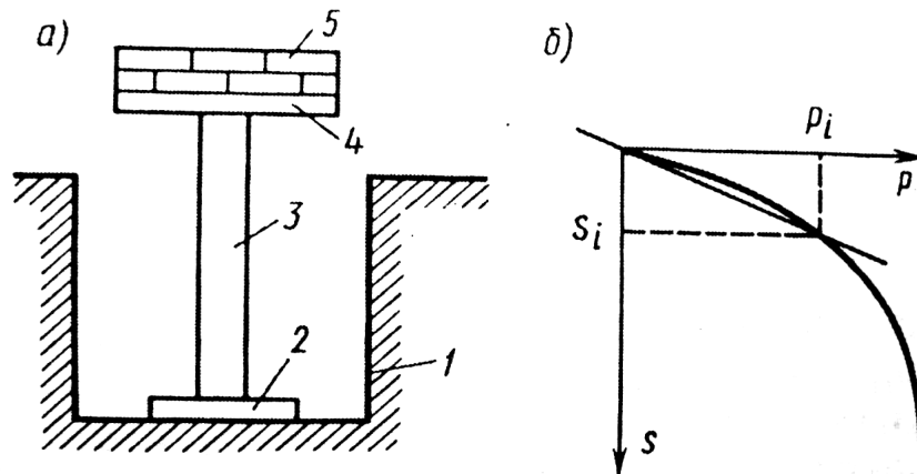
2.14-rasm. Grunt da siqish yo'li bilan o'tkaziluvchi dala sinovlari sxemasi (a) va natijalari (b).
