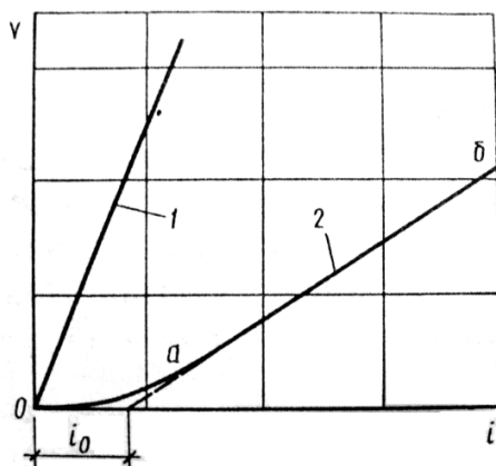
2.8-rasm. Gruntidagi filtratsiya tezligining gidravlik gradiyentga bog'liqligi.
