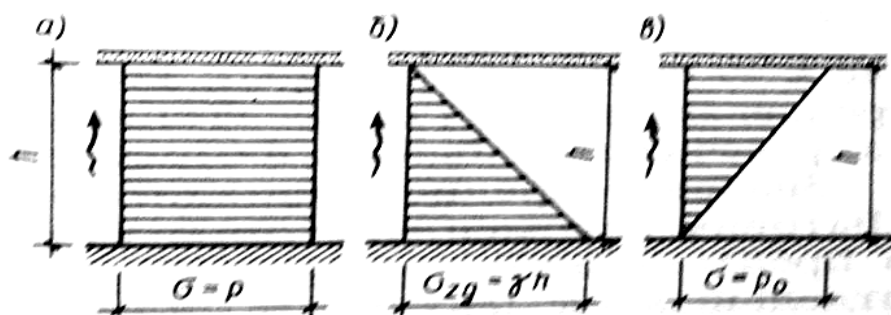
5.4-rasm. Quyidagi holatlar uchun zichlovchi kuchlanishlarning epyuralari: a – 0; b – 1; v – 2
