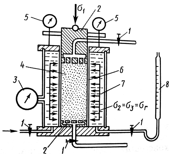
2.12-rasm. Stabilometr sxemasi
