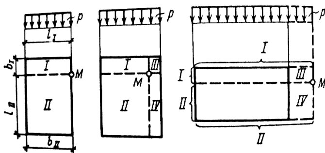
3.9-rasm. Zo'riqishlarni burchak nuqtalari usuli bilan hisoblash sxemasi
