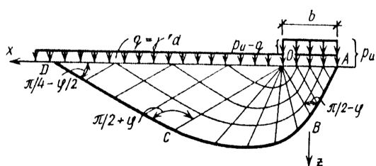
4.4-rasm. Vaznsiz ( \gamma=0 ) zamin uchun chegaraviy qo'shimcha yuk tushgan holda sirpanish chiziqlari
