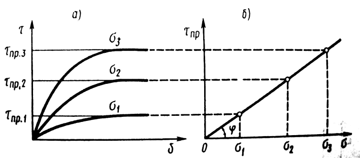
2.10 -rasm. \sigma ning har xil qiymatlarida namunalar gorizontal siljishlarining egri chiziqlari (a) va qumli grunt namunalarining siljishga qarshilik grafigi (b)
