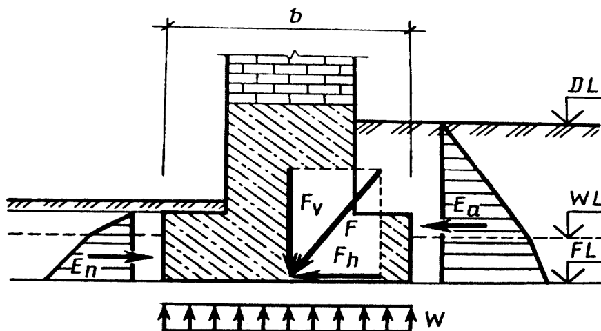
4.6-rasm. Poydevorni tekislik bo‘ylab siljishga hisoblashga doir sxema.
