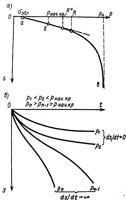
4.1-rasm. Pirovard cho‘kishning zaminga tushuvchi yukka bog‘liqligi (a) va p ning turli qiymatlarida cho‘kishning vaqtda rivojlanishi (b)
