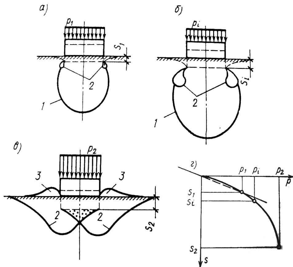
1.5-rasm. Shtamp ostida bosim kuchaygan holda zaminda gruntning chegaraviy muvozanati mintaqalarining rivojlanishi (a-v) va bunga mos tarzda shtamp cho'kishining bosimga bog'liqligi (g): 1 – gruntning zichlangan sohasi chegaralari; 2 – chegaraviy muvozanat mintaqalarida gruntning zichlangan sohasi chegaralari; 3 – o'pirilgan grunt uyumlari.
