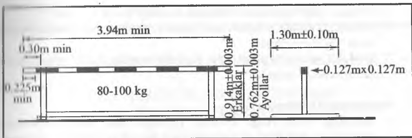
32-rasm. To'siq va uning o'lchamlari
