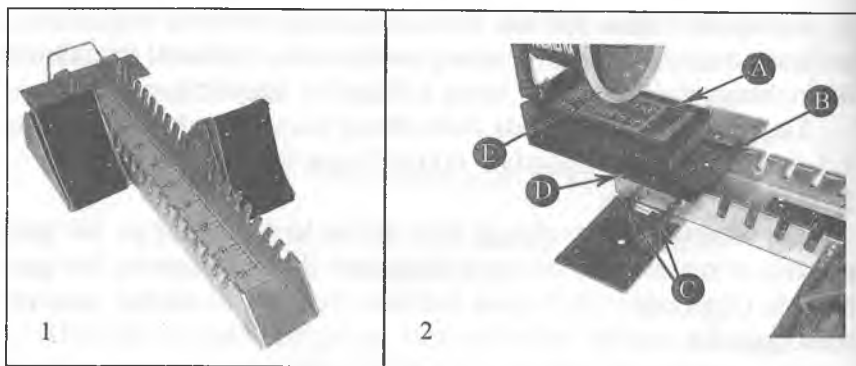
10-rasm. Start tirgaklari (1) va Falstartni qayd etuvchi moslama – ReactTime (2). A. Sensor qutisi, B. Vint, C. Qotirgichlar, D. Montaj platasi, E. Ovoz kuchaytirgich
