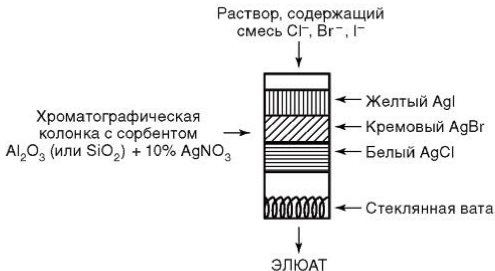
Рис. 10.7. Схема разделения ионов \text{Cl}^- , \text{Br}^- и \text{I}^- в хроматографической колонке методом осадочной хроматографии
