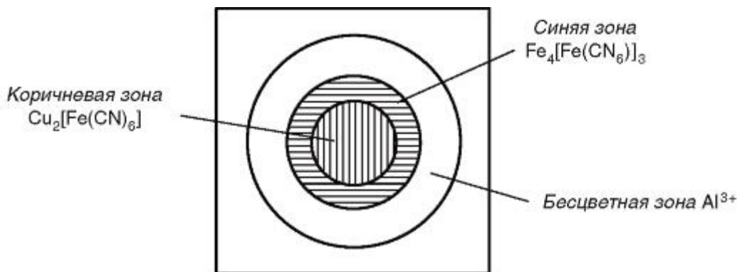
Рис. 10.8. Схема разделения \text{Cu}^{2+} , \text{Fe}^{3+} и \text{Al}^{3+} методом осадочной хроматографии
