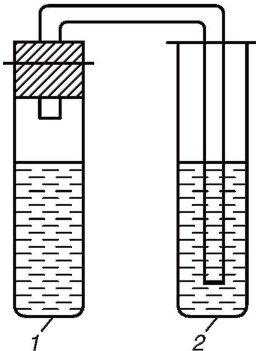
Рис. 16.1. Прибор для обнаружения газов: 1 - пробирка с анализируемым раствором; 2 - пробирка-приемник
