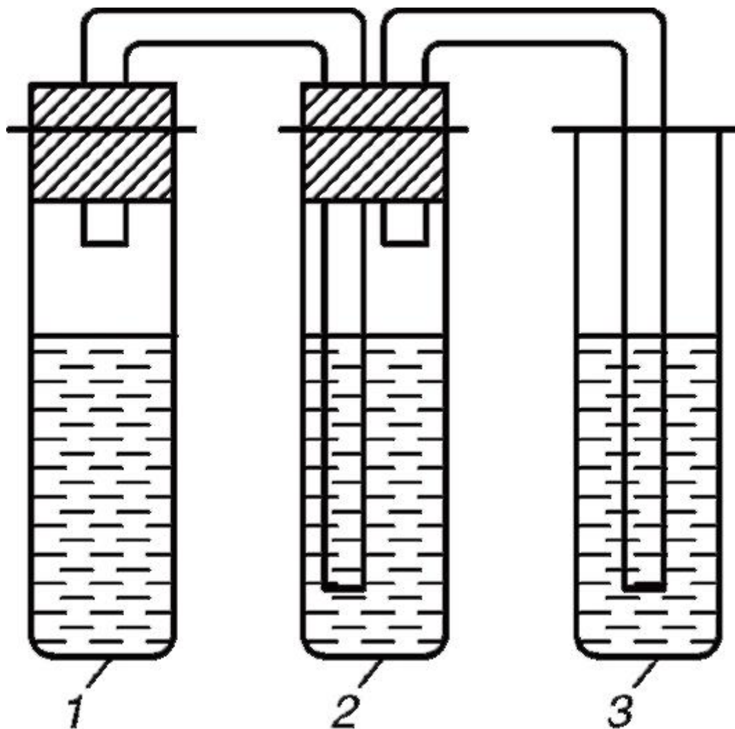
Рис. 18.1. Прибор для открытия карбонат-ионов в присутствии сульфит- и тиосульфат-ионов
