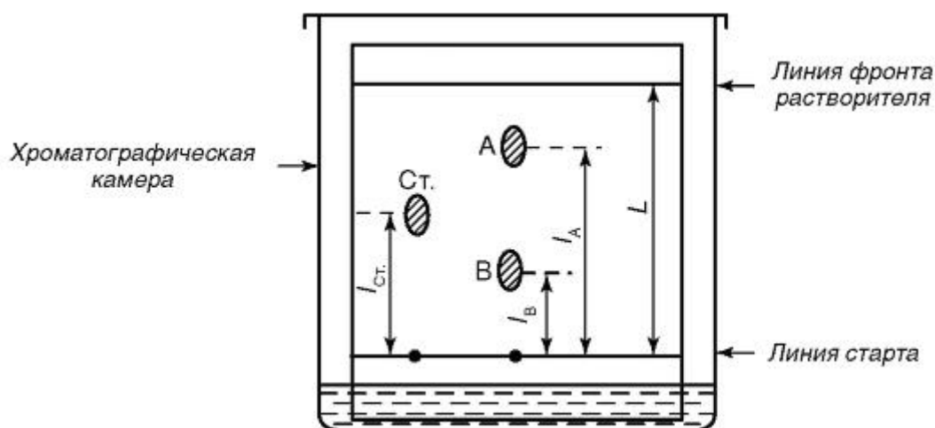
Рис. 10.4. Схема разделения компонентов А и В методом ТСХ
