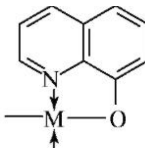
металлоцикл с депротонированным остатком 8-оксихинолина
