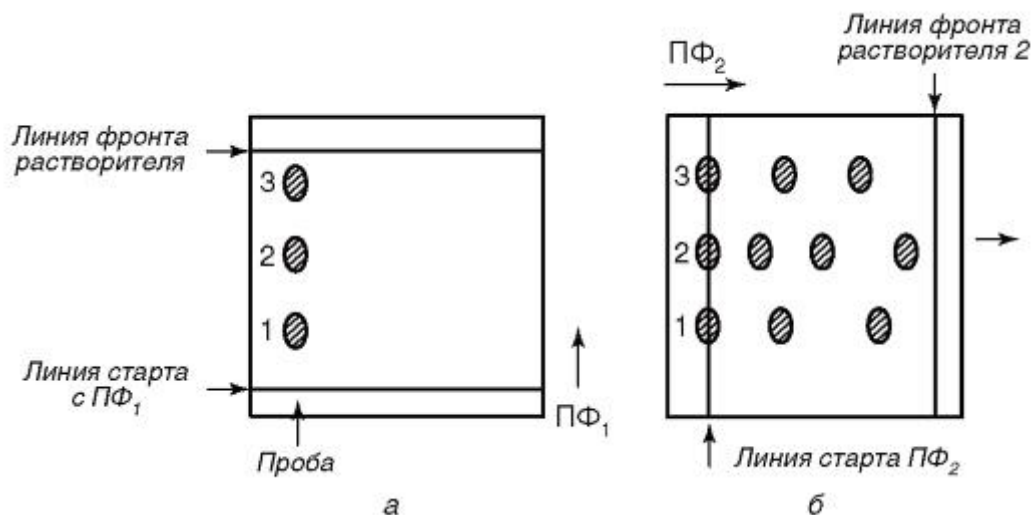
Рис. 1О.6. Схема, иллюстрирующая принцип двухмерной хроматографии:
