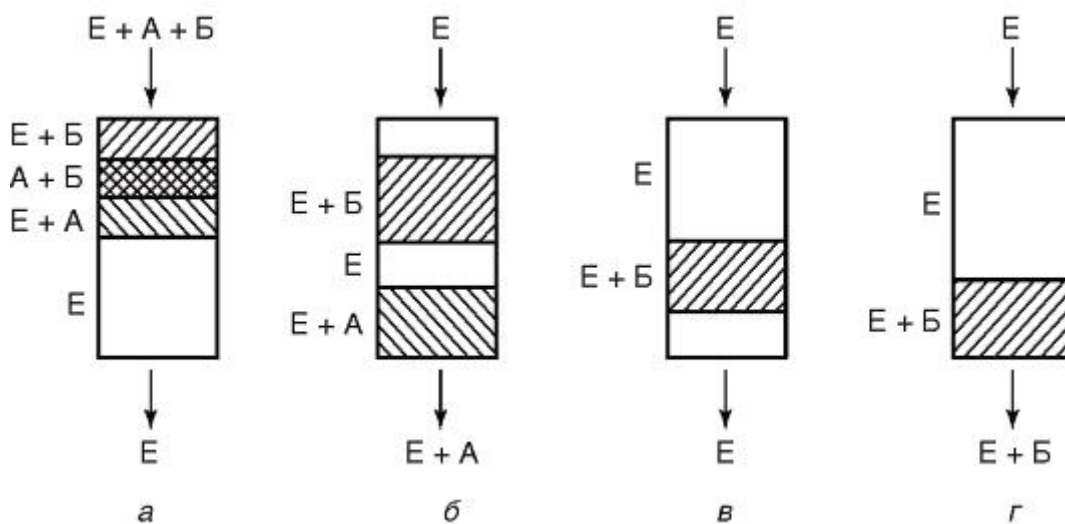
Рис. 10.2. Схема разделения компонентов в методе элюентной (проявительной) хроматографии:
