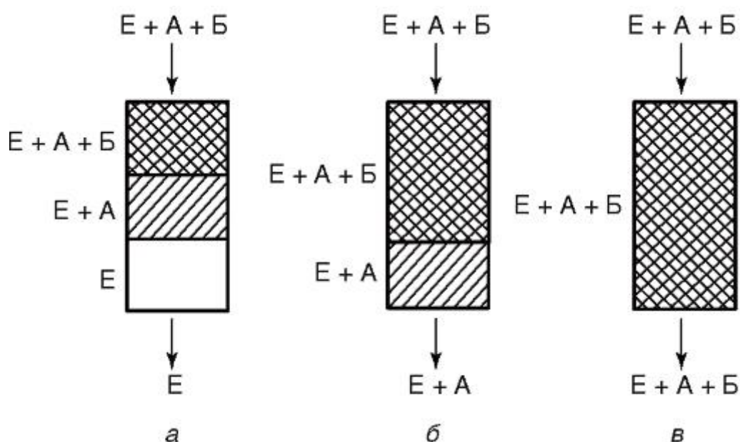
Рис. 10.1. Схема разделения компонентов смеси в методе фронтальной колоночной хроматографии:
