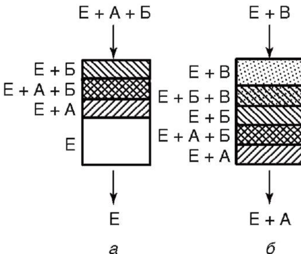
Рис. 1О.3. Схема разделения компонентов в методе вытеснительной хроматографии: а - начало процесса; б - продолжение процесса
