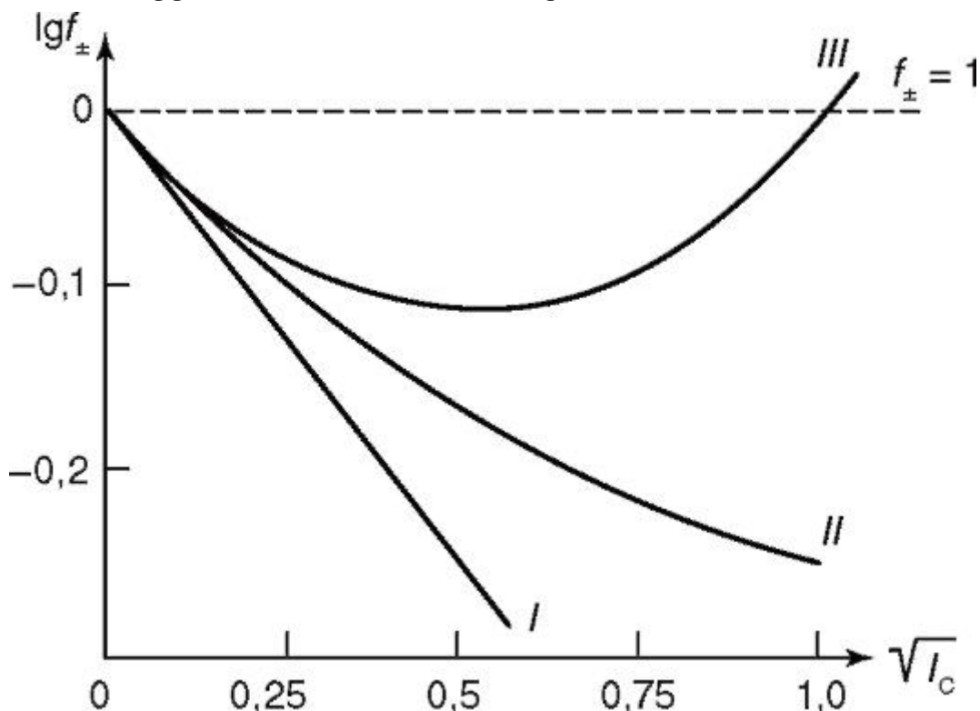
Рис. 3.1. Зависимость логарифма среднеионного коэффициента активности \lg f_{\pm} от
