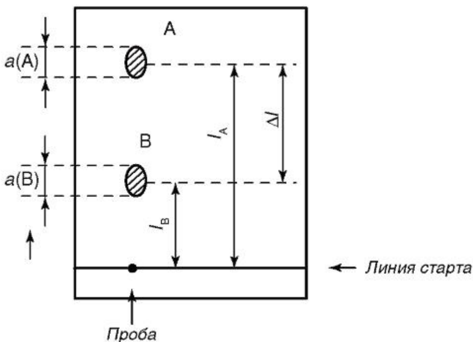
Рис. 10.5. К определению степени разделения R ( A/B ) компонентов А и В
