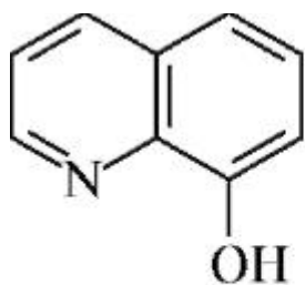
8-оксихинолин
