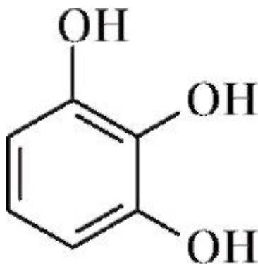
пирогалол
