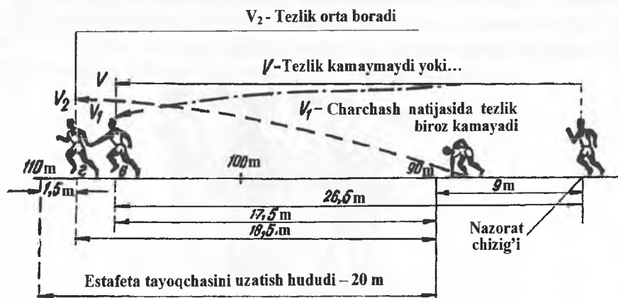
14a-rasm. Estafeta tayoqchasini qabul qiluvchi yugurishni boshlashi uchun nazorat chiziqlarini belgilash sxemasi.
