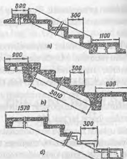
13-rasm. Yirik elementli zinlarning konstruksiyasi.
