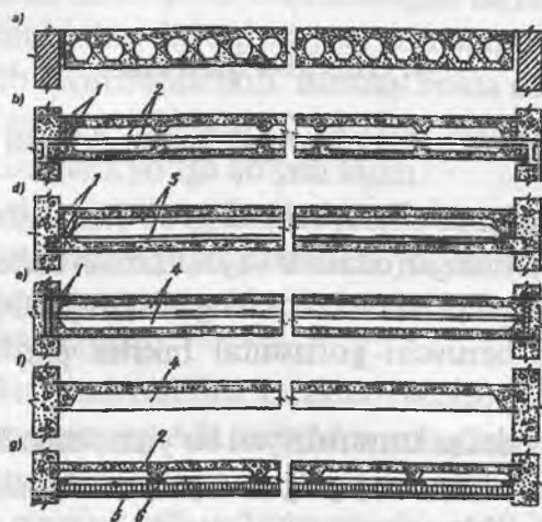
4-rasm. Yirik panelli orayopmalar.
