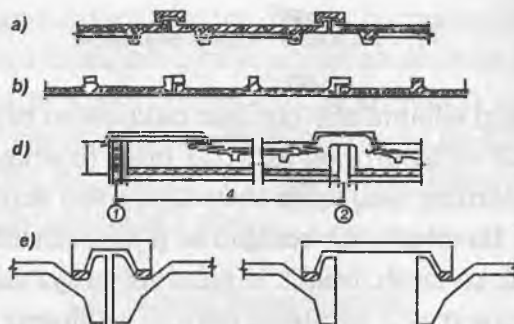
10-rasm. Rulonsiz tomqoplamalarning konstruktiv yechimlari. a — osma chekkalarida suvni chiqarib tashlovchi rombasi boʻlgan va qopqoqli yopma bilan; b — G shaklidagi orayopma bilan; d va e — oralari ochiq va birlashtirilgan shakldagi tomqoplama chokli TaShZNIIEP (UzLITTI) konstruksiyasi.
