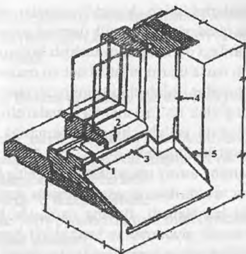
11- rasm. Deraza to'ldirmasining nuqsonlari:
