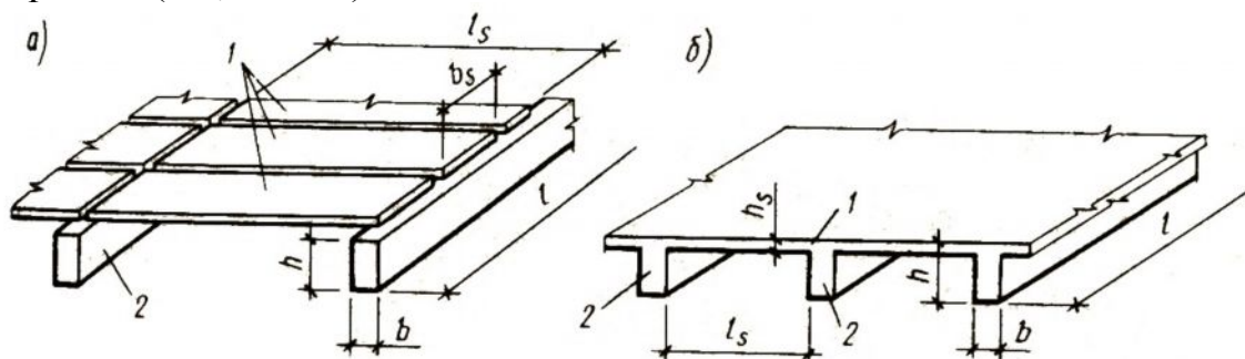
1.7-rasm. Qovurg'ali konstruktsiyalar:
