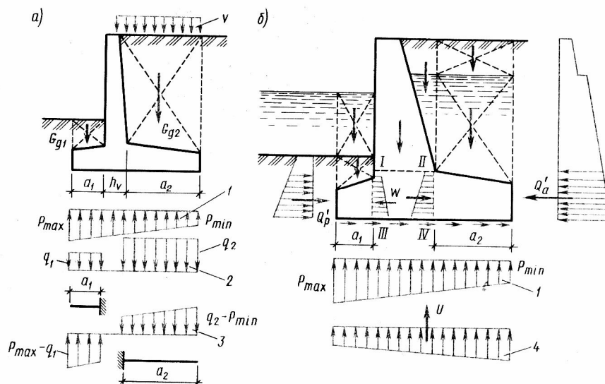
6.11-rasm. Tirgak devorlarning poydevor plitalarini hisoblash sxemalari:
