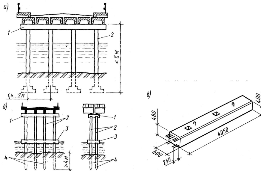
3.11-rasm. Ko'prik tayanchlari:
