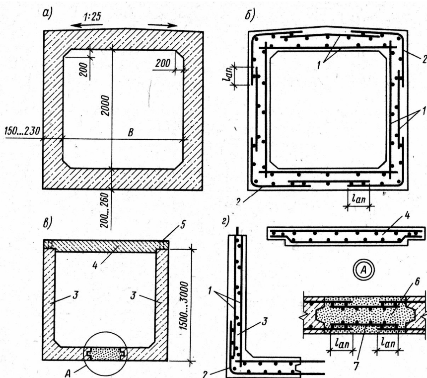
7.10-rasm. To'g'ri to'rtburchak shaklidagi bir ko'zli temirbeton quvurlar: 1 – yassi metall to'rlar; 2 – burchaksimon to'rlar; 3 – G shaklidagi bloklar; 4 – yopma plita; 5 – shponka; 6 – tutashtirish choklariga quyilgan beton; 7 – tutashtiruvchi to'rlar.
