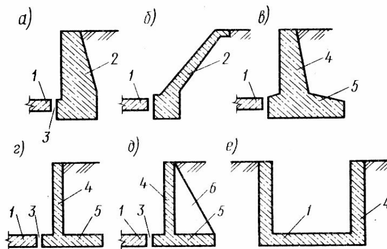
6.1-rasm. Suv tashlagich va tezoqarlar yon devorlarining turlari:
