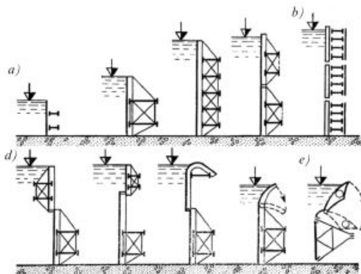
9.1-rasm. Yassi zatvorlarning asosiy turlari:
