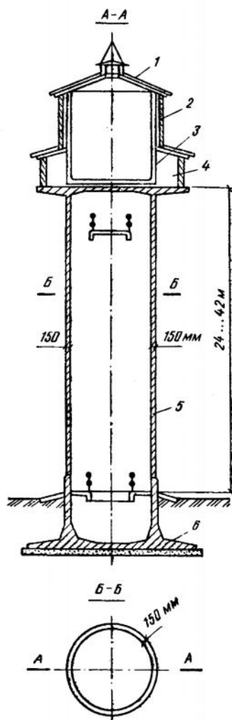
2.17-rasm. Yaxlit quyma temirbeton tayanchli bosimli suv minorasi.
