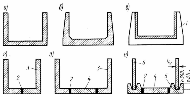
6.14-rasm. Dok konstruktsiyalarning konstruktiv sxemalari:
