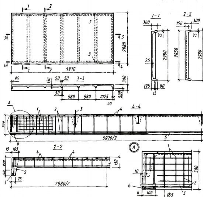
1.15-rasm. O'lchamlari 3x6 m. bo'lgan qovurg'ali temirbeton yopma plitaning konstruktsiyasi:
