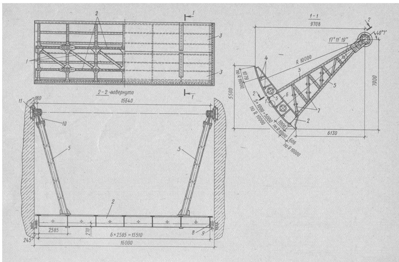
9.11-rasm. Segmentli zatvorning asosiy elementlari
