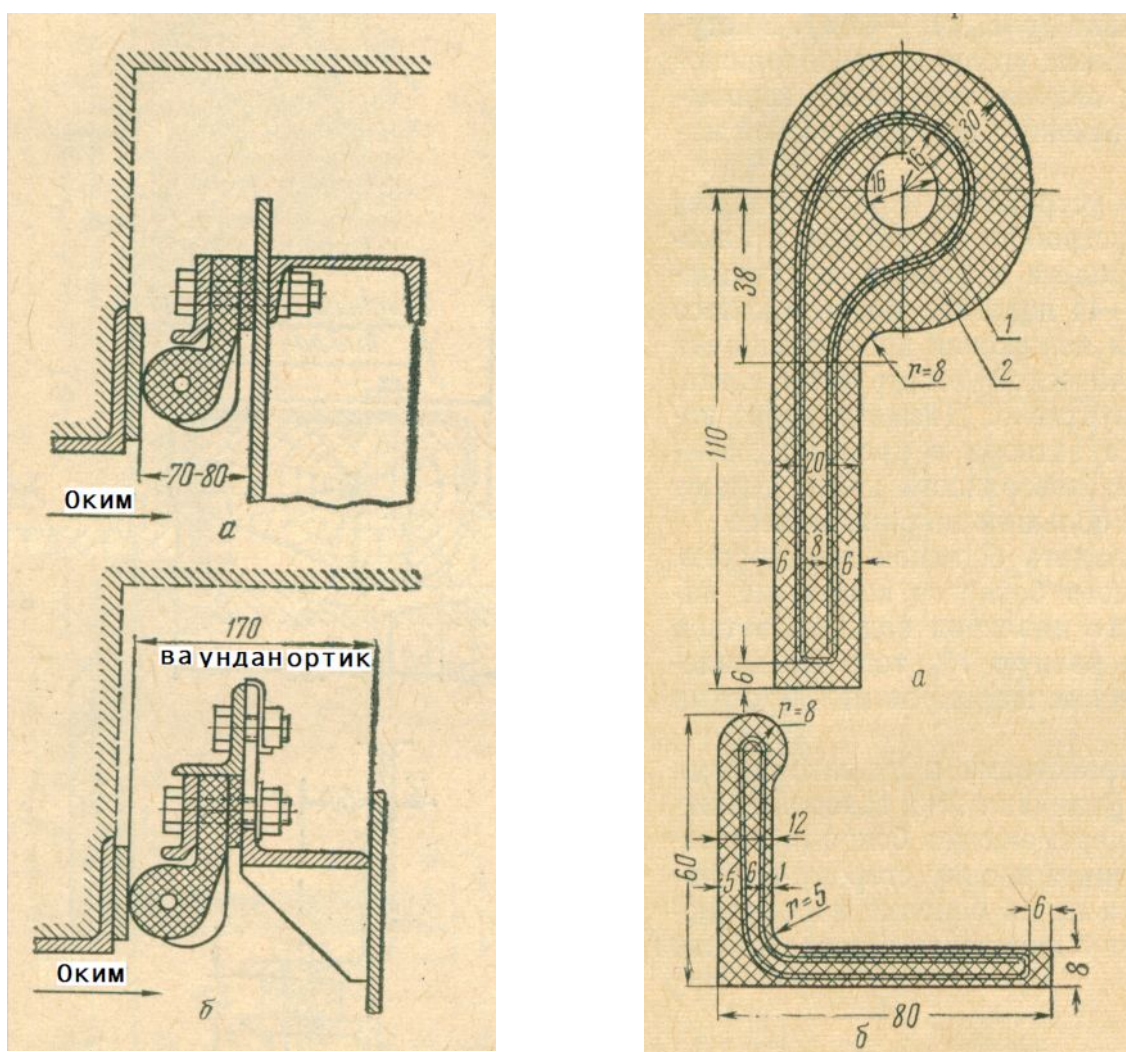
9.8-rasm. Rezina zichlagichlar va ularni o'rnatish sxemalari:
