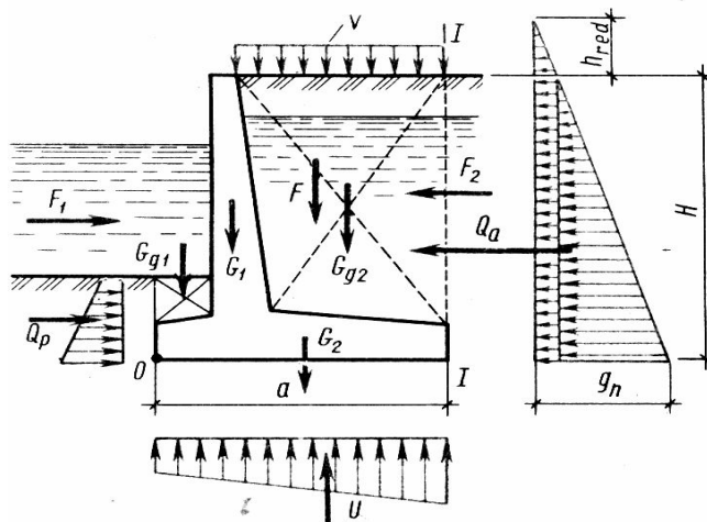
6.10-rasm. Yuklarni tirgak devorga ta'sir etish sxemasi
