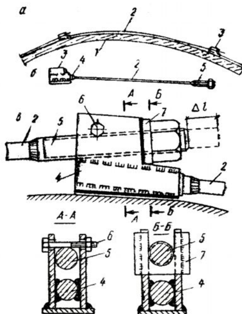
2.5-rasm. Elektrotermik usulda zo'riqtiriladigan armatura sterjenlarining detallari:
