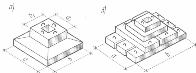
5.3-rasm. Yig‘ma poydevorlarning turlari
