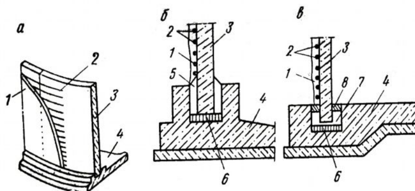
2.3-rasm. Tsilindr shaklidagi yigʻma temirbeton sigʻimning detallari:
