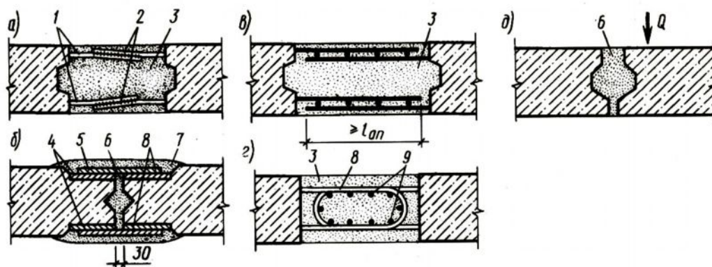
4.5-rasm. Yig'ma temirbeton plitalarni o'zaro biriktirishda qo'llaniladigan tutashmalarining turlari
