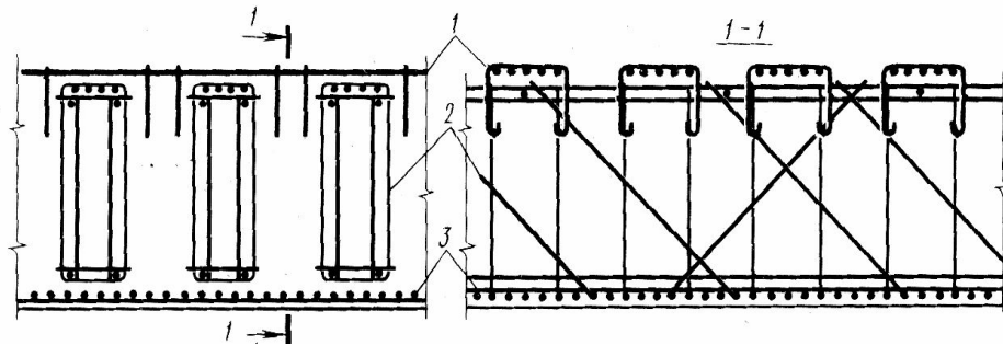
6.8-rasm. Inshootni armaturalashda armokonstruktsiyalarni joylashish sxemasi:
