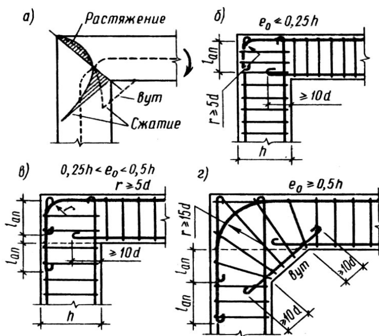
4.3-rasm. G – shaklidagi tugunlarning kirish burchaklaridagi siqilgan qismlarini aramturalash
