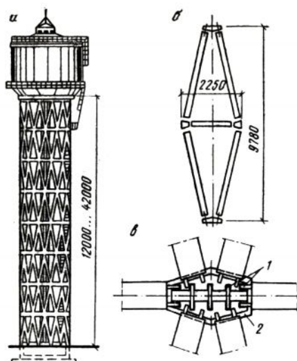
2.19-rasm. To‘rsimon yig‘ma temirbeton tayanchli bosimli suv minorasi.
