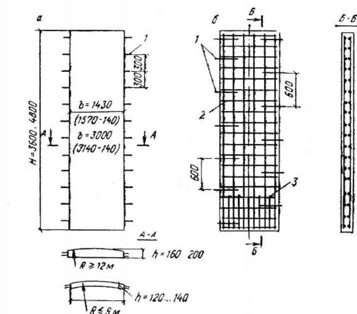
2.4-rasm. Silindr shaklidagi sig'imlarning devor panellari:
