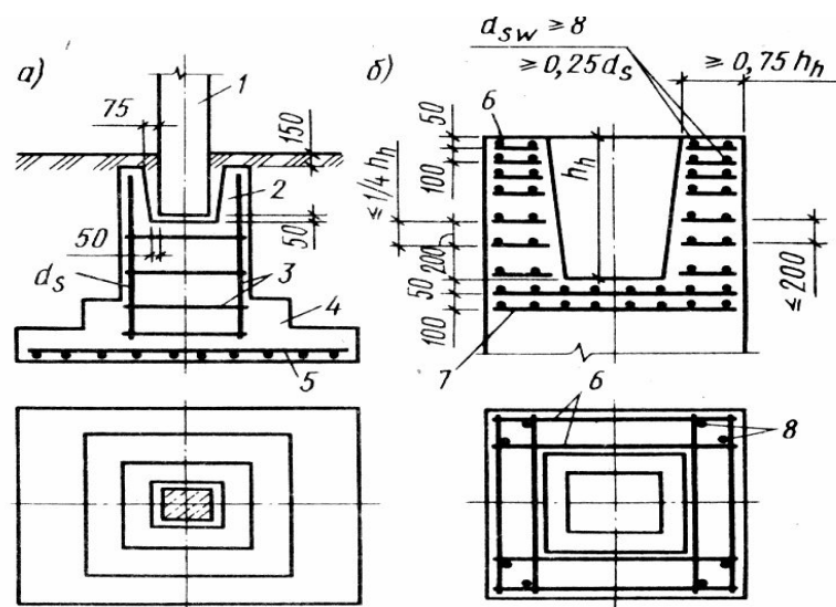
5.6-rasm. Stakan ko‘rinishidagi maxsus chuqurchali bir butun quyma poydevor.
