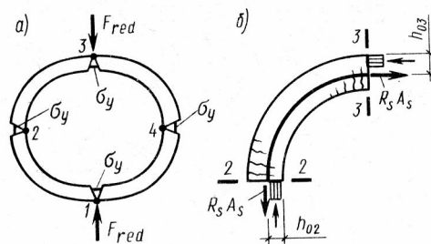
7.8-rasm. Bosimsiz quvurlarning chegaraviy muvozanat bosqichida mustahkamligini hisoblash sxemalari
