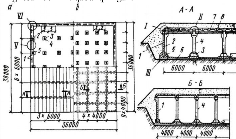
2.10-rasm. Prizma shaklidagi yig'ma temirbeton sig'im:
