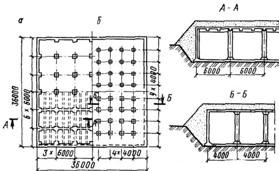
2.9-rasm. Prizma shaklidagi yaxlit quyma temirbeton sig'im:
