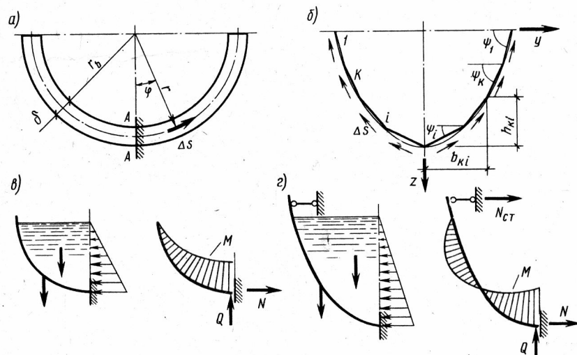
8.5-rasm. Temirbeton novlarning hisoblash sxemalari:
