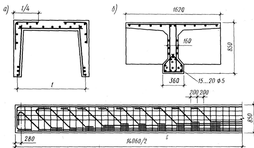
3.10-rasm. Asosiy to‘sinlarni armaturalash sxemalari
