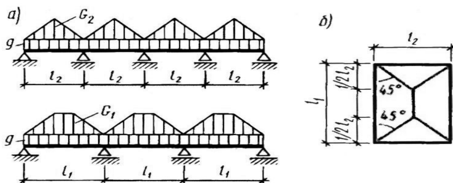
1.10-rasm. Qovurg'ali konstruktsiyalarda konturi bilan tayangan plitalar orqali yuklarni to'sinlarga uzatish sxemalari.
