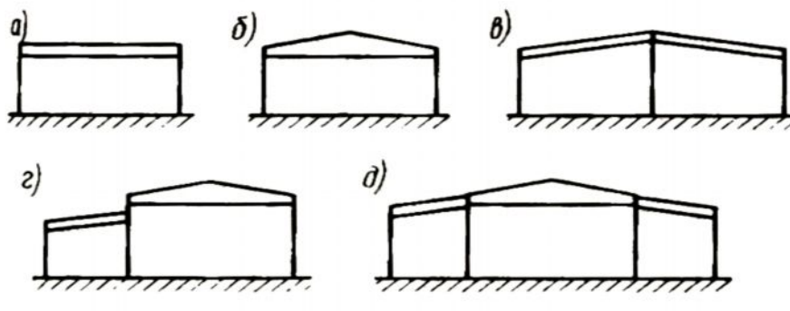
1.11-rasm. Bir qavatli ishlab chiqarish binolarining konstruktiv sxemalari
