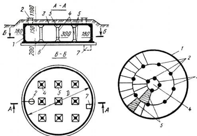
2.1-rasm. Silindr shaklidagi to'sinsiz ustyopmani yaxlit quyma temirbeton sig'im 1 - sig'im devori; 2 - lyuk; 3 - to'sinsiz ustyopma; 4 - kolonnalar; 5 - kolonnalarning kengaytirilgan qismi (kapitel); 6 - inshoot tubi; 7 - chuqurcha.
