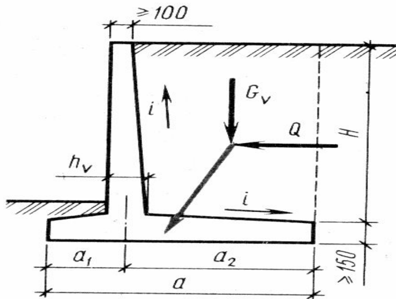
6.2-rasm. Burchaksimon tirkak devor
