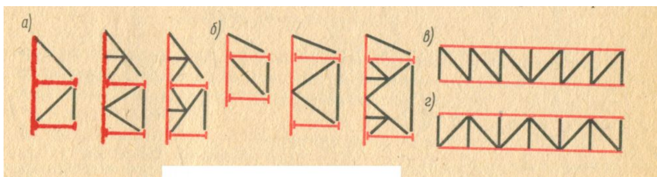
9.16-rasm. Yassi zatvorlarning ko'ndalang va bo'ylama bog'lam fermalari
