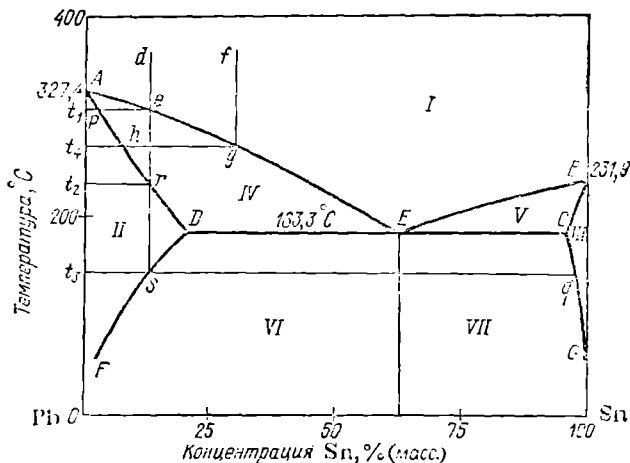
Рис. 151. Диаграмма состояния системы Pb—Sn.
