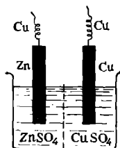
Рис. 82. Схема медно-цинкового гальванического элемента.
