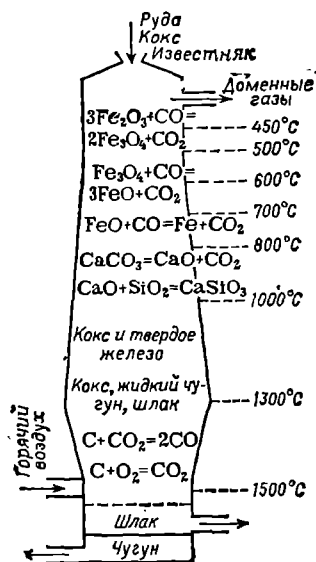
Рис. 172. Схема химических реакций, протекающих в различных частях доменной печи.
