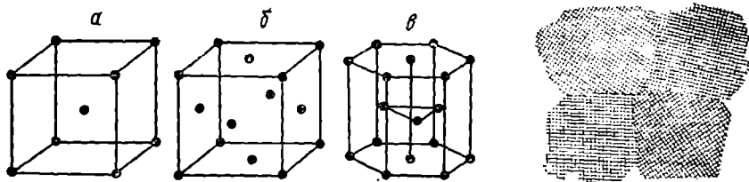
Рис. 139. Основные типы кристаллических решеток металлов:
