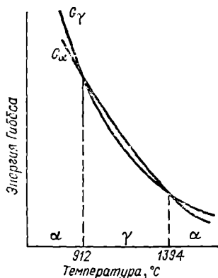
Рис. 166. Температурная зависимость энергии Гиббса α-железа ( G_\alpha ) и γ-железа ( G_\gamma ).
