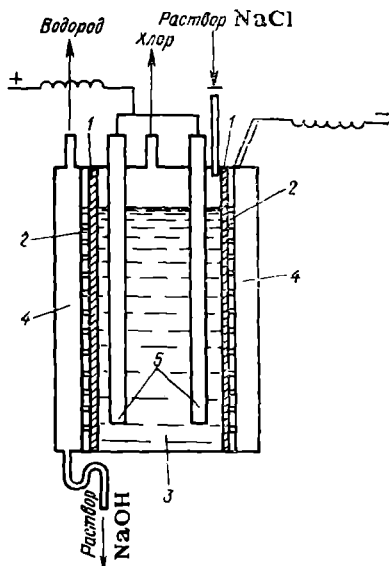
Рис. 154. Схема электролизера с вертикальной диафрагмой:
