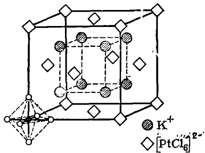
Рис. 159. Кристаллическая решетка K_2[PtCl_6] .
