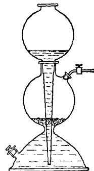
Рис. 105. Аппарат Киппа.
