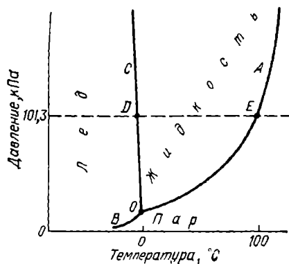
Рис. 73. Диаграмма состояния воды в области невысоких давлений.
