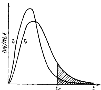
Рис. 63. Распределение молекул газа по кинетической энергии.
