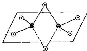
Рис. 165. Схема пространственного строения молекулы \text{Al}_2\text{Cl}_6 :
