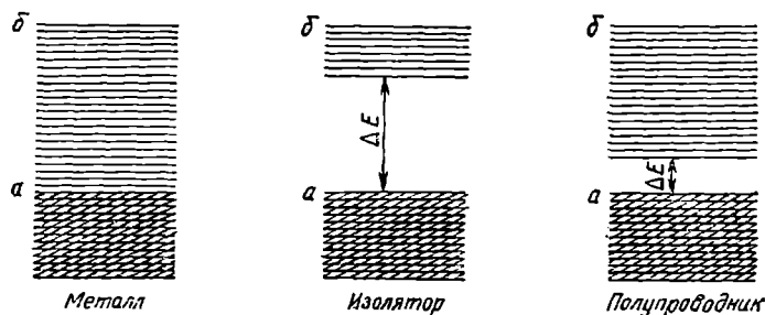
Рис. 138. Схема расположения энергетических зон в металле, изоляторе и полупроводнике a — валентная зона; b — зона проводимости.
