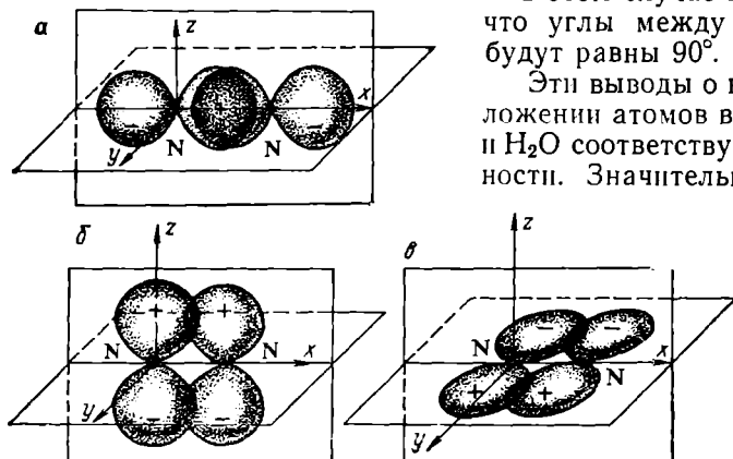
Рис. 35. Схема перекрывания 2p -электронных облаков в молекуле N_2
