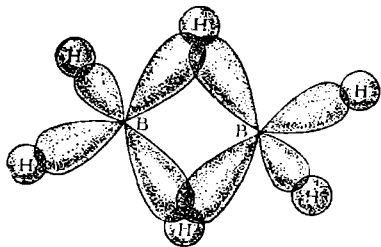
Рис. 164. Перекрытие атомных орбиталей в молекуле диборана.
