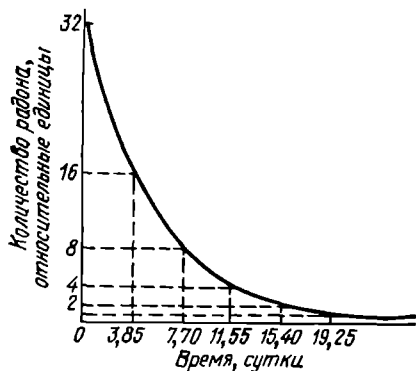
Рис. 25. Зависимость количества нераспавшегося радона от времени.
