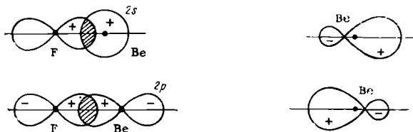
Рис. 38. Схема перекрывания 2p -электронных облаков атомов фтора с 2s - и 2p -электронными облаками атома бериллия (для каждой связи отдельно). Области перекрывания электронных облаков заштрихованы.
