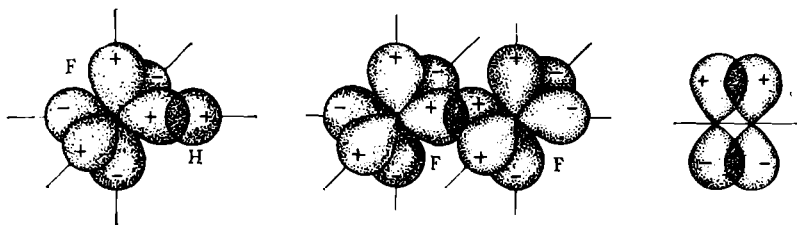
Рис. 32. Схема перекрывания 2p -электронного облака атома фтора и 1s -электронного облака атома водорода при образовании \sigma -связи в молекуле HF: + и — — знаки волновой функции.
