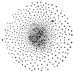
Рис. 5. Электронное облако атома водорода.
