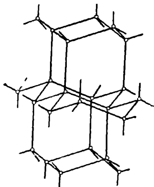
Рис. 72. Схема структуры льда.
