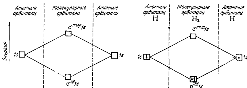
Рис. 45. Энергетическая схема образования МО при взаимодействии 1s -орбиталей двух одинаковых атомов.
