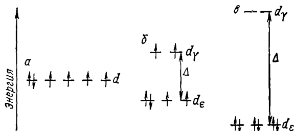
Рис. 162. Распределение электронов иона \text{Co}^{3+} по d -орбиталям: a — в гипотетическом сферическом поле; b — в слабом октаэдрическом поле лигандов (комплекс [\text{CoF}_6]^{3-} ); c — в сильном октаэдрическом поле лигандов (комплекс [\text{Co}(\text{CN})_6]^{3-} ).
