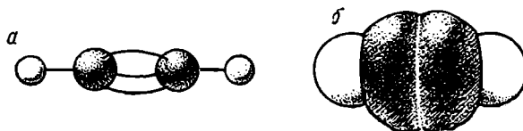
Рис. 129. Модели молекулы ацетилена; а — шариковая; б — сегментовая.
