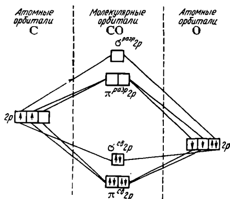
Рис. 53. Энергетическая схема образования молекулы оксида углерода CO.
