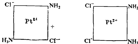
Рис. 156. Пространственное строение изомеров [Pt(NH_3)_2Cl_2] :
