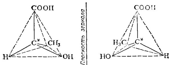
Рис. 130. Тетраэдрические модели молекул зеркальных изомеров молочной кислоты.
