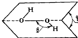
Рис. 106. Схема строения молекулы \text{H}_2\text{O}_2 .
