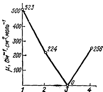
Рис. 155. Изменение молярной электрической проводимости \mu в ряду комплексных соединений платины (IV):
