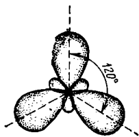
Рис. 41. Взаимное расположение гибридных sp^2 -электронных облаков.
