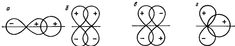
Рис. 28. Схема различных случаев перекрывания электронных облаков:
