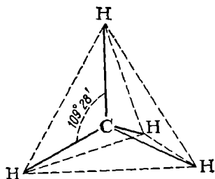
Рис. 120. Тетраэдрическая модель молекулы метана.
