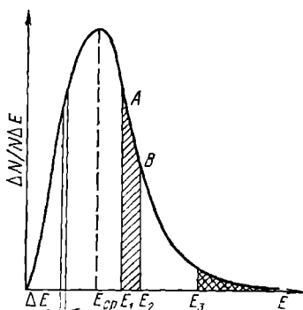
Рис. 63. Распределение молекул газа по кинетической энергии.
