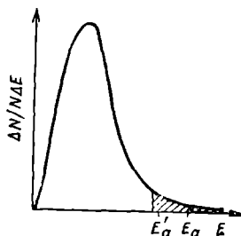
Рис. 67. Влияние катализатора на число активных молекул; E_a — энергия активации без катализатора; E'_a — то же в присутствии катализатора. Площадь заштрихованного участка правее E_a равна доле активных молекул без катализатора, площадь участка правее E'_a — доле активных молекул в присутствии катализатора.
