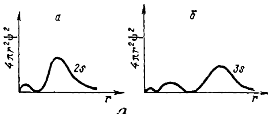
Рис. 13. Схематическое изображение электронного облака 2s-электрона.
