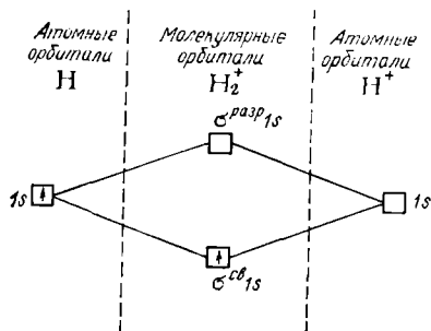
Рис. 47. Энергетическая схема образования молекулярного иона водорода \text{H}_2^+ .
