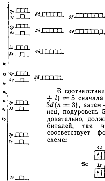
Рис. 22. Последовательность заполнения электронных энергетических подуровней в атоме.
