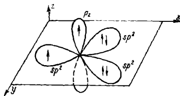
Рис. 111. Схема орбиталей центрального атома кислорода в молекуле озона.
