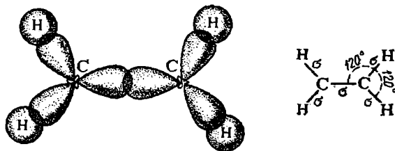
Рис. 125. Схема образования \sigma -связей в молекуле этилена.
