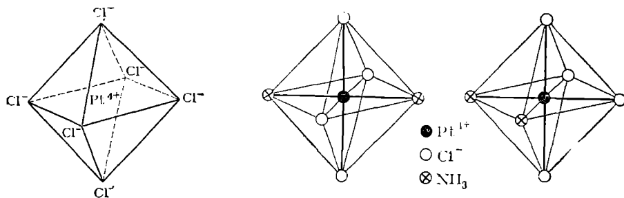
Рис. 157. Пространственное строение комплексного иона [\text{PtCl}_6]^{2-} .
