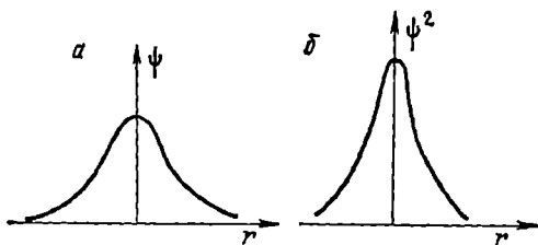
Рис. 9. Графики функций \psi и \psi^2 для 1s -электрона.
