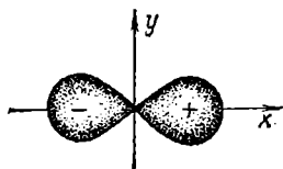
Рис. 17. Схематическое изображение электронного облака 2p-электрона.
