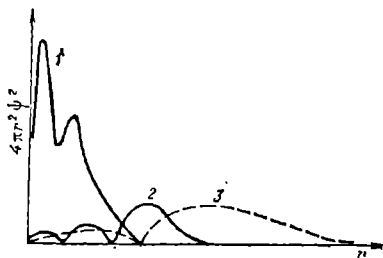
Рис. 21. График радиального распределения вероятности в атоме натрия:
