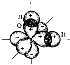
Рис. 36. Схема образования химических связей в молекуле воды.
