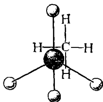
Рис. 122. Шариковая модель молекулы метана.
