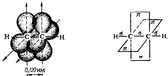
Рис. 127. Схема образования \pi -связей в молекуле ацетилена.
