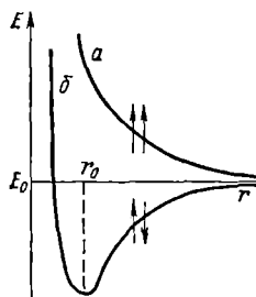
Рис. 26. Энергия системы, состоящей из двух атомов водорода: а — при одинаково направленных спинах электронов; б — при противоположно направленных спинах; E_0 — энергия системы из двух невзаимодействующих атомов водорода; r_0 — расстояние в молекуле водорода.
