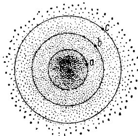
Рис. 7. К понятию об орбитальном моменте количества движения.
