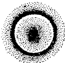
Рис. 13. Схематическое изображение электронного облака 2s-электрона.
