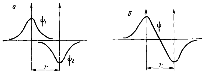
Рис. 44. Схема образования разрыхляющей МО из атомных 1s -орбиталей.
