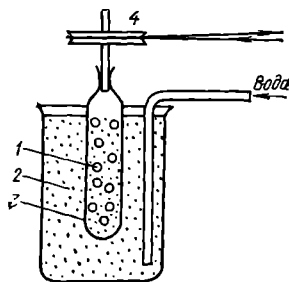
Рис. 91. Схема диализа:
