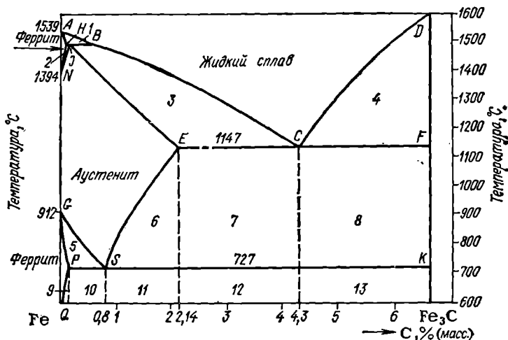
Рис. 168. Диаграмма состояния системы железо—углерод.
