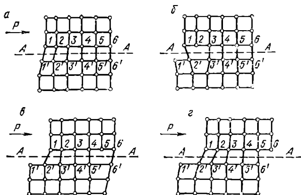
Рис. 142. Дислокационная схема пластического сдвига.
