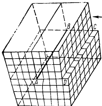
Рис. 62. Схема краевой дислокации.
