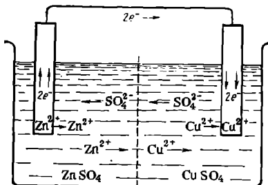
Рис. 82. Схема медно-цинкового гальванического элемента.
