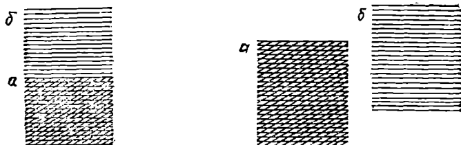
Рис. 136. Схема заполнения электронами энергетических уровней в кристалле щелочного металла:
