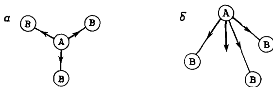
рис. 31. Дипольные моменты отдельных связей в молекулах типа AB_3 :
