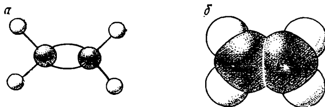
Рис. 128. Модели молекулы этилена; а — шариковая; б — сегментовая.
