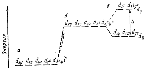
Рис. 160. Схема энергетических уровней d -орбиталей центрального иона:
