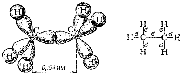
Рис. 124. Схема образования \sigma -связей в молекуле этана.
