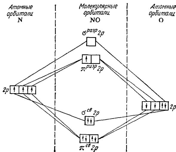
Рис. 116. Энергетическая схема образования молекулы NO.
