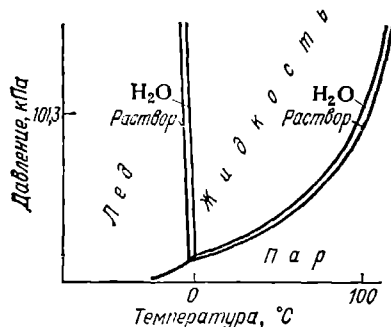
Рис. 78. Диаграмма состояния воды и водного раствора нелетучего вещества.
