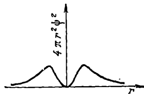
Рис. 16. График радиального распределения вероятности для 2p -электрона.
