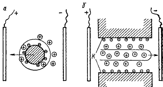
Рис. 101. Схема передвижения коллоидной частицы при электрофорезе (а) и электроосмотическом переносе жидкости через капилляр (б) ( K — внутренняя поверхность капилляра). Поверхности коллоидной частицы и капилляра заряжены отрицательно.
