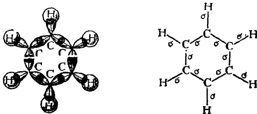
Рис. 131. Схема образования \sigma -связей в молекуле бензола.
