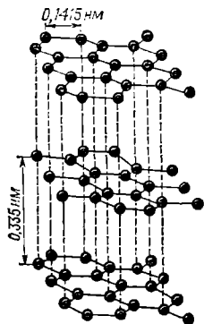
Рис. 118. Структура графита.
