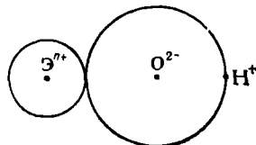
Рис. 108. Ионная схема фрагмента молекулы гидроксида \text{Э}(\text{OH})_n .
