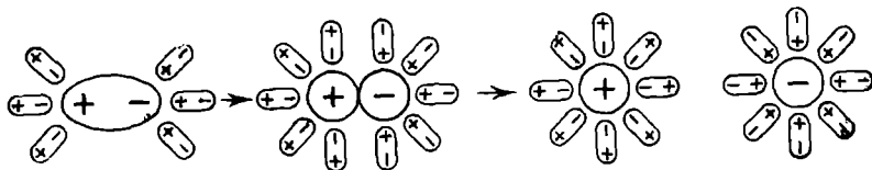
Рис. 81. Схема диссоциации полярных молекул в растворе.
