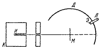
Рис. 2. Схема опыта по рассеянию \alpha -частиц.
