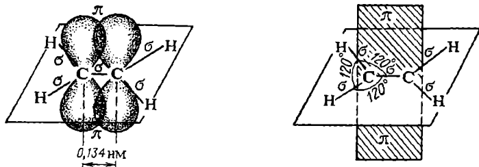
Рис. 126. Схема образования \pi -связи в молекуле этилена.
