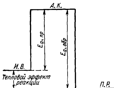
Рис. 65. Энергетическая схема реакции:
