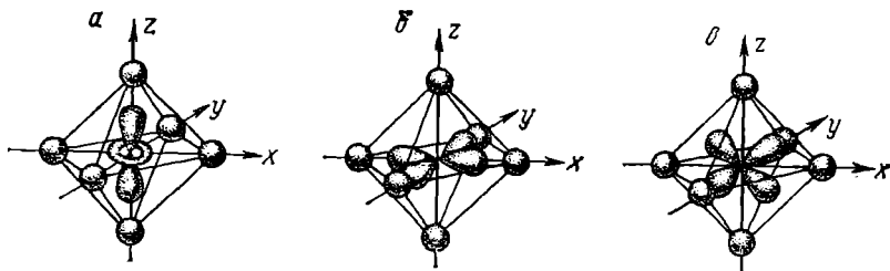
Рис. 161. Орбитали d_{z^2} (а), d_{x^2-y^2} (б) и d_{xz} (в) в октаэдрическом поле лигандов (лиганды условно изображены в виде шариков).
