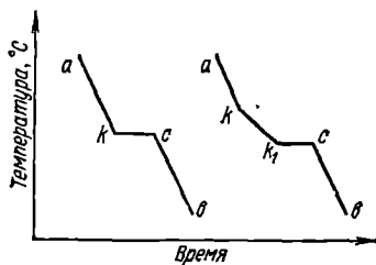
Рис. 145. Кривые охлаждения.
