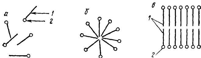
Рис. 80. Растворы мицеллярных коллоидов: молекулярный раствор (а), коллоидные растворы со сферическими (б) и пластинчатыми (в) мицеллами.
