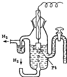
Рис. 84. Водородный электрод.
