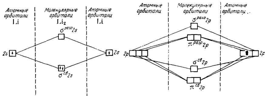
Рис. 49. Энергетическая схема образования молекулы лития \text{Li}_2 .
