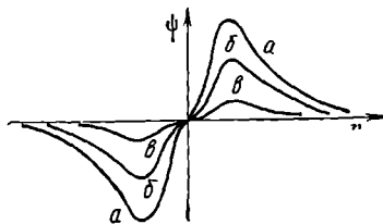
Рис. 15. График волновой функции 2p -электрона.
