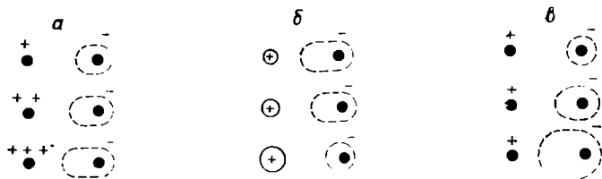
Рис. 55. Схема влияния на поляризацию отрицательных ионов:
