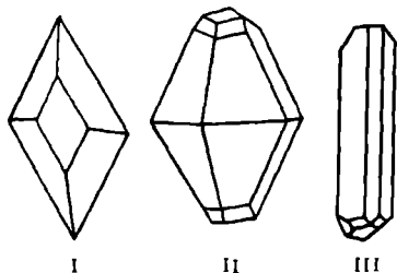
Рис. 112. Кристаллы ромбической серы (I и II).
