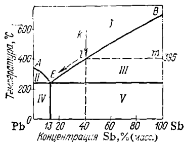
Рис. 147. Диаграмма состояния системы Pb—Sb.
