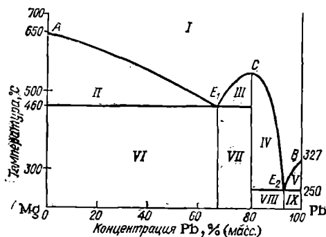
Рис. 152. Диаграмма состояния системы Mg—Pb.
