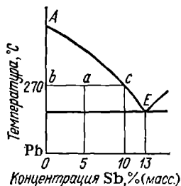
Рис. 149. Часть диаграммы состояния системы Pb—Sb.
