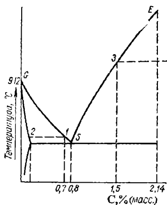
Рис. 169. Часть диаграммы состояния системы железо — углерод.
