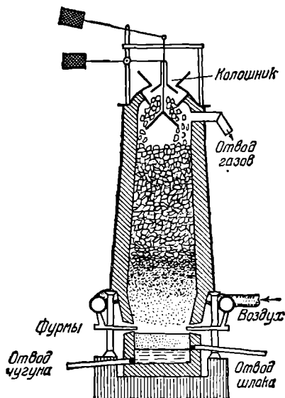
Рис. 171. Схема доменной печи.
