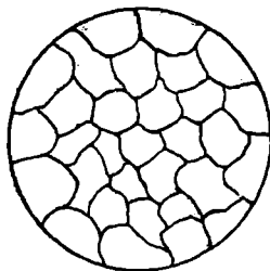
Рис. 143. Микроструктура сплава двух металлов, образующих механическую смесь.
