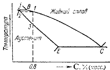
Рис. 169. Часть диаграммы состояния системы железо — углерод.
