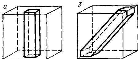
Рис. 60. Бруски, вырезанные из кристаллов каменной соли:
