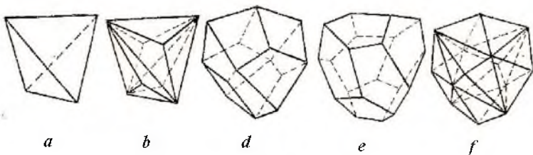
14-rasm. Tetrayerdlar. a) tetrayerdr, b) trigontritetrayerdr, d) tetragontiritetrayerdr, e) pentagontritetrayerdr, f) geksa tetrayerdr.
