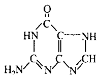
guanin
