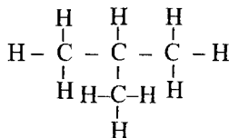
izobutan
