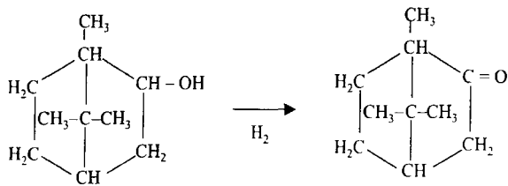
Borneol
