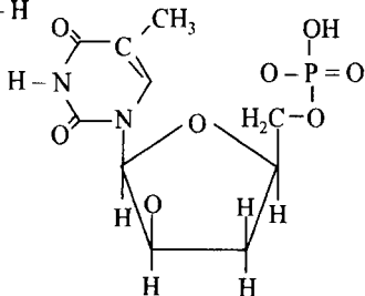
Sitizin qoldig'i
