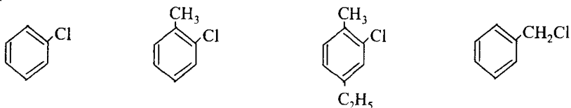
xlорbenzol
