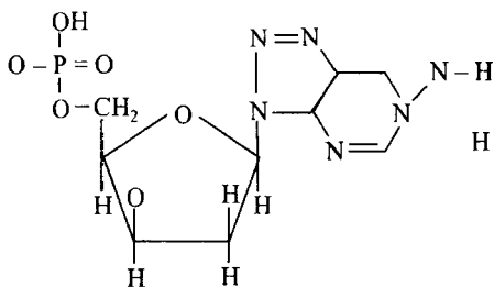
Guanin qoldig'i
