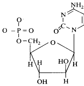
Dezoksitsitin-5'-monofosfat
