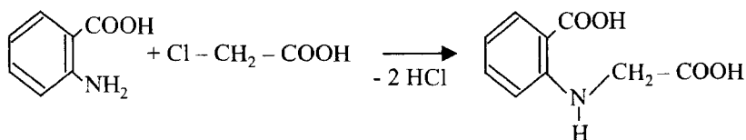
N-(o-karbokifenil)-gliksin
