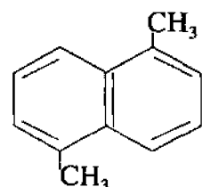
ana- dimetil- naftalin
