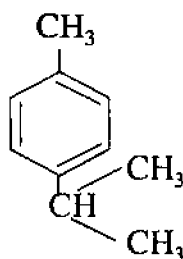
simol, 1-metil - 4- izopropilbenzol
