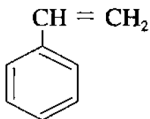
stirol, vinilbenzol, feniletilen
