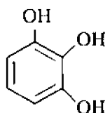
pirogallol (1,2,3-benzentriol, 1,2,3-trigidroksi- benzol )
