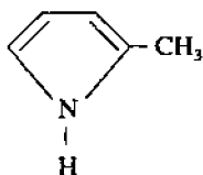
\alpha - metilpirrol yoki 2 - metilpirrol
