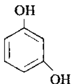
rezorsin (1,3 – benzendiol, 1,3 – digidroksibenzol)
