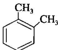
o – ksilol , o-dimetilbenzol, 1,2-dimetilbenzol
