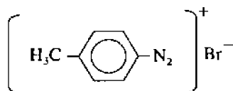
p - tolildiazoniy bromidi
