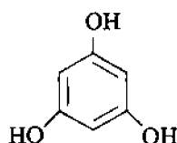
floroglyutsin (benzentriol – 1,3,5; 1,3,5 – trigidroksi - benzol )
