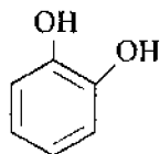
pirokatexin (1,2 – benzendiol, 1,2 – digidroksibenzol)
