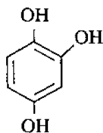
gidroksigidroxinon (1,2,4--benzentriol, 1,2,4- trigidroksi- benzol)
