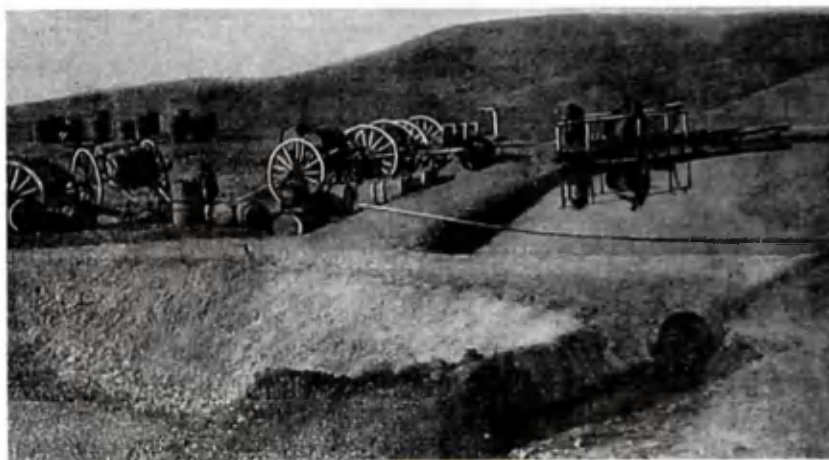
Чимёндаги нефт ҳавзалари.
