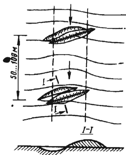
3.2.5-rasm. Suv oqimini tutuvchi zovur.
