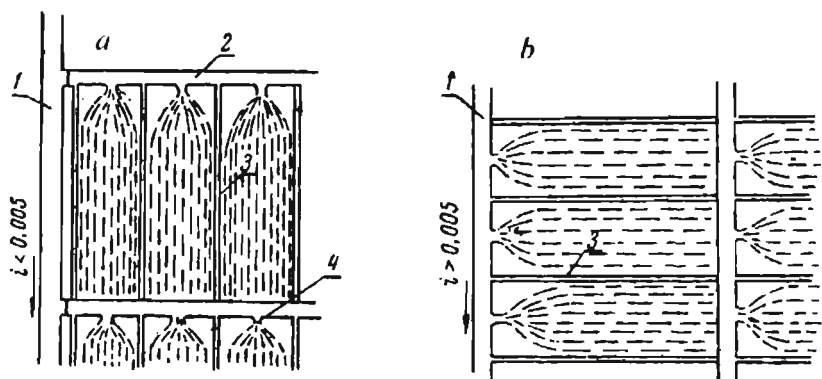
5.1.2-rasm. Yaylov o'tlarini marzalarga bo'lib sug'orish: a —yerning nishabligi 0,005 dan kichik bo'lgan sharoitda; b —yerning nishabligi 0,005 dan katta bo'lgan sharoitda. 1—vaqtinchalik sug'orish tarmog'i; 2—suvni taqsimlash ariqlari; 3—marza; 4—quvur yoki sifon nay.
