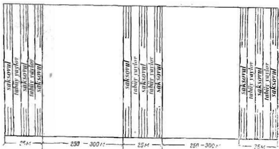
3.2.22-rasm. Polosani bo'laklarga bo'lib shudgorlash va qora saksovil ihotazorini barpo qilish tizimi.
