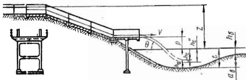
Temir-beton novlar orqali oqizish
