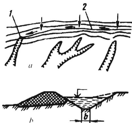
3.2.6-rasm. Suvni oqizib yuboruvchi kanava:
