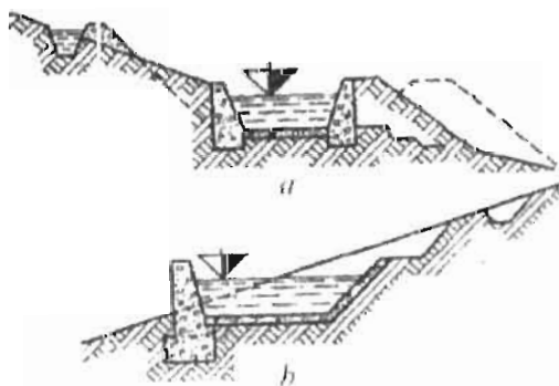
Latoklarni qiyaliklarda joylashtirish tizimi
