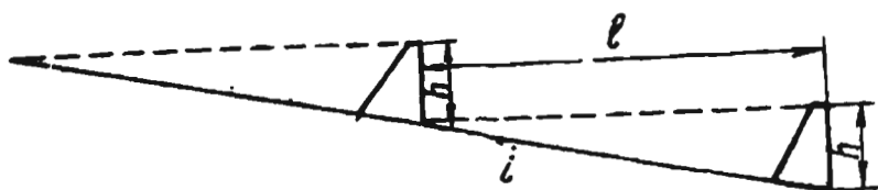
3.2.9-rasm. Jarlik o'zani bo'ylab to'siqlarni joylashtirish tizimi.
