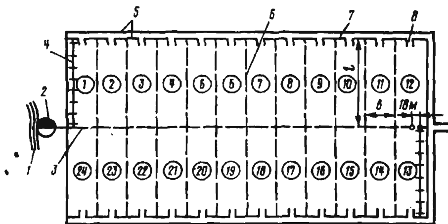
5.1.7-rasm. DKG-801 «Oka» yomg'irlatgich mashinasi gidrantlari va yaylov bo'laklarini joylashtirish tizimi: 1–suv manbasi; 2–nasos stansiyasi; 3–asosiy truboprovod gidrantlari bilan; 4–mashinaning yomg'irlakichlari; 5–doimiy quralar; 6–vaqtinchalik quralar; 7–chorva molini haydash yo'llari; 8–bo'lakka kirish yo'llari; L–bo'lak uzunligi; V–bo'lak kengligi; 1–bo'laklar raqami.
