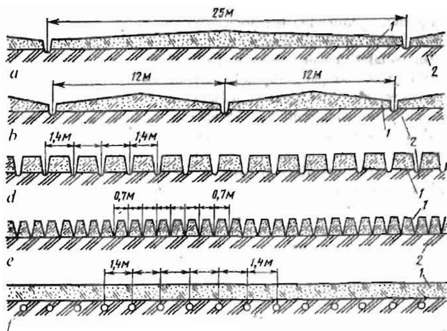
4.1-rasm. Botqoqlanishga moyil yerlarda o'tkaziladigan agromelioratsiya tadbirlari:
