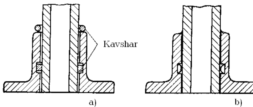
17.2-rasm. Kapillar usulda kavsharlash sxemasi:
