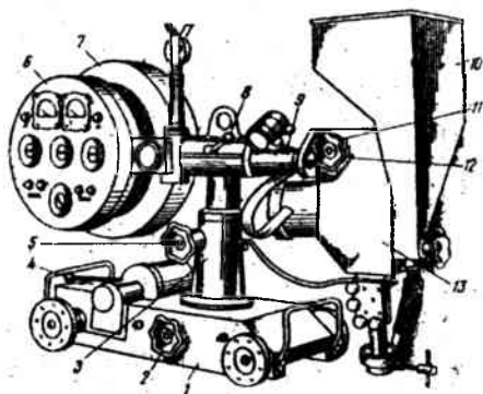
3.3-rasm. Payvandlash traktori:
