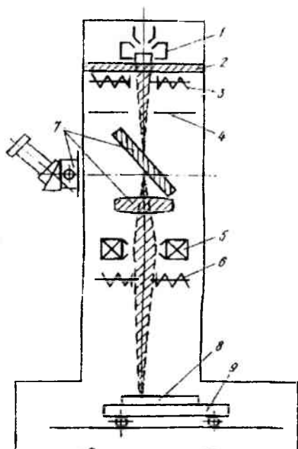
7.4 - rasm. Elektron nurli qurilmaning ko'rinishi:
