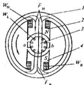
5.10-rasm. Kollektorli payvandlash generatorining (ko'ndalang kesimi) tuzilishi:
