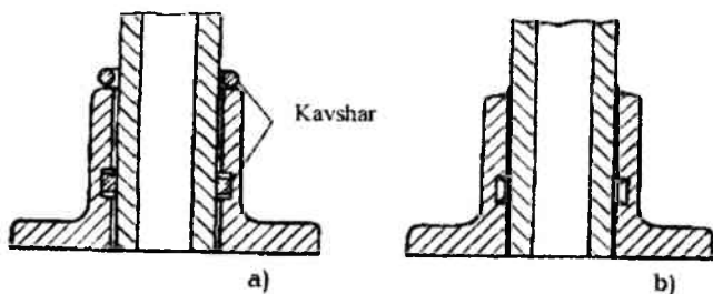
16.2-rasm. Kapillar usulda kavsharlash sxemasi: a – kavsharlashdan oldin; b – kavsharlashdan keyin.
