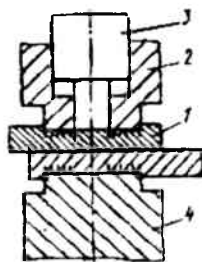
10.3-rasm. Payvandlanayotgan detalni bir tomonli deformatsiyalash bilan sovuq holatda nuqtali payvangdlash chizmasi.
