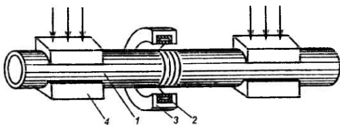
13.2-rasm. Quvurni yuqori chastotali tok bilan payvandlash sxemasi:
