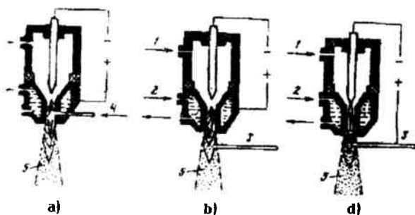
15.4-rasm. Plazmali changlatish sxemasi:
