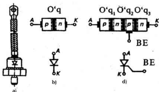
5.4-rasm. Diod va tiristorni qurilmasi va ishlash prinsipi.
