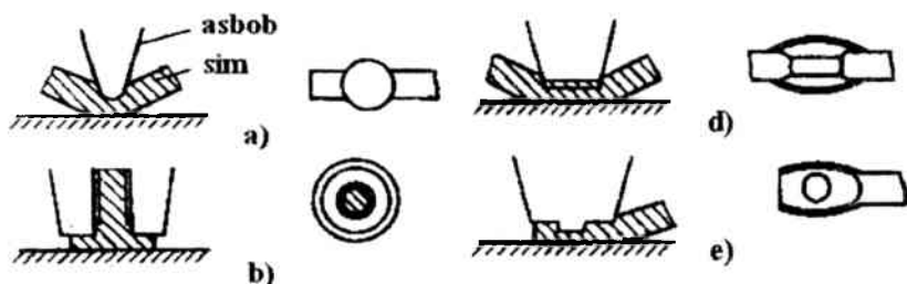
12.3-rasm. Ishlatilayotgan asbob shakli bo'yicha termokompression birikmalarning asosiy turlari:
