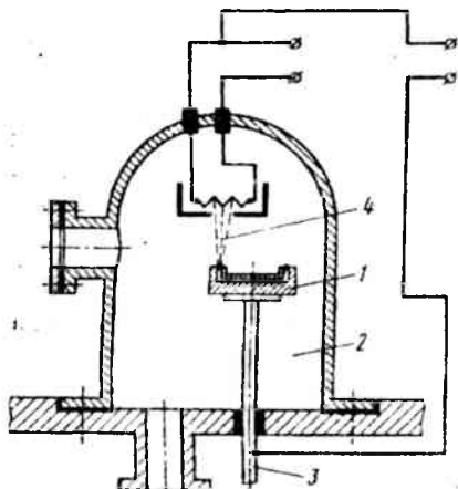
7.1-rasm. Elektron-nurli payvandlash sxemasi:
