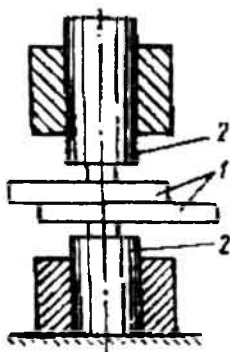
10.1-rasm. Payvandlanayotgan detallarni oldindan qismasdan sovuq holatda nuqtali payvandlash sxemasi:
