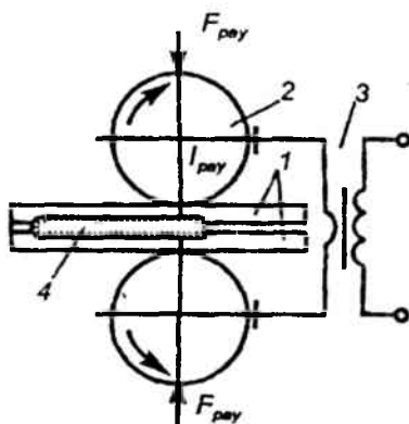
9.2-rasm. Kontaktli choqli payvandlash sxemasi:
