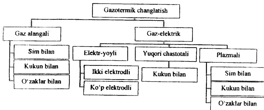
15.1-rasm. Gazotermik changlatish usullarining klassifikatsiyasi.
