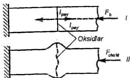
9.5-rasm. Qarshilik bilan uchma-uch payvandlashda birikma hosil bo'lish sxemasi ( F_b – boshlangich kuch; F_{cho'kt} – cho'ktirish kuchi).
