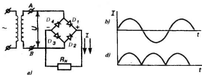
5.5-rasm. Bir fazali ikki yarim davrli ko'priqli to'g'rilash sxemasi: a – qo'shish sxemasi; b – to'g'rilangan tok; d – tashqi zanjirining tok kuchi.
