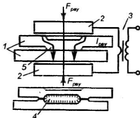
9.3-rasm. Relyefli payvandlash sxemasi:
