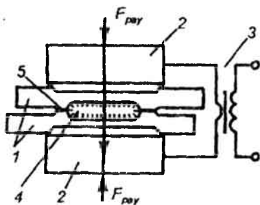
9.1 - rasm. Kontaktli nuqtali payvandlash sxemasi:
