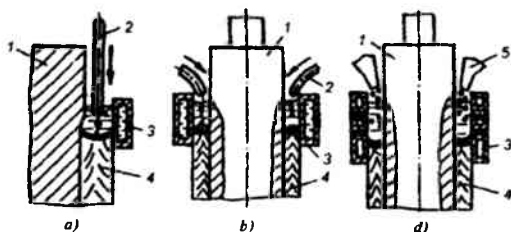
14.4-rasm. Elektr-shlak eritib qoplash chizmasi:
