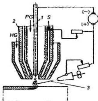
14.7-rasm. Plazma-kukunli eritib qoplash tok uzatuvchi qo'shimcha sim bilan: 1 – elektrod; 2 – soplo; 3 – qo'shimcha tok uzatuvchi sim; PG – plazma tashkil etuvchi gaz; HG – himoya gazi; S – suv.
