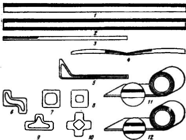
12.5-rasm. Payvand birikmalarning ko'ndalang kesim profillari:
