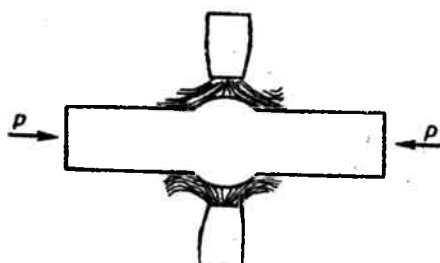
1.4-rasm. Bosim ostida payvandlash chizmasi.
