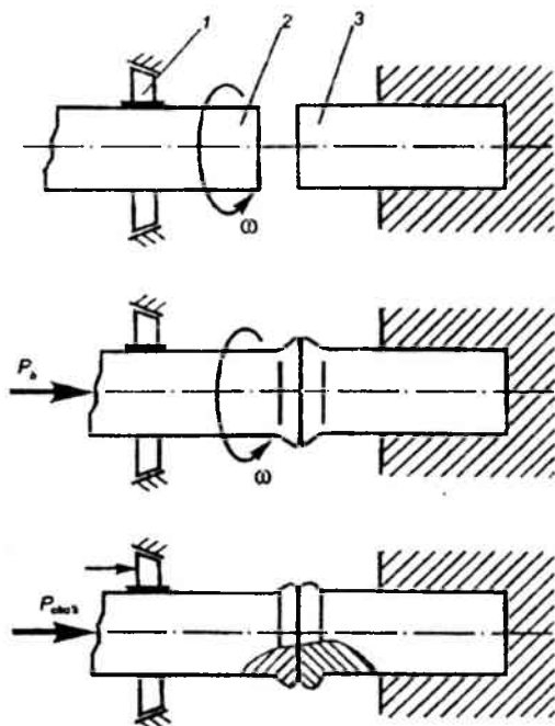
11.2-rasm. Uzluksiz yurg'izib ishqalab payvandlash sxemasi:
