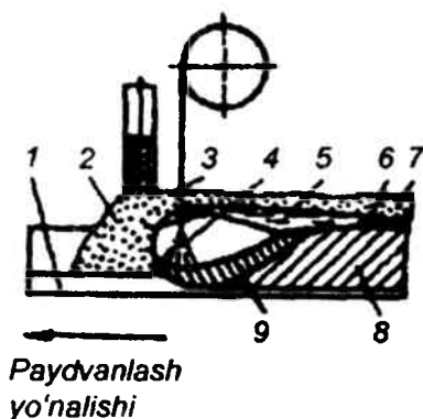
3.1-rasm. Flyus ostida payvandlash chizmasi:
