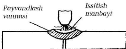
1.3-rasm. Erirtib payvandlash chizmasi.
