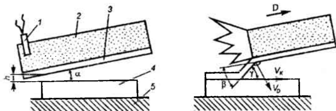
13.1-rasm. Portlatib burchak ostida payvandlash sxemasi:
