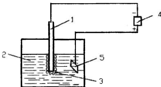
16.6-rasm. Qarshilik bilan kavsharlashning prinsipial sxemasi: 1 – kavsharlanayotgan detallar; 2 – elektrolit; 3 – vodorod buluti; 4 – ta'minlash manbai; 5 – anod.
