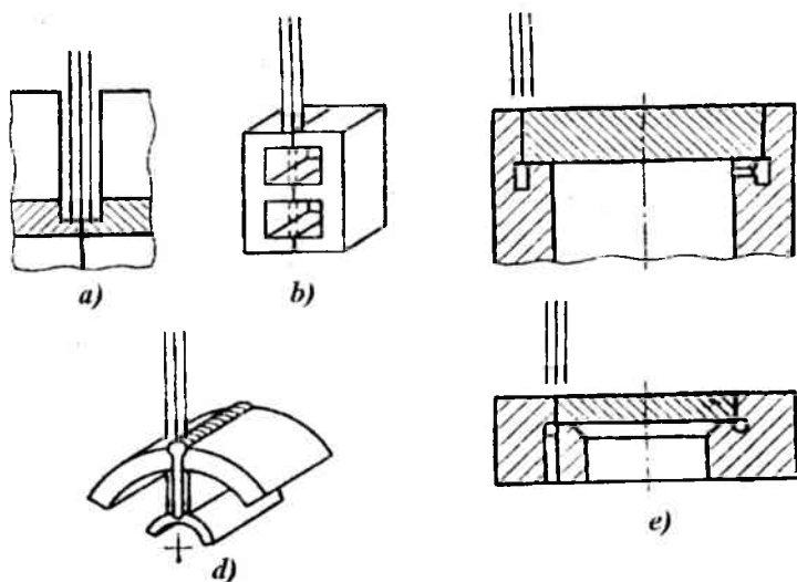
7.3-rasm. Elektron nurli payvandlashda ayrim birikmalarning turlari:
