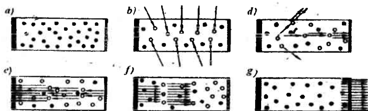
8.2-rasm. Tashqi qo'zg'atish ta'sirida rubin kristalida fotonlar sharrasini ko'chkisimon o'sish sxemasi.
