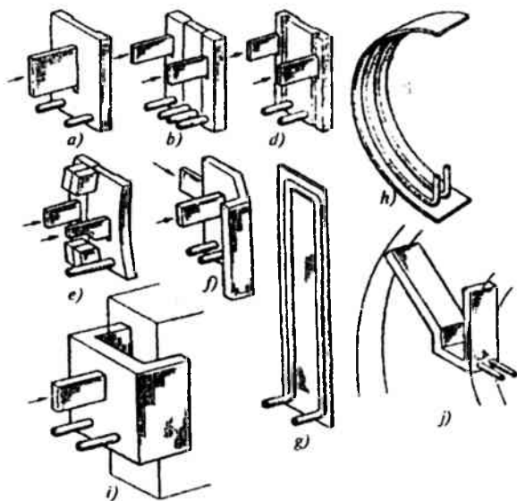
6.3-rasm. Elektr-shlak payvandlash uchun harakatlanuvchi va qo'zg'almas shakllantiruvchi qurilmalar (polzun):
