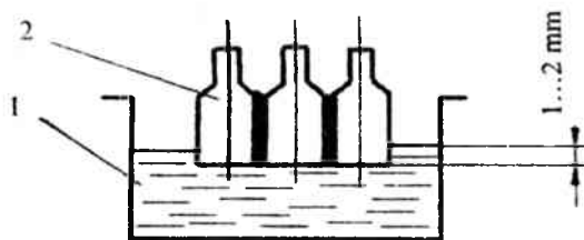
16.7-rasm. Eritilgan kavsharga detalni cho'ktirib kavsharlash sxemasi: 1 – kavshar; 2 – kavsharlanayotgan detallar.
