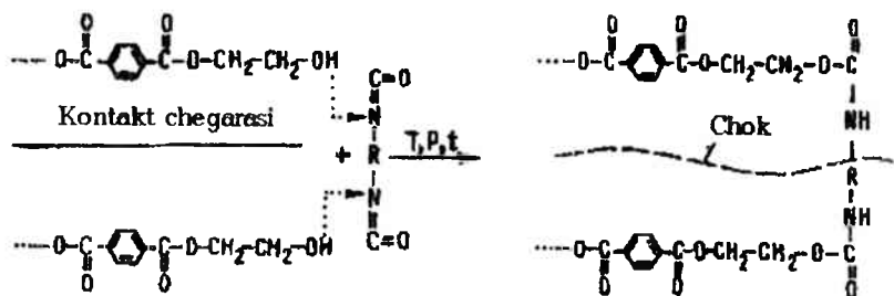
17.6 - rasmi. Diizotsianat yordamida kimyoviy payvandlash mexanizmi.
