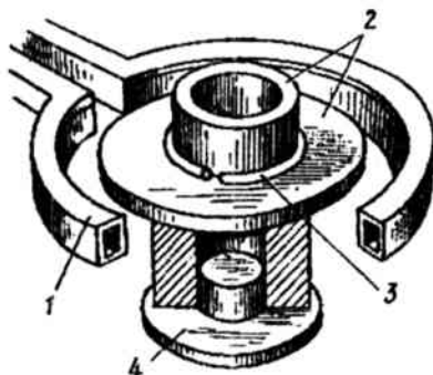
16.5-rasm. Induksion kavsharlashning prinsipial sxemasi: 1 – induktor; 2 – kavsharlanayotgan detallar; 3 – kavshar; 4 – taglik.
