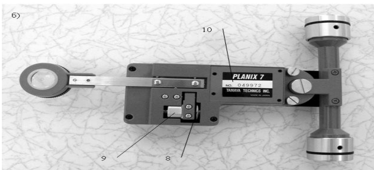
15- rasm. Planix 7 elektron planimetri : a- old tomondan ko‘rinishi; b- orqa tomondan ko‘rinishi; 1- g‘ildirakli mexanizm; 2- raz’yem; 3- ekran; 4- trasser dastasi; 5- rolik; 6- tugmalar; 7- trasser linzasi; 8- g‘ildirak; 9- bosh qism; 10- batareya.
