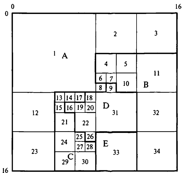
Рис. 11. Разбиение (декомпозиция) исходного участка (см. рис. 10) на квадранты (1—34)
