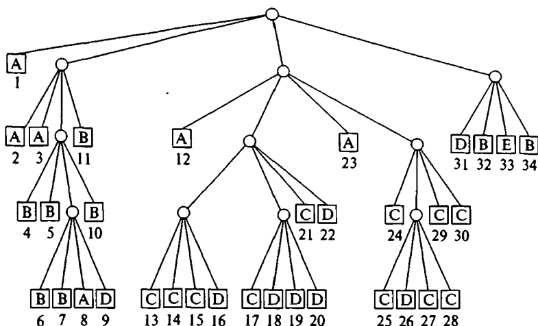
Рис. 12. Итоговое квадродерево как графическая иллюстрация результатов декомпозиции участка на рис. 11
