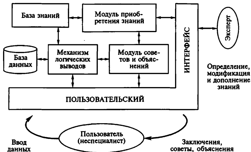
Рис. 43. Базовая структура экспертной системы
