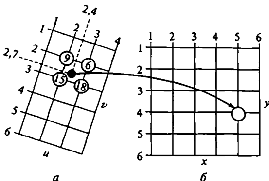
Рис. 38. Присвоение пикселям трансформированного изображения b в сетке (x, y) значений яркости исходного изображения a из сетки (u, v) : черной точкой показано ретрансформированное положение пиксела, отмеченного кружком в эталонной сетке (по [J. R. Jensen, 1996])
