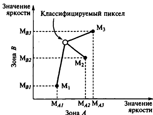
Рис. 40. Метод минимального расстояния
