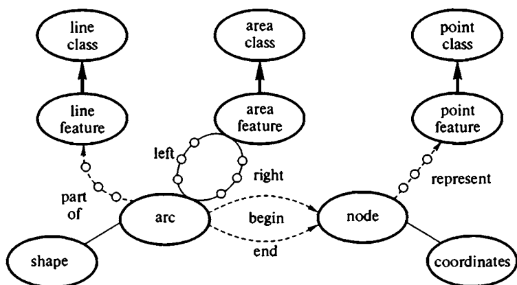
Рис. 14. Одна из возможных векторных моделей данных [М. Molenaar, 1989]. Объекты точечного, линейного и полигонального типов (point, line, area features), дуги (arc), узлы (node), последовательности координат (coordinates), формы (shape), связанные отношениями типа «часть чего-либо» (part of), «левый» и «правый» по отношению к чему-либо (left, right), «начало» и «конец» чего-либо (begin, end)
