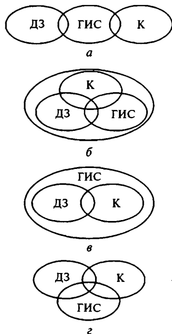
Рис. 3. Модели соотношения картографии (К), дистанционного зондирования (ДЗ) и геоинформационных систем (ГИС):
