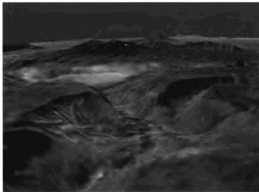
Рис. 12. Анаглифическое отображение ВММ (эффект стереовосприятия местности)
