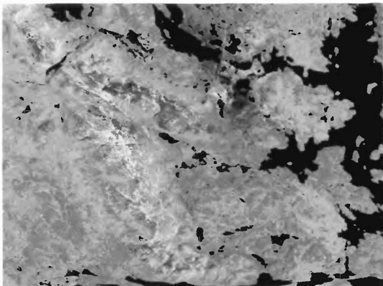
Рис 20. Синтез многозональных снимков, полученных съемочной системой Ландсат MSS 28.06.1978 г. (зоны 3, 2, 1 в диапазонах 0,70 – 0,80; 0,60 – 0,70; 0,50 – 0,60 соответственно), представлена композиция истинного (натурального) цвета
