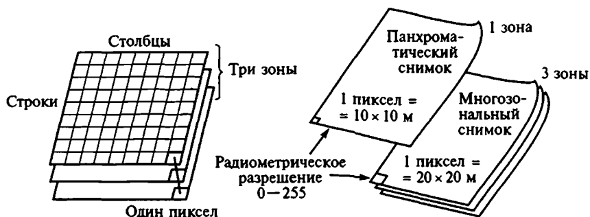
Рис. 32. Пиксел и зоны растрового изображения
