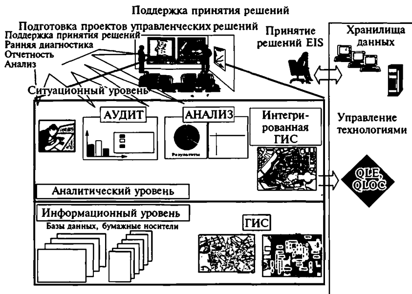
Рис. 48. Схема взаимоотношения информационных уровней в СППР
