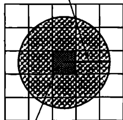
Рис. 37. Область допустимых значений средне-квадратической ошибки
