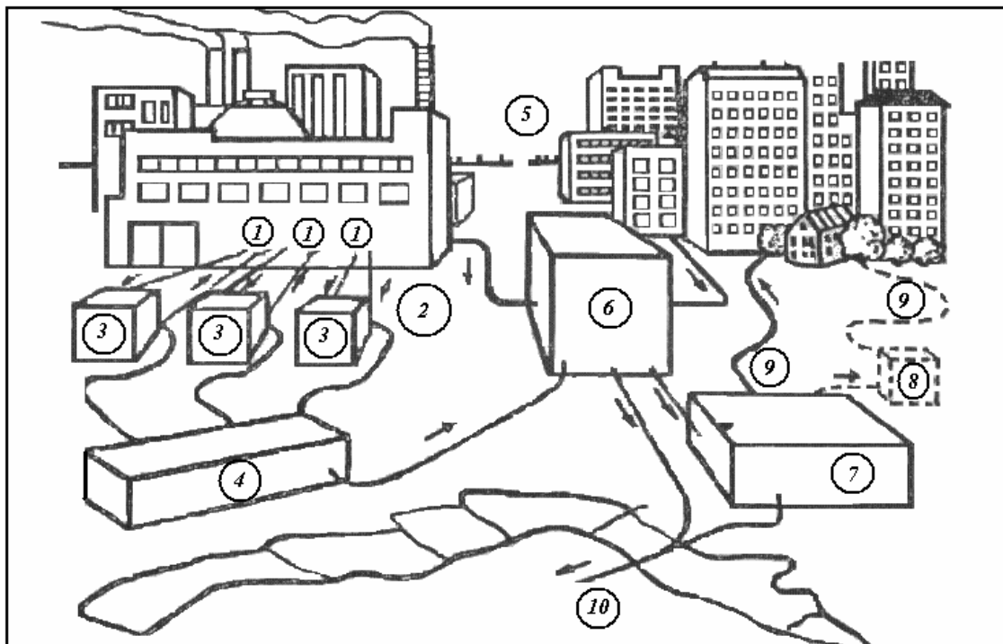
3-Расм. Саноат ва шаҳар айланма сув таъминоти схемаси (Иванов, 1991)
