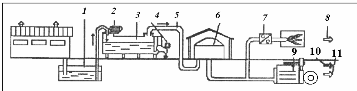
4-расм. Чорвачилик комплекслари оқаваларида мавжуд бўлган компонентларни утилизациялаш схемаси.
