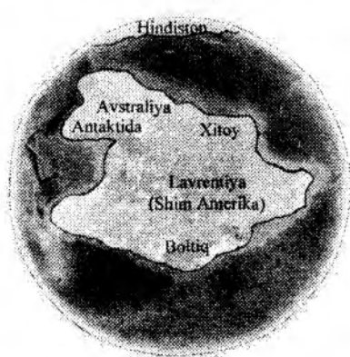
Kenorland supermaterigi
