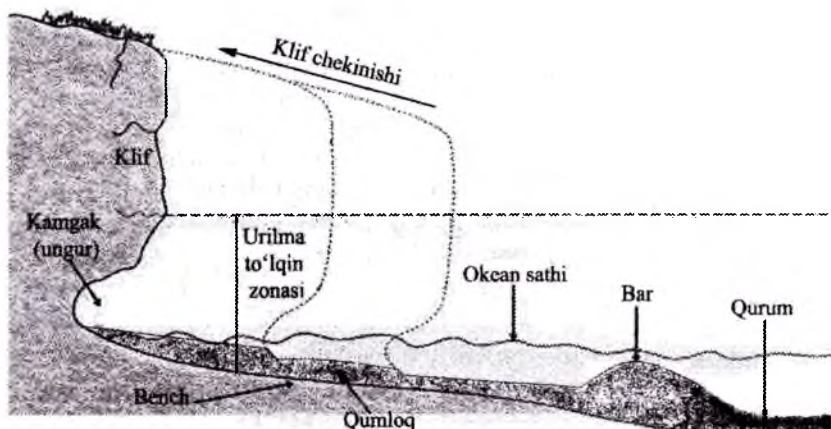
64-rasm. Qirg'oqning morfologik elementlari
