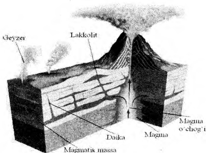
31-rasm. Lakkolitning paydo boʻlishi
