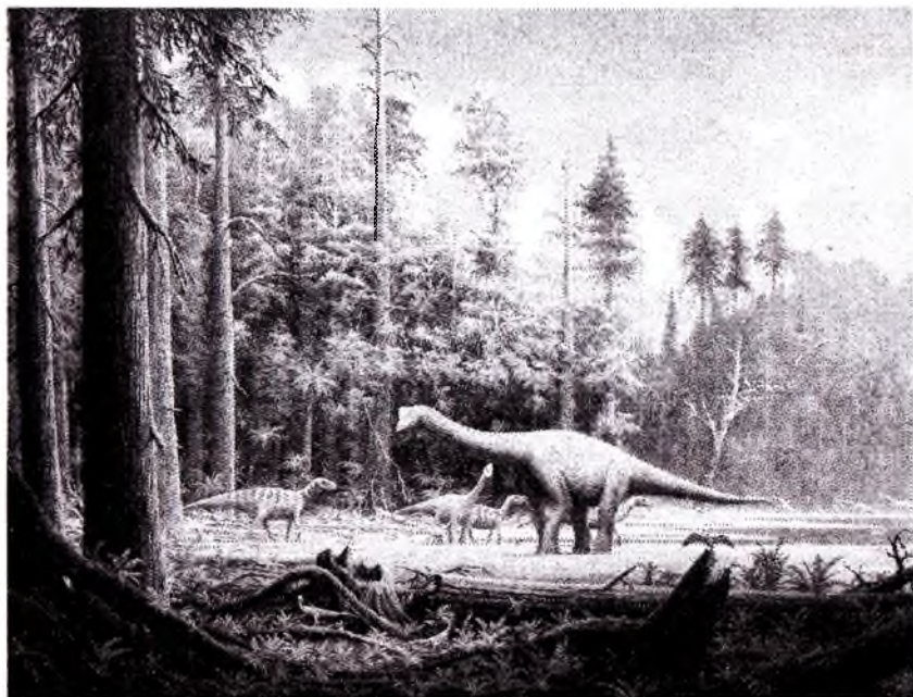
26-rasm. Dinozavrlar mezozoyda Yerdagi umurtqalilar orasida dominant hisoblangan
