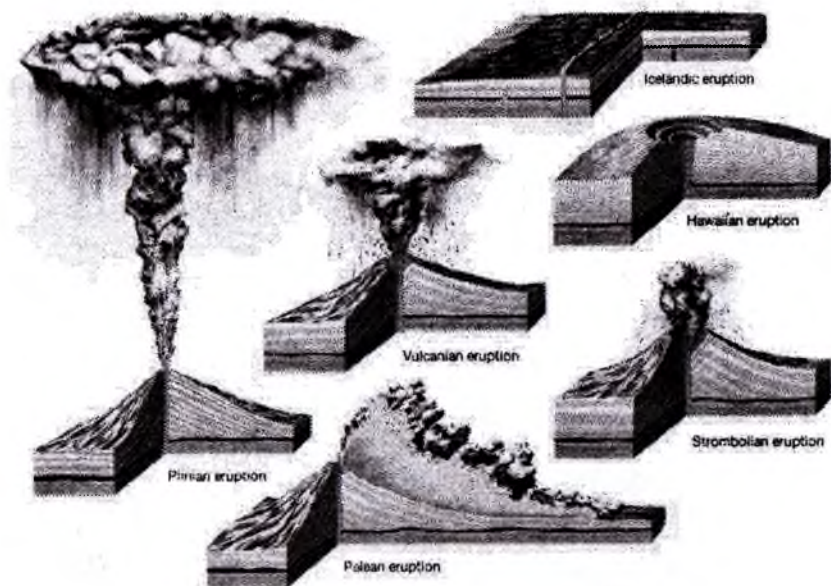
36-rasm. Vulkan turlari
