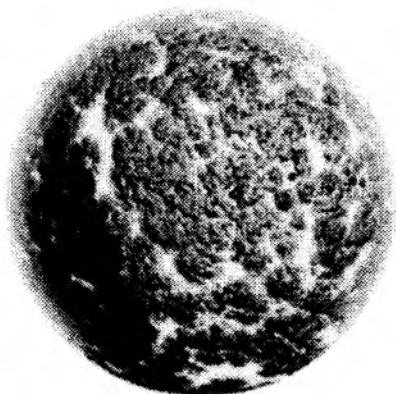
12-rasm. Yerning 4,5 mlrd. yil oldingi holati
