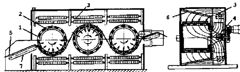
178- rasm. To'r barabanli quritgichning sxemasi:
