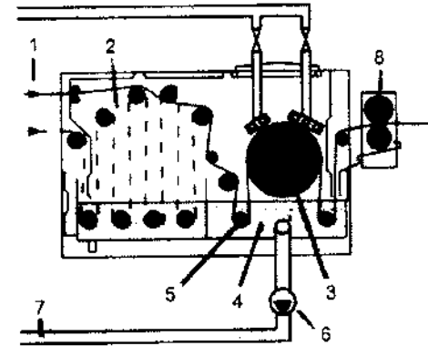
72- ras. "Triko fleks – 2000" yuvish mashinasining sxemasi:
