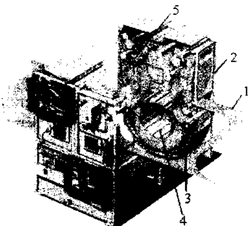
79- rasm. LU – 250 turidagi relaksatsiya kamerasi. 1 – mato; 2 – kamera korpusi; 3 – konveyer; 4 – markaziy baraban; 5 – taxlagich.
