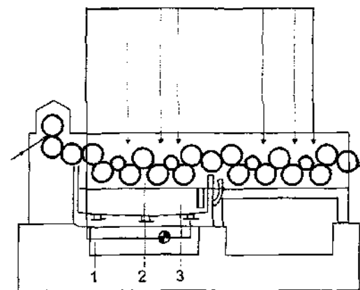
91- rasm. Shimdirish zonasida ishqor eritmasining aylanish sxemasi: 1 – eritmani zonaga uzatish; 2 – shimdirish vannasi; 3 – eritma harorati va konsentratsiyasi regulirovka qilinadigan birlamchi vanna.
