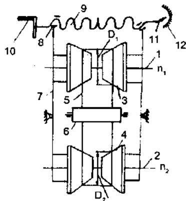
24- rasm. Tezlik variatorining sxemasi:
