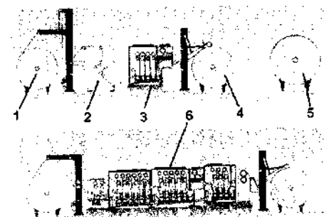
81- rasm. Matoni sovuq holatda oqartirish agregati:
