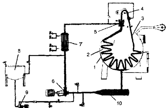
126- rasm. MCD ejektor bo'yash mashinasinig sxemasi:
