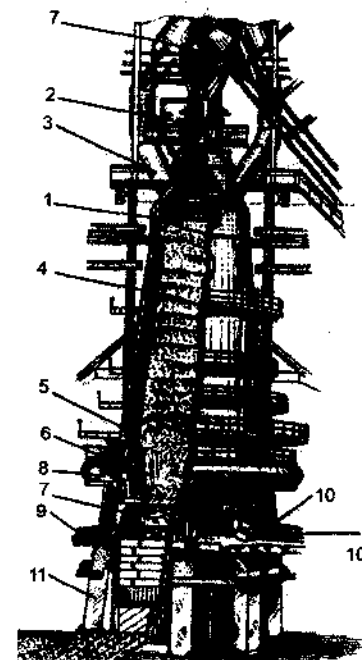
1- rasm. Domna pechining umumiy ko'rinishi:
