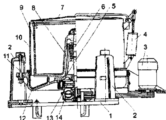
155- rasm. FMK – 1529 K – I markali sentrifuga sxemasi:
