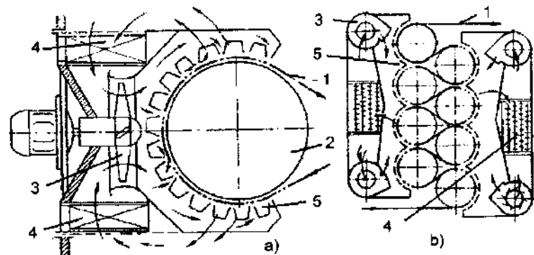
169- rasmda. Quritish barabanida matoni ko'p saploli moslama yordamida puflash sxemasi;
