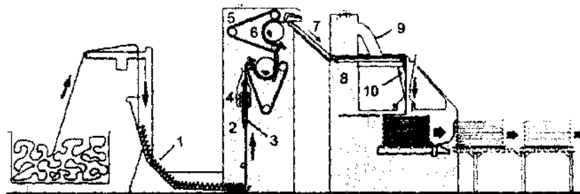
228- rasm. Ikkita kirishtirish mexanizmlil mashina sxemasi:
