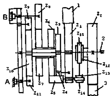
204- rasm. "Kovo" firmasi mashinasining aylana bo'yicha trafleniye qilish uzeli sxemasi:
