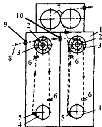
38- rasm. "Tenzitrol" yuvish mashinasining texnologik sxemasi:
