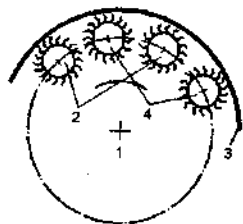
101- rasm. Paxmoqlash va qarshi paxmoqlash vallari va matoning harakatsiz holatida mashina ishchi organlarining o'zaro ta'siri:
