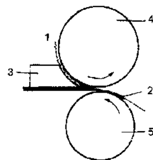
224- rasm. "Monforts" firmasi mato kirishtirish mashinasining sxemasi: 1 – kiritilayotgan mato; 2 – siqilgan mato; 3 – tayanch plita; 4 – yuqoridagi silindr; 5 – pastki silindr.
