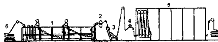
98- rasm. Matoni karbonlash agregati:
