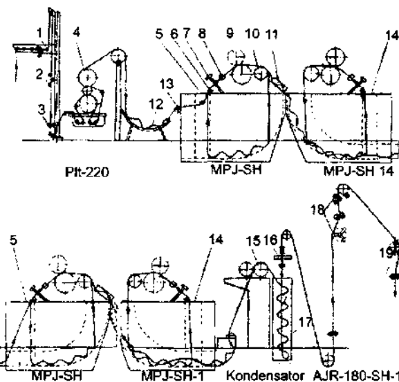
94- rasm. LPJ – 1 – Sh agregatining texnologik sxemasi:
