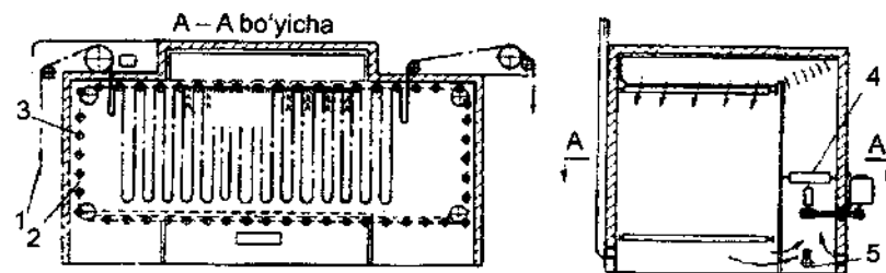
172- rasm. Mato sirtmog'ini osilgan holatda quritish mashinasi sxemasi:
