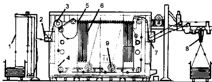
219- rasm. Bug'lash kamerasining sxemasi:
