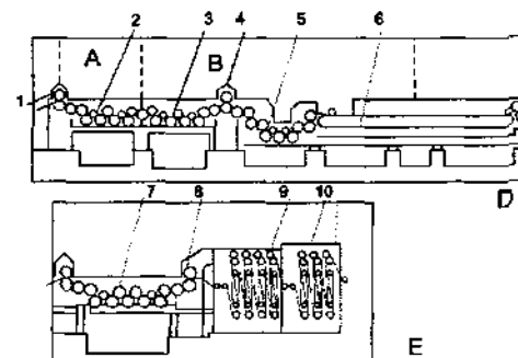
89- rasm. Yengil va o'rta og'irlikdagi matolarni merserlash agregatining texnologik sxemasi:
