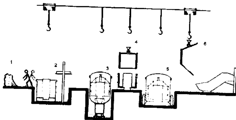
123- rasm. Tola bo'yash va quritish agregatida tolani transportirlash sxemasi: 1 – xomashyo; 2 – tolani bo'shatish va tutqich silindriga yuklash; 3 – bo'yash; 4 – tutqichdan tola solingan silindrga olish; 5 – namlikni kamaytirish; 6 – silindrga toladan bo'shatish.
