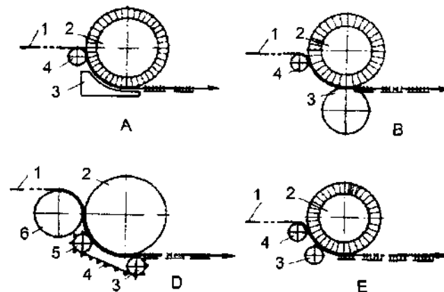
185- rasm. Mato chetini ignalarga sanchish mexanizmlar sxemalari:
