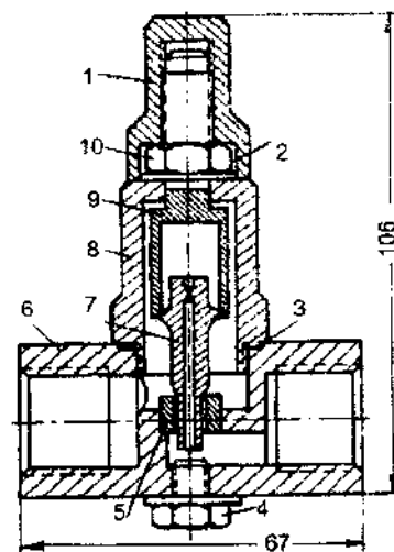
167- rasm. Kichik o'lchamli kondensat chiqaruvchi:
