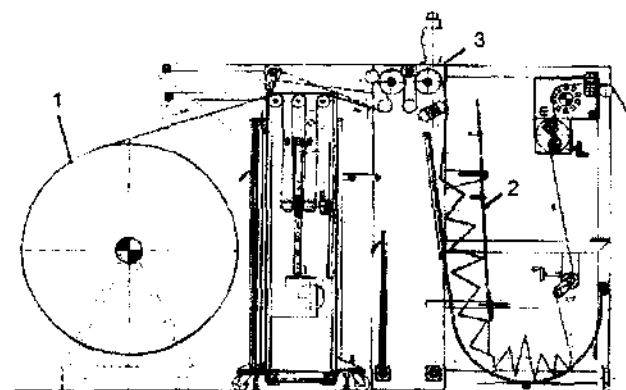
21- rasm. Rolikdan matoni yoyib olish mexanizmi:
