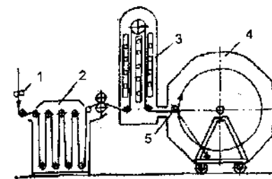
80- rasm. "Pedrol" usulida mato oqartirish agregati:
