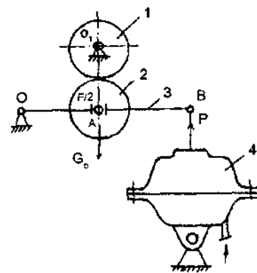
16- rasm. Tarelkasimon membranali pnevmomexanizmlar siqish mexanizmi:
