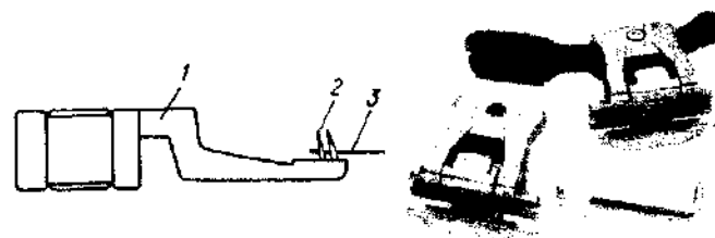
188- rasm. Ignali klupp sxemasi va uning fotografiyasi: 1 – gardish; 2 – igna; 3 – mato.
