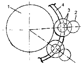
205- rasm. "Mater-Plat" firmasi mashinasi shesternyalar blokining mahkamlanish sxemasi:
