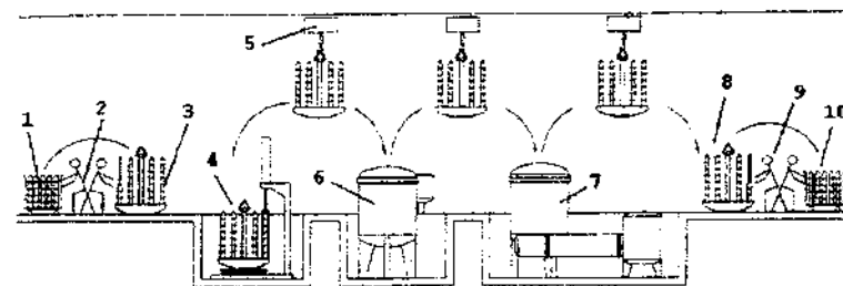
122- rasmda Bo'yash va quritish apparatlaridan iborat agregatda yarim mahsulotlarni transportirlash:
