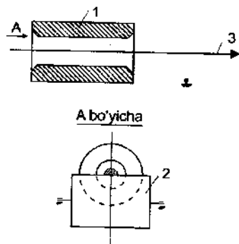
3- rasm. Mato jgutini yo'naltiruvchi halqa: 1 – halqa; 2 – rolik; 3 – mato.
