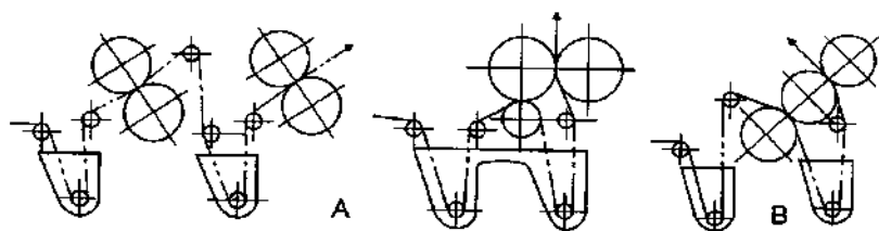
12- rasm. Siqish vallarini fazoda joylashish sxemalari:
