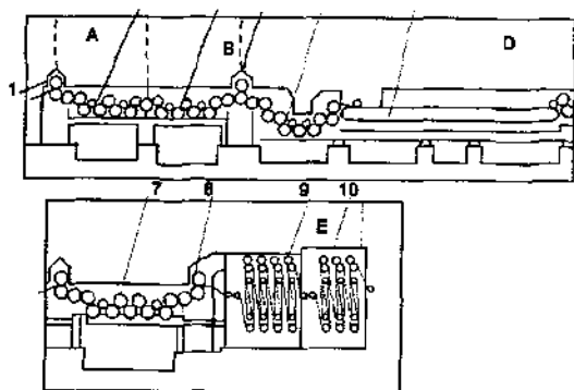
90- rasm. Og'ir matolarni merserlash agregatining texnologik sxemasi:
