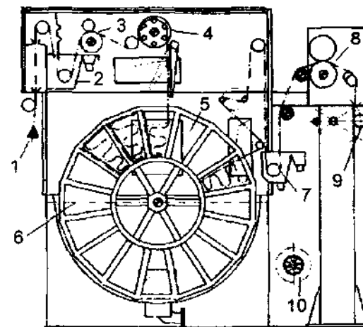
49- rasm. "Star-trans" bug'lash-qaynatish kamerasining texnologik sxemasi:
