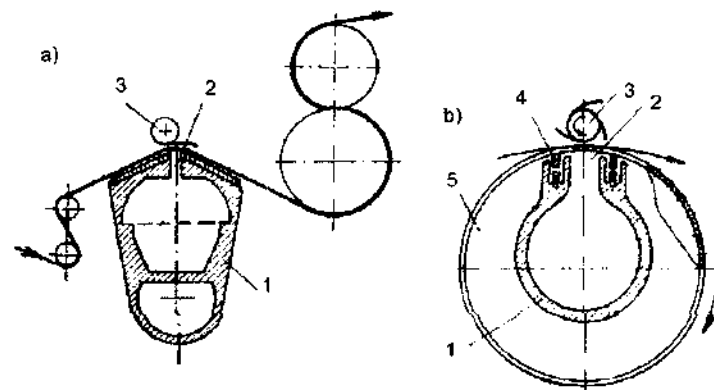
157- rasm. Vakuum so'rish jihozi:
