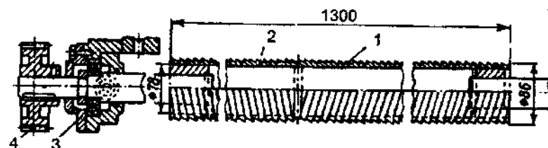
8-rasm. Vintli mato yuzasini rostlovchi sxemasi:
