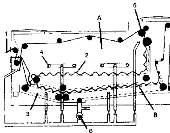
45- rasm. “Ramish Kleynevefers” firmasining bug‘lash-qaynatish kamerasi: A – bug‘lash zonasi; B – eritmada ishlov berish zonasi; 1 – mato; 2 – yuqoridagi konveyer; 3 – pastdagi konveyer; 4 – purkagichlar; 5 – tortuvchi vallar; 6 – nasos.
