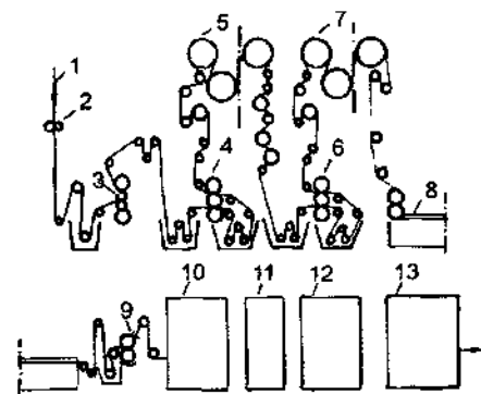
85- rasm. Zanjirli merseqlash agregatining texnologik sxemasi:
