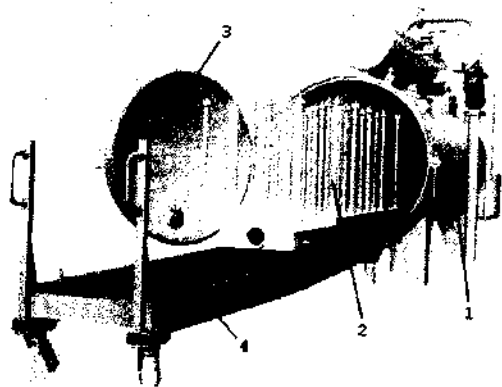
118- rasm. Ispaniyaning "Atus" firmasi universal bo'yash agregati: 1 – avtoklav; 2 – mahsulot tutqich; 3 – avtoklav qopqog'i; 4 – aravacha.
