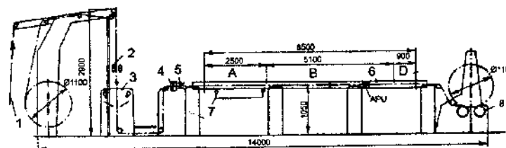
114- rasm. Tarkibida SHS – 120 mashinasi bo'lgan agregatning texnologik sxemasi;
