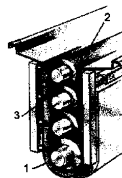
10- rasm. Yuvish vannasiga o‘rnatilgan yo‘naltiruvchi vallar:
