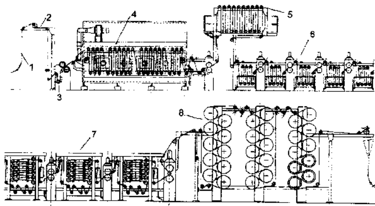
145- rasmda "Sando" firmasinig "Ped-Steam" bo'yash usulida uzluksiz ishlovchi bo'yash agregati:
