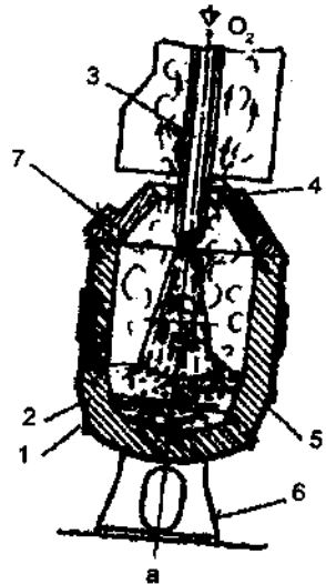
2- rasm. Kislorod konvertorining tuzilishi va ishlash sxemasi:
