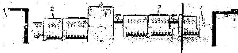
78- rasm. Tarkibida LU turidagi relaksatsiya kamerasi bor yuvish agregati: 1 – mato; 2 – yuvish vannasi; 3 – LU turidagi relaksatsiya kamerasi; 4 – siqish vallari.
