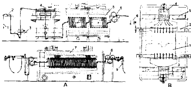
148- rasm. "Sando" firmasining Termozol bo'yash usulida uzluksiz ishlovchi bo'yash agregati
