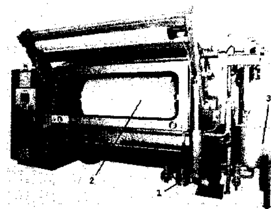
138- rasm. "Mezzera" firmasi jiggerlarining tashqi ko'rinishi: 1 – gardish; 2 – mato o'ralgan rolik; 3 – eritma tayyorlash baki.
