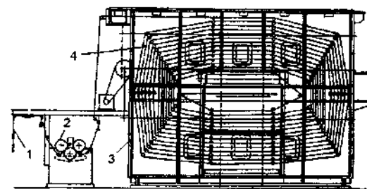
217-rasm. "Kristovitsa" sistemasidagi zrelnik sxemasi:
