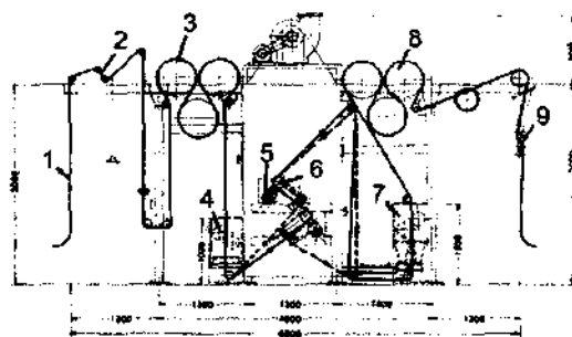
30- rasmda "Sando" firmasi gazli kuydirish agregatining texnologik sxemasi:
