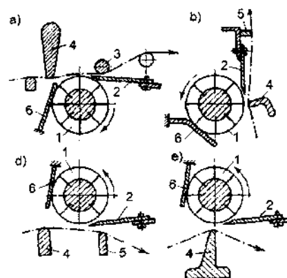
107- rasm. Qirqish apparatlarining sxemalari:
