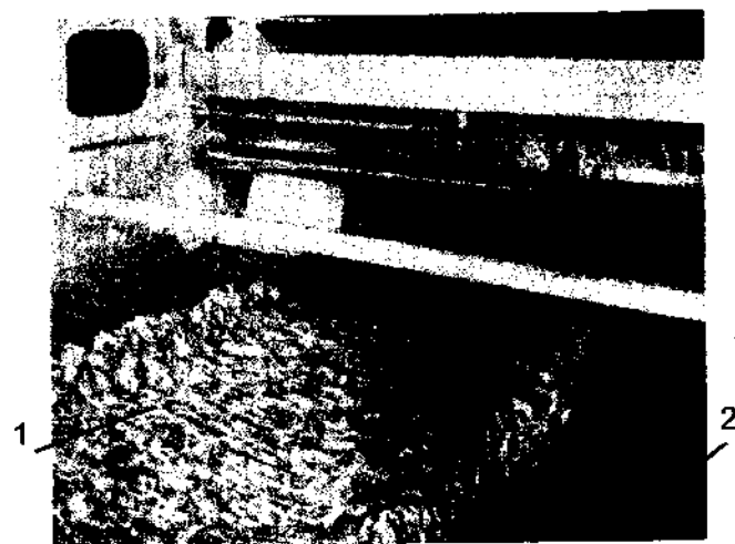
47- rasm. Kamera konveyeri roliklari ustidagi mato taxlami: 1 – mato yoki trikotaj polotnosi taxlami; 2 – konveyer roligi.
