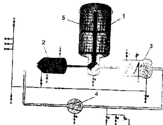
159- rasm. "Tiss" firmasi quritgichining sxemasi;
