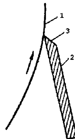
196- rasm. Raklyaning gul bosish vali yuzasiga nisbatan joylashishi;
