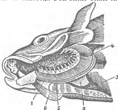
5-rasm. Baliqning jabra apparati: 1 – birinchi jabra yoyi; 2 – yurak; 3 – jigarning bir qismi; 4 – jabra yaproqlari; 5 – jabra tichinkalari; 6 – jabra nurlari.
