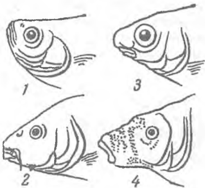
8-rasm. Baliqlarning og'iz tiplari: 1 — yuqoriga qaratilgan og'iz; 2 — oxir- gi og'iz; 3 — pastga qaratilgan og'iz; 4 — oldinga bo'rtib turuvchi og'iz.
