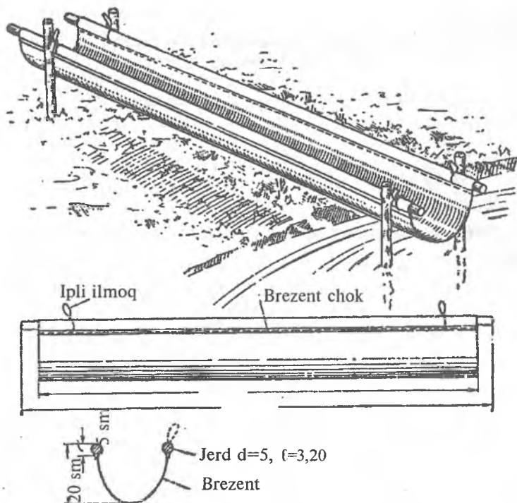
65-rasm. Tirik baliq (segoletka, molod)larni avtosisternadan suvga qo'yish uchun mo'ljallangan brezent-nova va uning sxemasi
