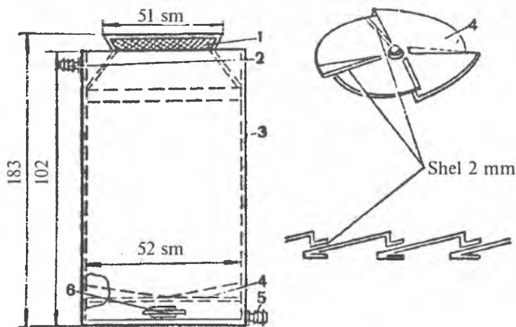
28-rasm. G.I. Savin va N.E. Arxipovlar tomonidan yaratilgan uvildiriq inkubatsiyasi uchun apparat:
