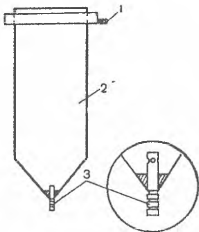
25-rasm. O'simlikxo'r baliqlar uvildiriqlarning inkubatsiyasi uchun qo'llaniladigan VNIIPRX apparati 1 – suv bo'shatiladigan moslama; 2 – inkubatsion silindr; 3 – suv kradigan moslama.
