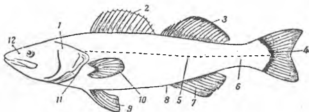
2-rasm. Baliqning umumiy ko'rinishi (sudak): 1. Jabra qopqog'i. 2. Orqa suzgichi — shoxlanmagan nurlar. 3. Orqa suzgichi — shoxlangan nurlar.
