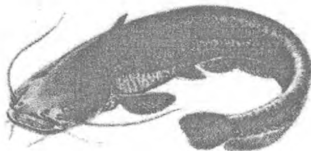
52-rasm. Oddiy laqqaning umumiy ko'rinishi
