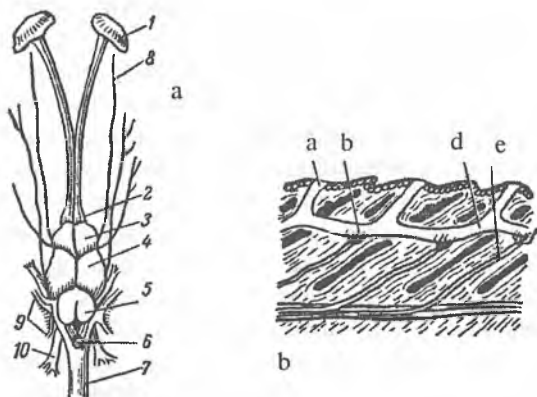
10-rasm. a — baliqning bosh miyasi (zog'ora), b — yon chiziq a'zosi. 1 — hidlov kapsulasi; 2 — hidlov bo'lagi; 3 — oldingi miya; 4 — o'rta miya; 5 — miya-cha; 6 — uzunchoq miya; 7 — orqa miya; 8,9,10 — bosh miya nervlari: a) yon chiziq a'zosining teshiklari; b) sezuvchi hujayralar; d) ko'ndalang kanal; e) nerv tolalari.
