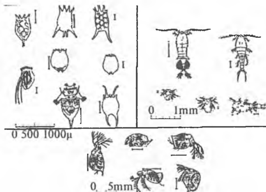
56-rasm. Kolovratkalar, kladatseralar va kapepodalarning xilma-xil turlari
