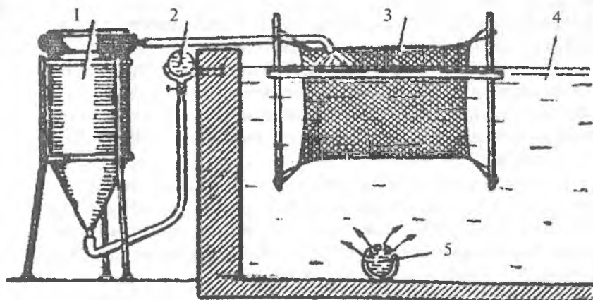
29-rasm. VNIIPRX apparati o'simlikxo'r baliqlar inkubatsiyasi va saqlash uchun maxsus moslama sxemasi:
