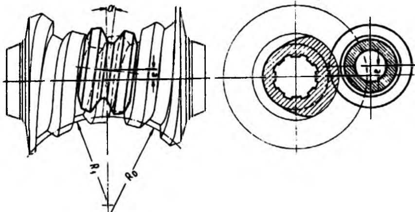
5.10-rasm. Globoidli chervyak va rolik.
