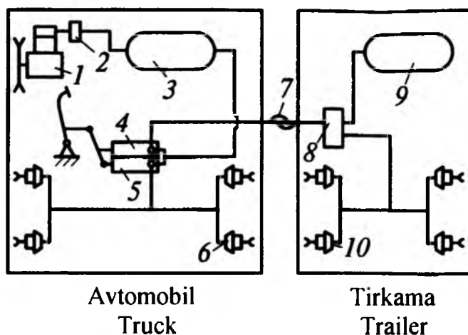
6.15-rasm. Avtopoyezdlarning bir uzatmalı pnevmatik tormoz yuritmasi sxemasi:
