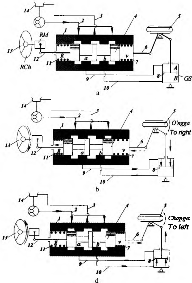
5.6-rasm. Rul kuchaytirgichning ishlash sxemasi. a—to'g'ri chiziqli harakat holati; b—o'ngga burilish jarayoni; d—chapga burilish jarayoni. RM—rul mexanizmi; GS—gidrosilindr; RCh—rul chambaragi.
