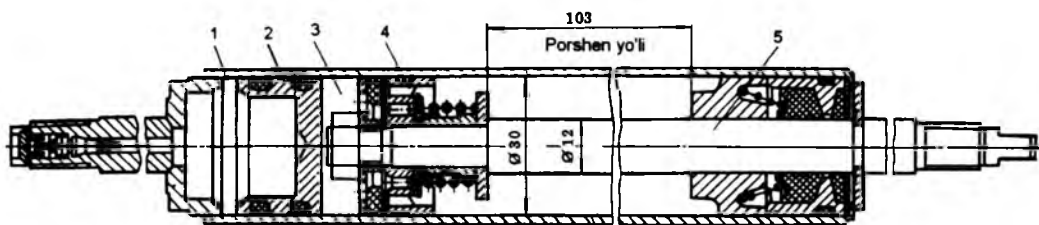
4.7-rasm. Bir trubali teleskopik amortizator:
