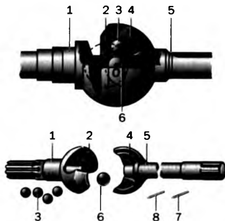
3.15-rasm. Burchak tezliklari teng sharchali kardan sharniri: 1 va 5—kardan yarim vallari; 2 va 4—ariqchalar; 3—to'rtta moment uzatuvchi sharchalar; 6—vallarni markazlashtiruvchi sharcha; 7 va 8—shipilkalar.
