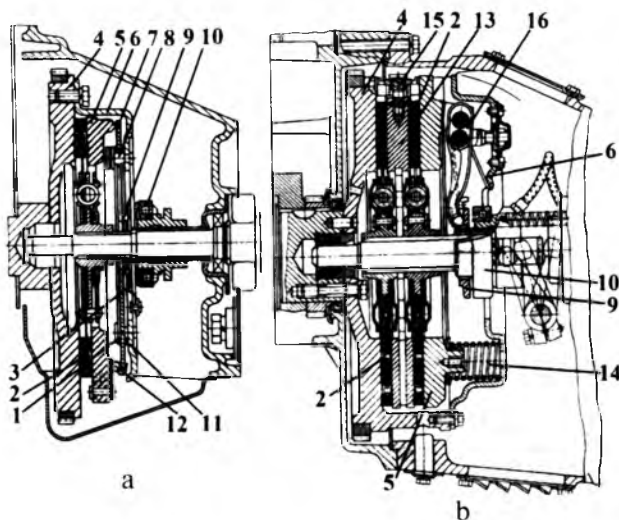
3.4-rasm. Bir (a) va ikki (b) diskli ilashish muftasi.
