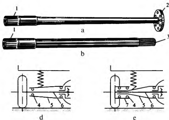
3.23-rasm: Yarim o'qlar: a—flanesli; b—flanesiz; d—yarim yuksizlantirilgan; e—to'la yuksizlantirilgan; 1, 3—shlisli uchlari; 2—flanes; 4—podshipnik; 5—balka; 6—yarim o'q; 7—stupitsa.
