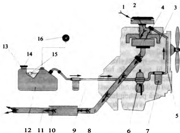
2.10-rasm. Karbyuratorli dvigatel ta'minlash tizimining sxemasi.
