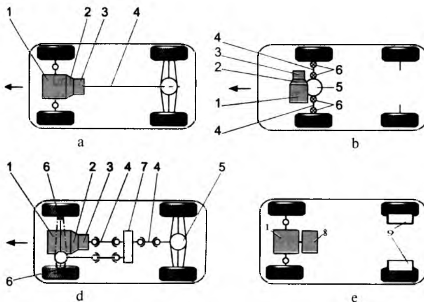
3.1-rasm. Avtomobillar transmissiyalarining sxemalari.
