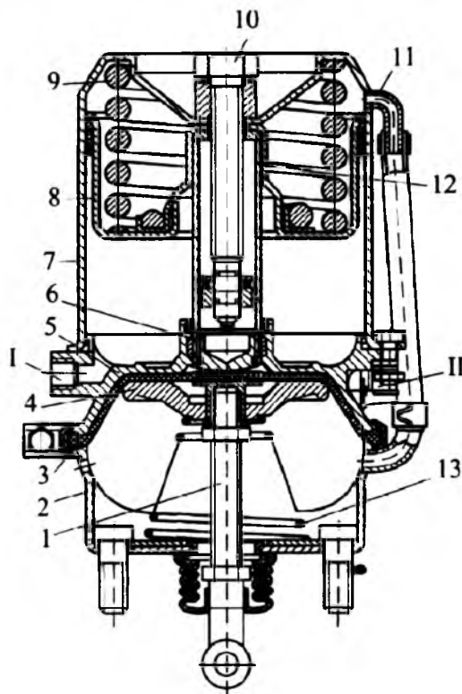
6.16-rasm. Energoakkumulyatorli tormoz kamerasi.
