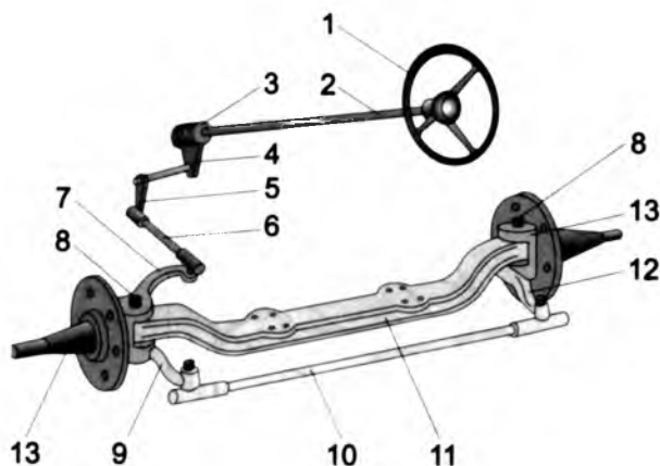
5.3-rasm. Nomustaqlil osmali avtomobil rul boshqarmasi sxemasi.
