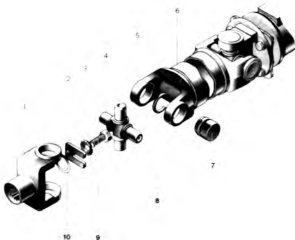
3.14-rasm. Burchak tezliklari teng bo'lmagan bikir kardan sharniri tarkibi:
