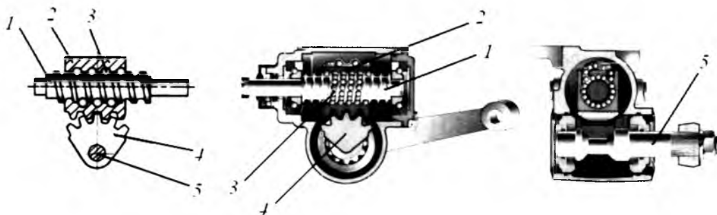
5.12-rasm. „Vint — gayka — reyka — sektor“ tipidagi rul mexanizmi.
