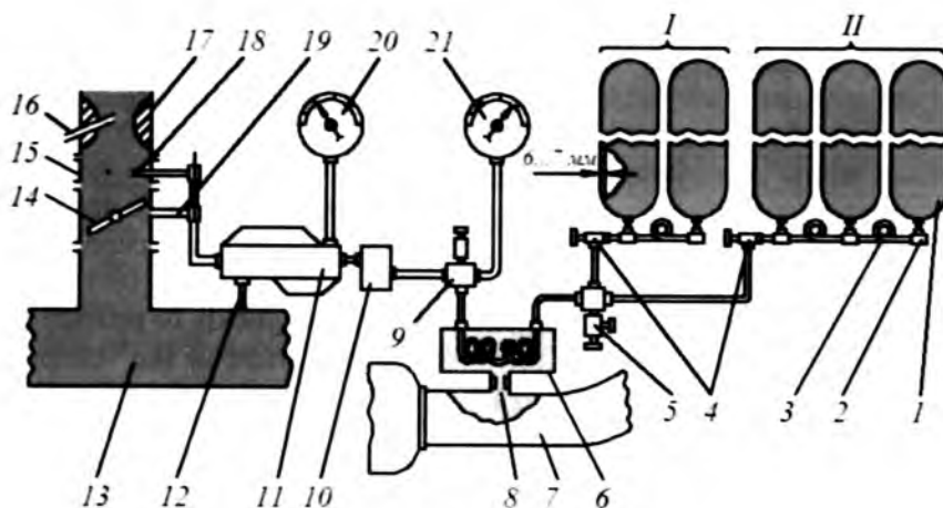
2.12-rasm. Gaz ballonli qurilmaning prinsipial sxemasi.
