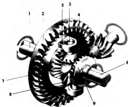
3.21-rasm. Differensial tuzilishini soddalashtirilgan sxemasi.
