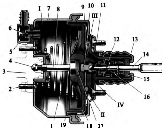
6.14-rasm. Yengil avtomobilning vakuum kuchaytirgichi:
