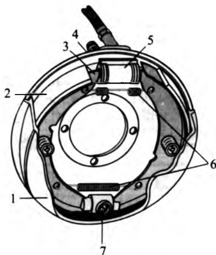
6.8-rasm. Barabanli tormoz mexanizmi:
