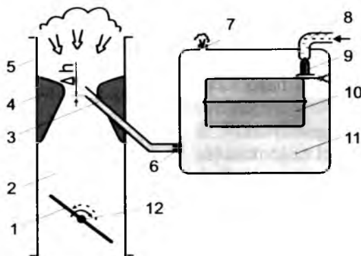
2.11-rasm. Oddiy karbyuratorning sxemasi.
