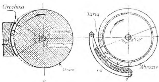
78-rasm. Tariq va grechixa donlarini valtsedeka uskunasi oqlash.
