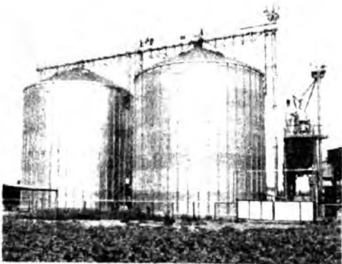
18-rasm. Donlarni saqlanadigan ombor turlarini zamonaviy ko‘rinishi.
