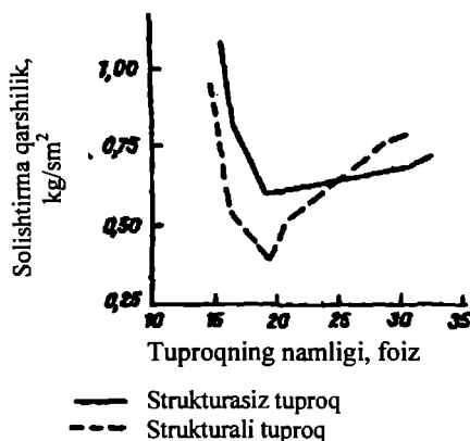
22- rasm. Strukturali va strukturasiz tuproqlar solishtirma qarshiligidan, uning namligiga bog'liqligi
