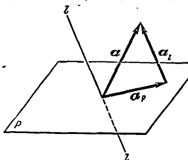
Рис. 151. a = a_p + a_z .
