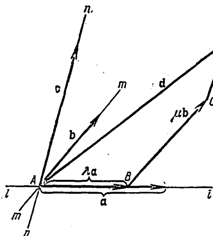
Рис. 150. d = \lambda a + \mu b + \nu c .
