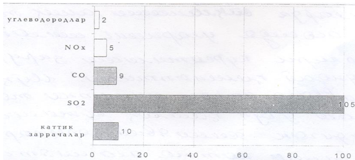
18-расм. Металлургия корхоналарининг ажратмалари (минг тонна ҳисобида).
