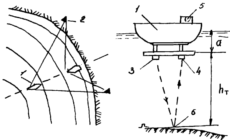
2.7-rasm. Exolot yordamida chuqurliklarni o'lchash:
