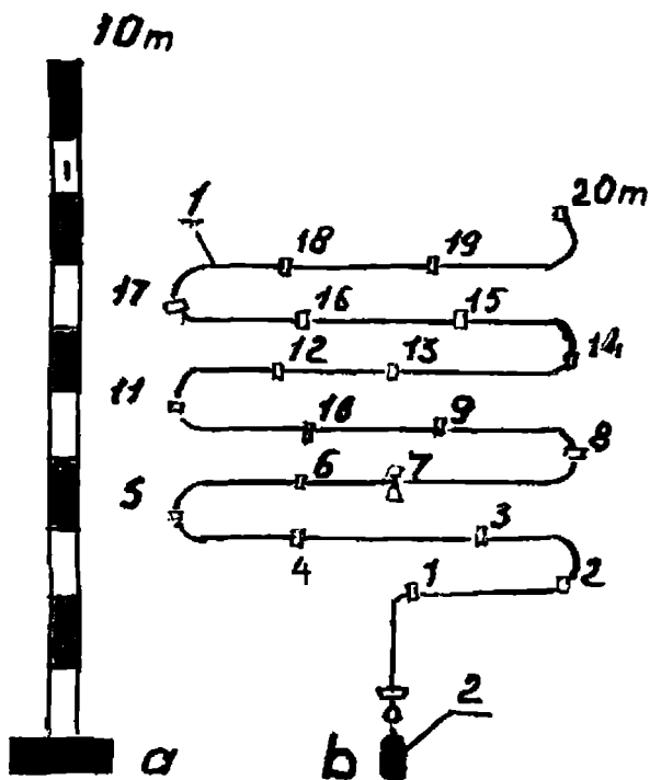
2.6-rasm. Reyka (a) va ko'l loti (b)
