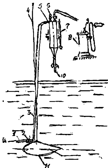
2.30-rasm. Vakuumli batometr
