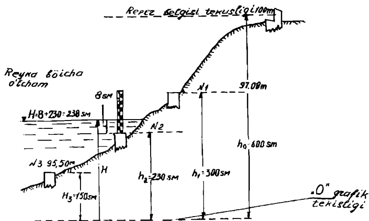
2.2-rasm. Qoziqli gidrologik postda o'lchanadigan suv sathi balandligining belgilari va sanoqlari chizmasi
