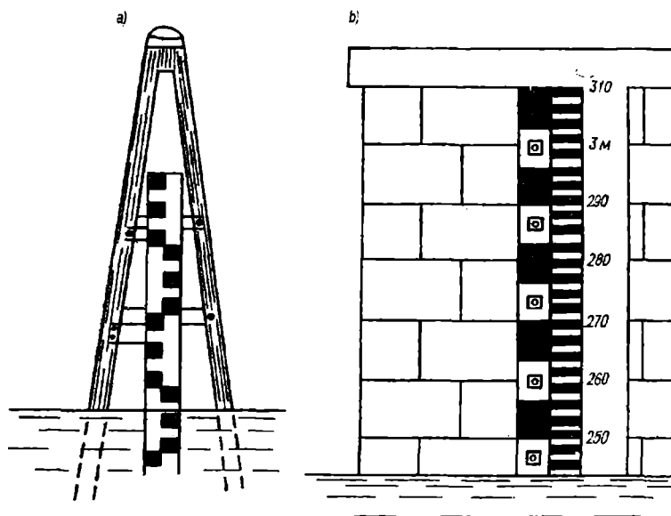
2.1-rasm. Reykali postlar:
