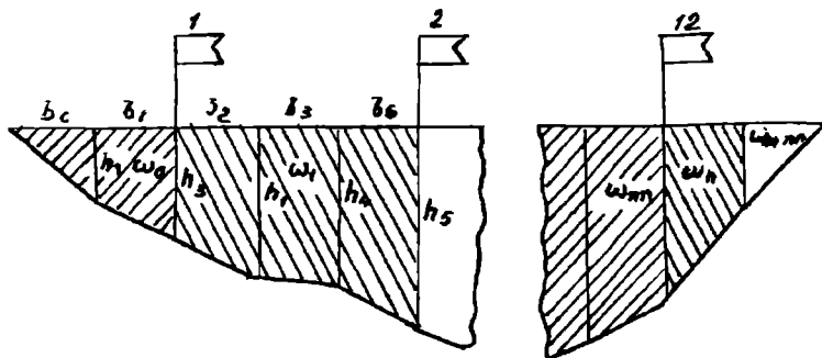
2.18-rasm. Ko‘ndalang kesim yuzasi (maydoni)ni hisoblash uchun chizma
