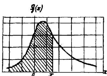
3.2-rasm. Tasodifiy sonlarning taqsimlanish egri chizig'i
