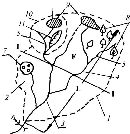
1.5-rasm. Daryo tizimi va qismlari:
