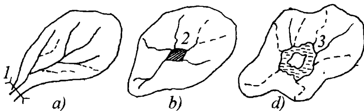
1.7-rasm. Suv yig'ilish maydonlarining turlari
