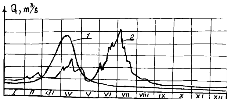
1.10-rasm. Tekislik (1) va tog'li (2) daryolar uchun tipik gidrograflar
