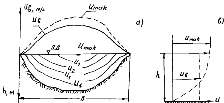
2.22-rasm. Oqim jonli kesimi bo'yicha tezliklarni taqsimlanishi:
