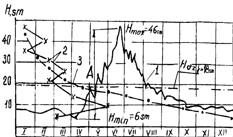
2.4-rasm. Suv sathining yillik grafigi:
