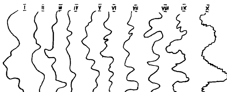
1.8-rasm. Daryo egriligi turlari
