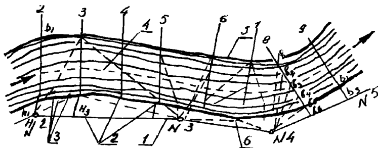
2.8-rasm. Suvning chuqurliklarini ko'ndalang kesimi bo'yicha o'lchash:
