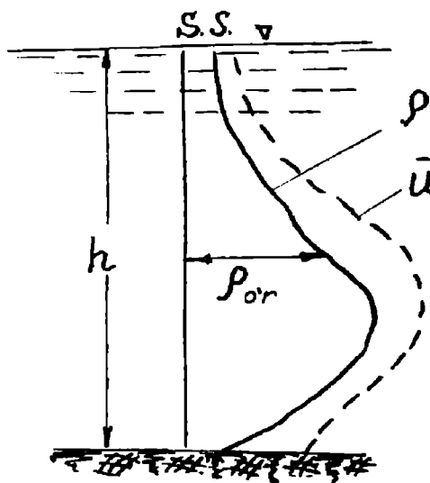
2.27-rasm. Oqiziq larni chuqurlik bo'yicha taqsimlanishi:
