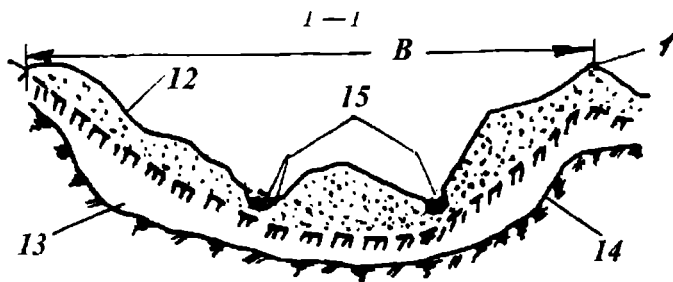
1.6-rasm. Havzaning ko'ndalang kesimi
