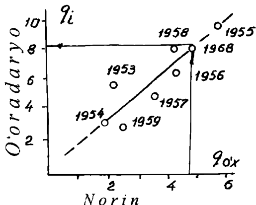
3.6-rasm. q_i = f(q_{o,x}) grafigi
