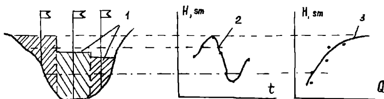
2.23-rasm. Suv sathining o'rtacha kunlik hisobini aniqlash chizmasi 1 – kuzatilgan sathlar; 2 – H=f(T) vaqt davomida suv sathining o'zgarish grafigi; 3 – Q=f(H) suv sarfini o'zgarish grafigi
