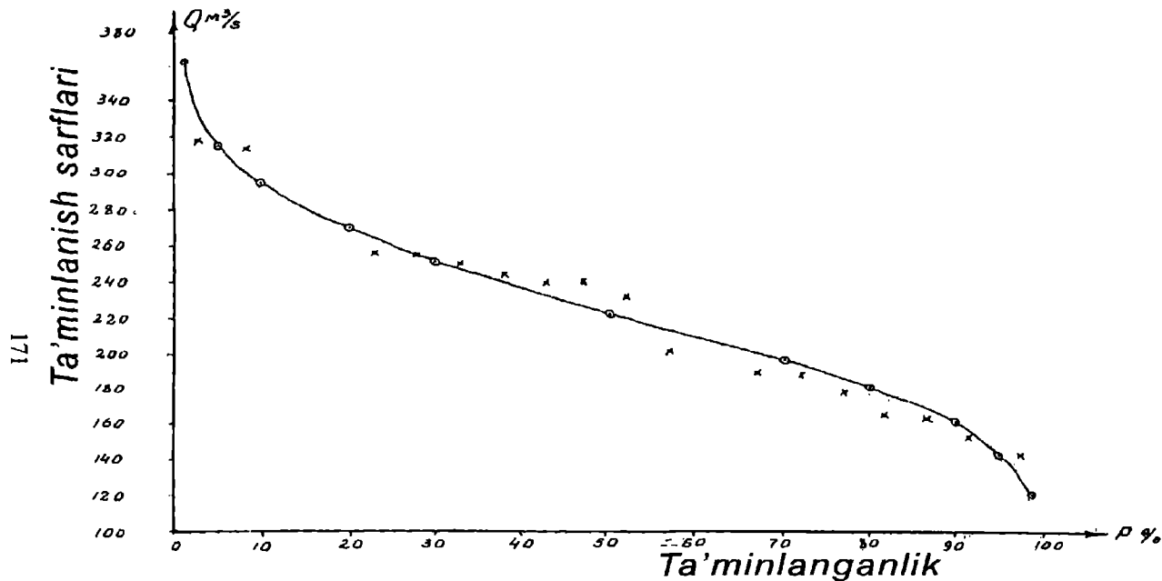
3.5-rasm. Chirchoq daryosining Xo'jakent postidagi amaliy ta'minlanganlik sarf nuqtalarining nazariy ta'minlanganlik egri chizig'i bilan taqqoslanishi. Shartli belgilari:
