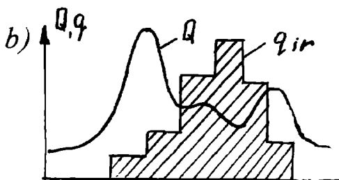
3.7. (b)-rasm. Oqimni murakkab rostlash gidrografi
