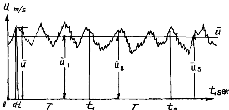
2.10-rasm. Nuqtadagi oniy tezlik grafigi
