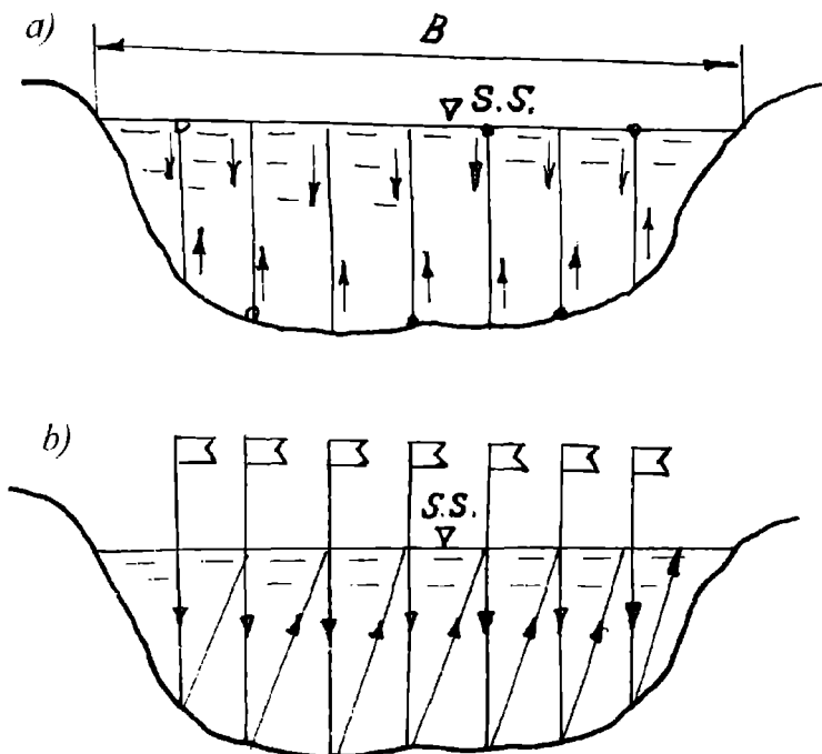
2.20-rasm. Integratsiya usuli bo'yicha oqim tezliklarini o'lchash a – vertushkani vertikkallar bo'yicha harakatlantirib tezlikni o'lchash; b – vertushkani oqim ko'ndalang kesim bo'yicha harakatlantirish; → – vertushkaning tezlik o'lchash mobaynida harakat yo'nalishi
