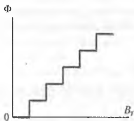
29.11-rasm. Halqa teshigida ushlanib qolgan magnit oqimi tashqi magnit maydon induktsiyasiga bog'liqlik grafigi.
