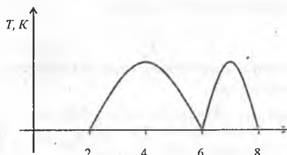
29.2-rasm. O'ta o'tkazuvchanlik holatiga o'tish temperaturasi valentli elektronlar soniga bog'liqligi grafiki.
