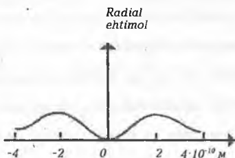
2p_x uyq'ongan holatda elektronning radial ehtimol zichligi
