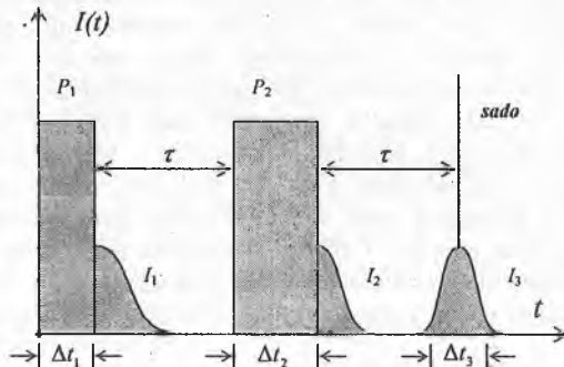
32.8-rasm. Vaqt bo'yicha foton sadosi. I(t) – javoblar (sadorlar) intensivligi: I_1 , I_2 va I_3 mos ravishda, 1–, 2–, 3– induksiya va sado intensivliklari; t –vaqt, P_1 va P_2 uyg'otuvchi impuls; \Delta t_1 va \Delta t_2 ularning davomiyliklari.
