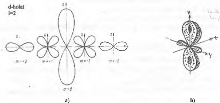
17.9-rasm. a) \theta - burchakka bog'liq bo'lgan p_\theta = |\theta_{2,1}, \theta_{2,1}| va p_\theta = |\theta_{2,2}, \theta_{2,2}| holat uchun ehtimol zichligi; b) To'la ehtimol zichlik, burchak ehtimol zichligi p_\theta bilan radial ehtimol zichligi p_r ga ko'paytmasi.
