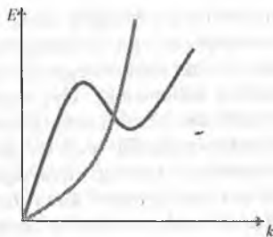
28.4-rasm. Real zarra va kvazizarralar uchun energiya va implus bog'liqligi grafiqi.
