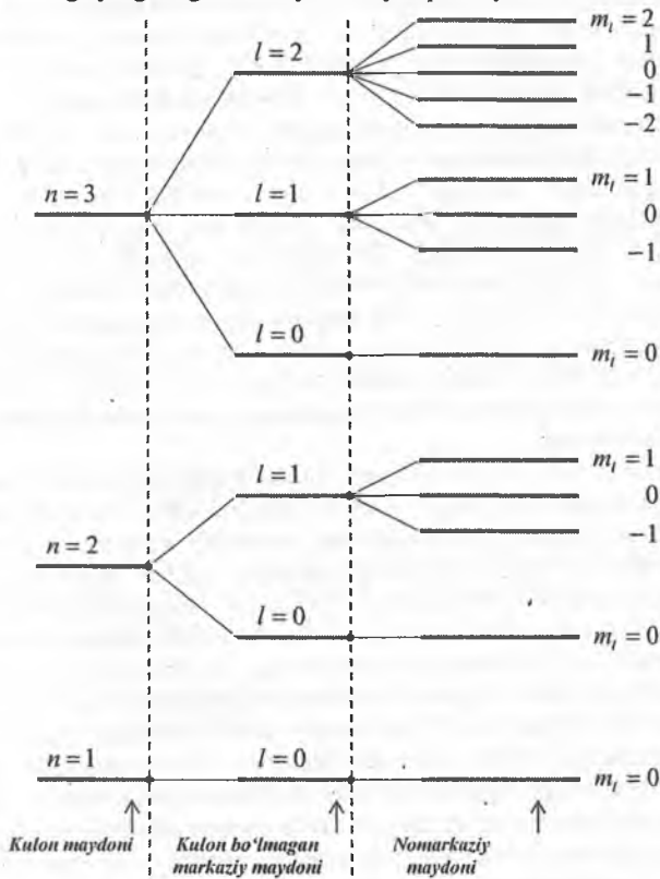
19.1- расм . Vodorod atomining energetik sathlarni aynishi va yo'qolishi yo'llari.
