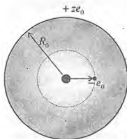
20.1-rasm. Vodorod atomi (Z=1) uchun Tomson modeli. Ze 0 musbat zaryad radiusi R 0 bo'lgan sfera ichida bir tekis taqsimlangan.
