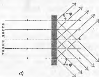
22.12-rasm. Gologrammada faqat tayanch dasta o'tishi ratijasida uchta to'liq hosil bo'lishi.
