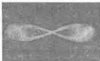
2p_x uyq'ongan holatda elektronning bo'lishi ehtimoli katta bo'lgan soha
