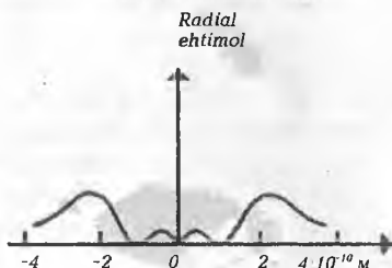
2s uyq'ongan holatda elektronning radial ehtimol zichligi
