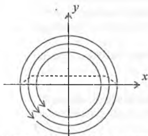
18.11-rasm. Doiraviy elektromagnit to'lqin paketida vaqt bo'yicha energiya oqimining sirkulatsiyasi.
