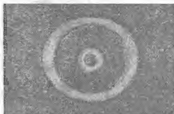
2s uyq'ongan holatda elektronning bo'lishi ehtimoli katta bo'lgan soha
