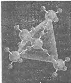
27.14-rasm. Germaniy strukturası.
