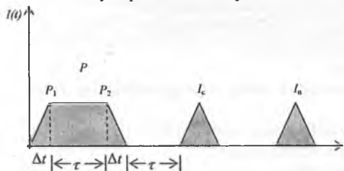
32.12-rasm. Chekkaviy va ko'p karrali sado. R uyg'otuvchi impuls, \Delta t va \tau chekkani davomligi va davomlilik, I_s - chekkaviy sado, I_k - ko'p karrali sado.
