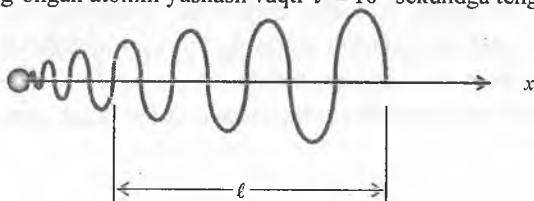
20.2-rasm. Yorug'lik impulsi yoki to'lqinlar sistemasini - sug.
