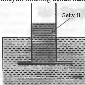
28.1-rasm. He-II ni o'ta oquvchanligi Ikkita silliqlangan shisha plastinka orasiidagi tor kanaldan Geliy-II bemolol oqib o'tadi. Suv esa bu kanaldan o'ta olmaydi.
