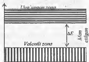
27.4-rasm. Kristallda energetik zonalarni soddalashtirilgan chizmasi.
