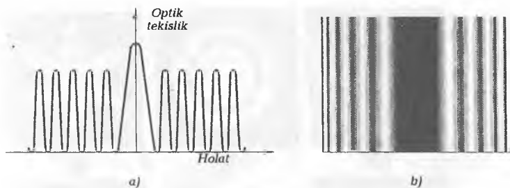
22.18-rasm. Yasssi va silindrik to'qlinlarni interferensiyasi tufayli intensivlikning taqsimlanishi.
