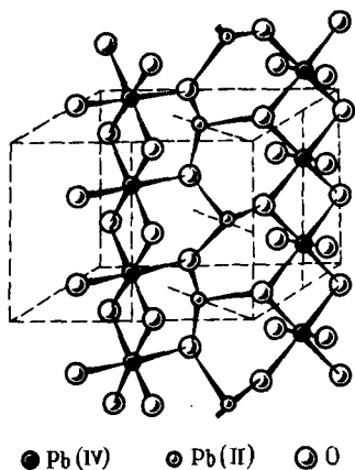
Р и с. 181. Структура сурика Pb_3O_4 ( Pb_2PbO_4 )
