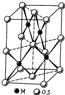
Р и с. 244. Структура \text{PdO} , \text{PtO} и \text{PdS}
