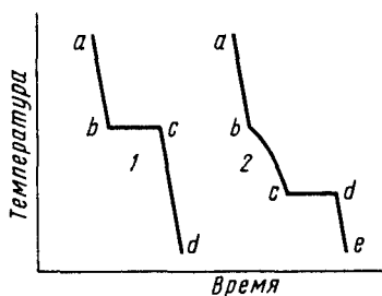
Р и с. 78. Кривые охлаждения:
