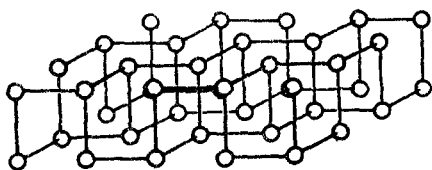
Рис. 164. Расположение атомов в кристалле черного фосфора
