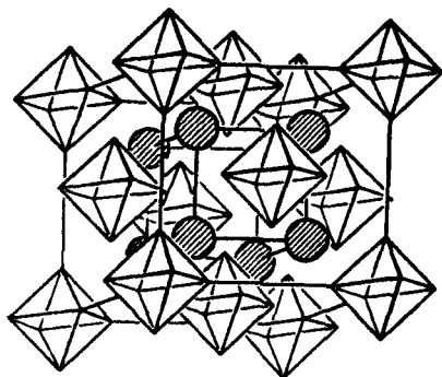
Р и с. 68. Кристаллическая решетка соединений типа: \overset{+1}{M}_2[\overset{+2}{M}(\text{Э}Hal_6)] или [\overset{+2}{M}(\text{NH}_3)_6]X_2 :
