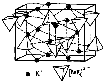
Р и с. 201. Структура \text{K}_2\text{BeF}_4
