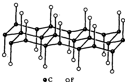
Р и с. 175. Структура фторида графита CF
