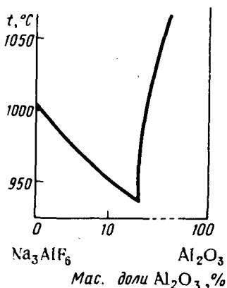
Рис. 190. Фрагмент диаграммы плавкости системы \text{Na}_3\text{AlF}_6 - \text{Al}_2\text{O}_3
