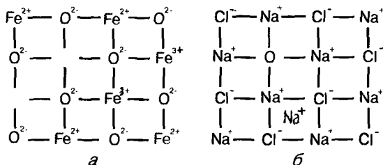
Р и с. 138. Катионный дефект в кристалле \text{FeO} ( a ) и анионный дефект в кристалле \text{NaCl} , легированном натрием ( б )
