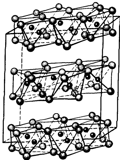
Рис. 191. Структура гидраргилита \text{Al(OH)}_3
