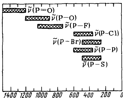
Р и с. 93. Волновые числа, характеризующие валентные колебания атомных группировок соединений фосфора
