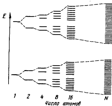
Рис. 71. Построение энергетических зон при последовательном присоединении атомов
