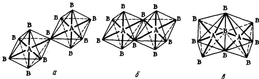
Р и с. 61. Двухъядерные комплексы:
