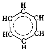
бензол
