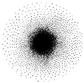
Рис. 2. Электронное облако
