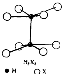
Р и с. 235. Структура двухъядерного кластера типа M_2X_8 на примере K_2[Re_2Cl_8] \cdot 2H_2O
