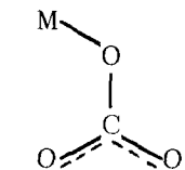
монодентатный
