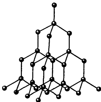
Рис. 65. Структура алмаза
