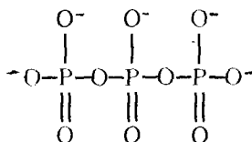
P_3O_{10}^{5-} трифосфат-ион
