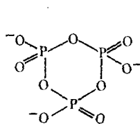
(PO_3)_3^{3-} триметафосфат-ион
