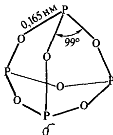
Рис. 165. Пирамидальная структурная единица (а) и строение молекулы \text{P}_4\text{O}_6 (б)
