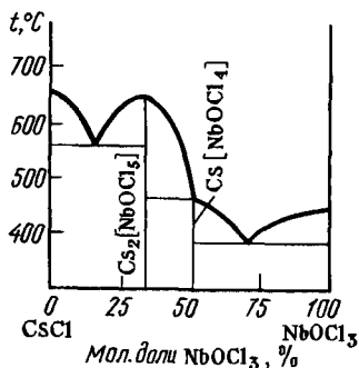
Р и с. 231. Диаграмма плавления системы \text{CsCl} - \text{NbOCl}_3
