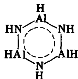
алазол
