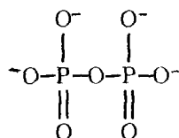
P_2O_7^{4-} дифосфат-ион
