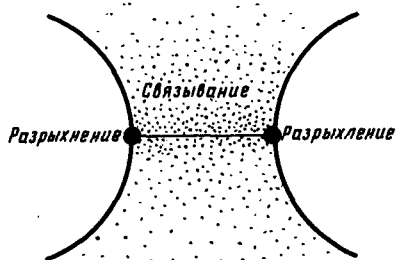
Р и с. 19. Области связывания и разрыхления в молекулярном ионе \text{H}_2^+
