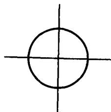
Рис. 3. Сечение границной поверхности
