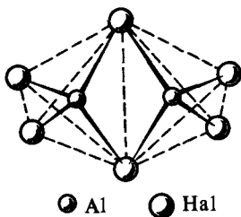
Р и с. 194. Строение молекулы \text{Al}_2\text{Hal}_6
