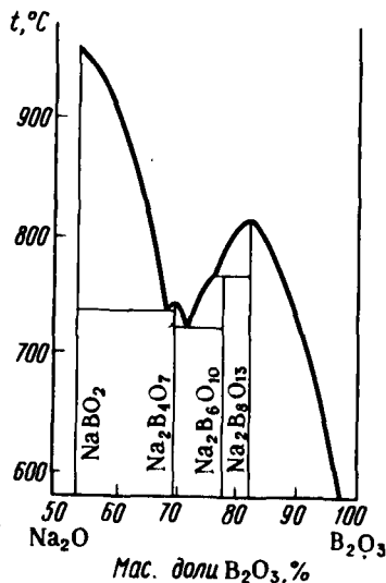
Р и с. 189. Диаграмма плавкости системы \text{Na}_2\text{O}-\text{B}_2\text{O}_3
