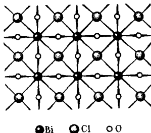
Р и с. 171. Структура слоя кристаллического \text{BiOCl} : атомы О и Cl лежат соответственно выше и ниже плоскости из атомов Bi
