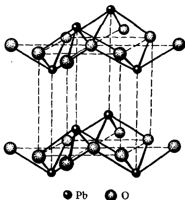
Р и с. 183. Структура PbO
