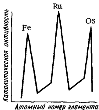
Р и с. 160. Зависимость каталитической активности ряда металлов в реакции 2\text{NH}_3 = \text{N}_2 + 3\text{H}_2 (800°C, 1 \cdot 10^5 Па) от атомного номера элемента
