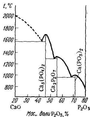
Рис. 167. Диаграмма плавления системы CaO - P_2O_5
