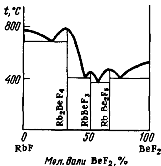
Р и с. 200. Диаграмма плавления системы \text{RbF} - \text{BeF}_2
