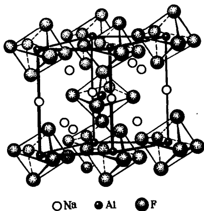
Р и с. 195. Структура криолита \text{Na}_3\text{AlF}_6
