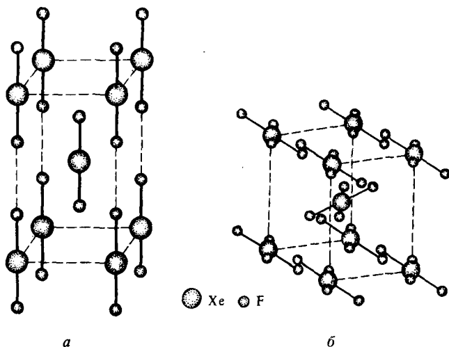
Р и с. 209. Структура кристаллов \text{XeF}_2 ( a ) и \text{XeF}_4 ( б )
