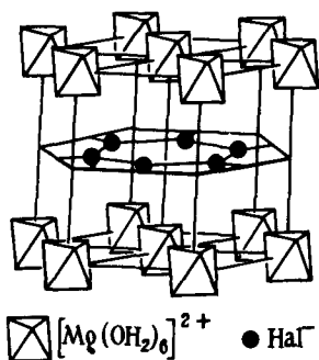
Р и с. 202. Структура бишофита MgCl 2 ·6H 2 O
