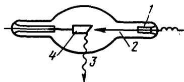
Р и с. 86. Схема рентгеновской трубки
