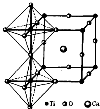
Рис. 70. Структура перовскита CaTiO_3
