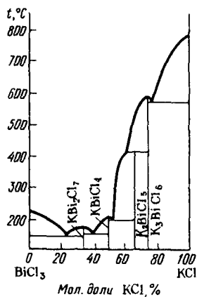
Р и с. 170. Диаграмма плавок-ности системы \text{BiCl}_3 - \text{KCl}
