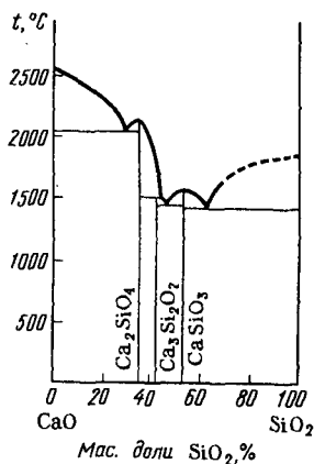
Р и с. 178. Диаграмма плавкости системы \text{CaO} - \text{SiO}_2
