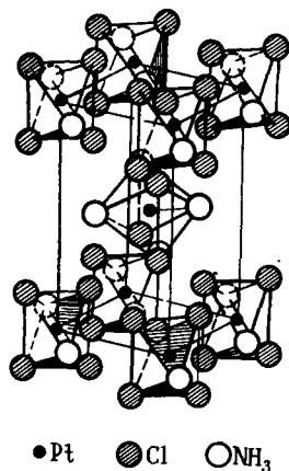
Р и с. 249. Строение кристалла [\text{Pt}(\text{NH}_3)_2\text{Cl}_4]
