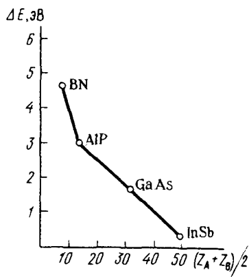
Рис. 199. Зависимость ширины запрещенной зоны \Delta E в соединениях типа A^{III}B^V от среднеарифметического атомного номера
