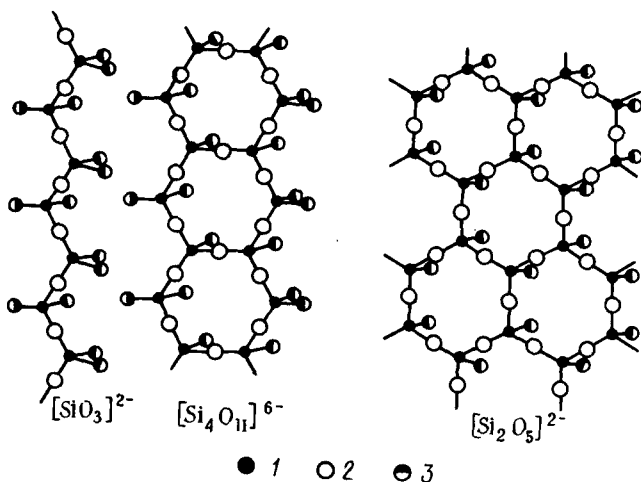
Р и с. 179. Полимерные оксосиликатные ионы:
