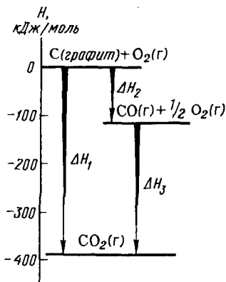
Рис. 109. Энтальпийная диаграмма окисления графита
