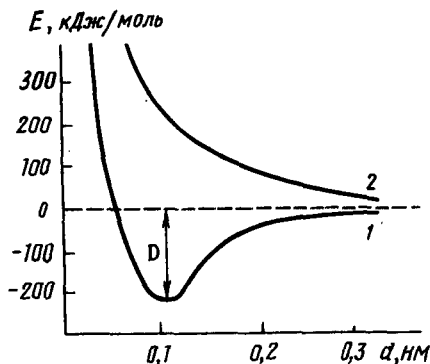
Р и с. 20. Зависимость потенциальной энергии молекулярного иона \text{H}_2^+ при нахождении электрона в связывающей (кривая 1) и разрыхляющей (кривая 2) области
