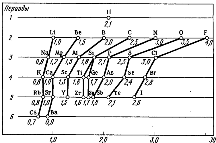
Р и с. 13. Шкала электроотрицательностей по Полингу
