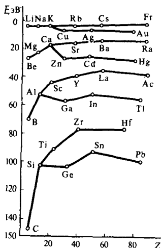
Р и с. 210. Зависимость энергии ионизации атомов в подгруппах s -, p - и d -элементов от атомного номера элемента: для I группы приведены значения E_1 , для II группы — E_1 + E_2 , для III — E_1 + E_2 + E_3 , для IV группы — E_1 + E_2 + E_3 + E_4
