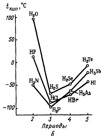
Р и с. 148. Температуры плавления (а) и кипения (б) водородных соединений p -элементов VII, VI, V групп
