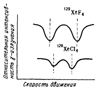
Р и с. 99. \gamma -Резонансные спектры молекул \text{XeCl}_4 и \text{XeF}_4
