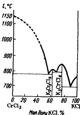
Р и с. 237. Диаграмма плавок- ти системы \text{CrCl}_3 - \text{KCl}
