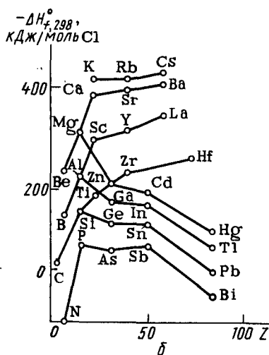
Р и с. 132. Зависимость энтальпии образования высших оксидов (а) и хлоридов (б) от атомного номера элемента с положительной степенью окисления
