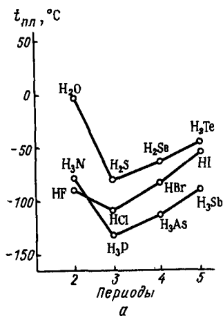
Р и с. 148. Температуры плавления (а) и кипения (б) водородных соединений p -элементов VII, VI, V групп
