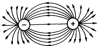
Рис. 56. Распределение электрических силовых полей двух разноименных ионов
