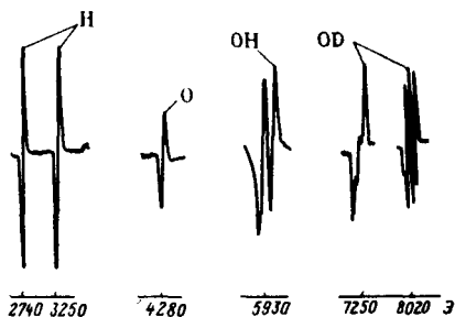
Р и с. 96. Спектры ЭПР атомов Н и О, свободных радикалов ОН и ОД
