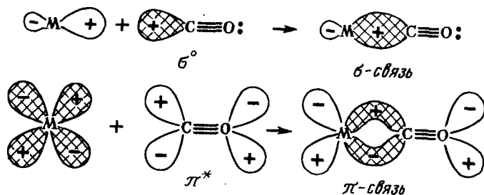
Р и с. 232. Схема образования \sigma - и \pi -связей M - CO в карбонилах d -элементов:
