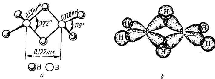
Рис. 185. Строение ( a ) и схема перекрывания атомных орбиталей ( b ) в молекуле \text{B}_2\text{H}_6 .
