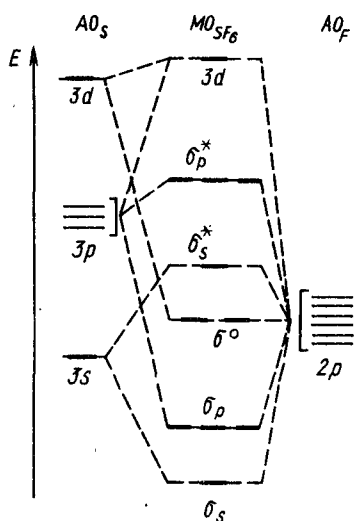
Р и с. 144. Энергетическая диаграмма орбиталей октаэдрической молекулы \text{SF}_6
