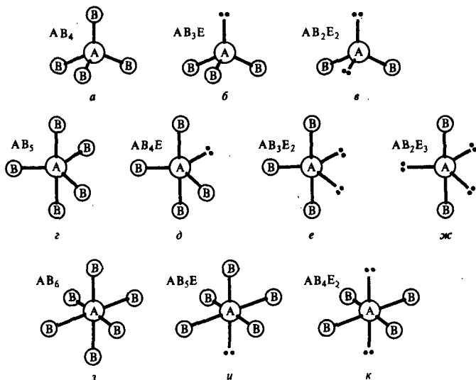
Р и с. 51. Влияние связывающих и несвязывающих электронных пар (Е) центрального атома на пространственную конфигурацию молекул:
