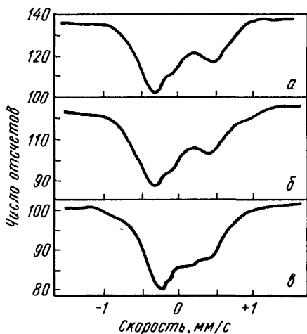
Р и с. 241. \gamma -Спектры берлинской лазури (а) и турбуллевой сини (б) и солей \text{KFe}^{\text{+3}}\text{Fe}^{\text{+2}}(\text{CN})_6 и \text{KFe}^{\text{+2}}\text{Fe}^{\text{+3}}(\text{CN})_6 (в)
