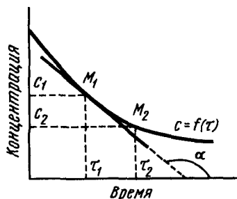
Р и с. 114. Изменение концентрации исходных веществ в процессе реакции
