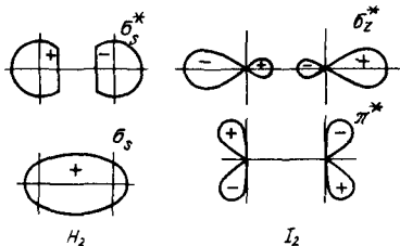
Р и с. 117. \sigma_s , \sigma_s^* -Орбитали H_2 и \pi^* , \sigma_z^* -орбитали I_2
