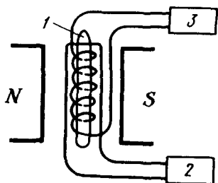
Рис. 94. Схема радиоспектроскопа для исследования ЯМР:
