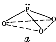
Рис. 165. Пирамидальная структурная единица (а) и строение молекулы \text{P}_4\text{O}_6 (б)
