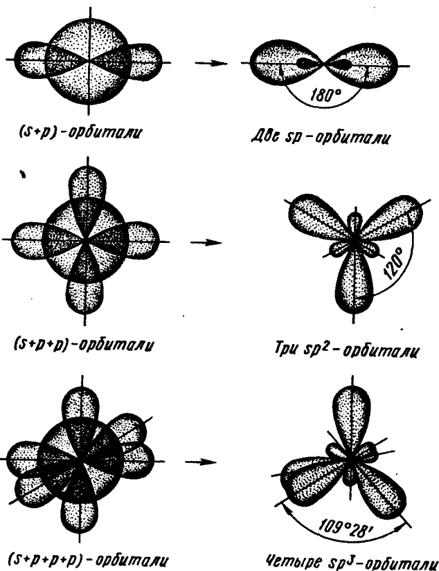
Р и с. 48. Гибридизация валентных орбиталей
