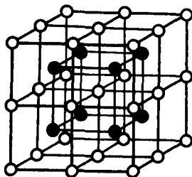
CsCl
