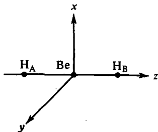
Р и с. 32. Взаимное расположение атомов в молекуле \text{BeH}_2
