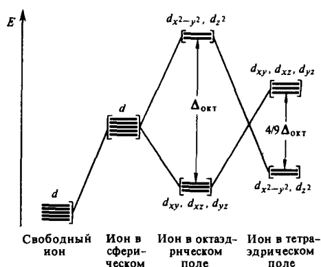
Р и с. 212. Расщепление d -уровня кристаллическим полем разной симметрии
