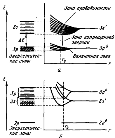
Р и с. 72. Возникновение энергетических зон кристаллов NaCl (а) и Na (б) из энергетических уровней атомов по мере их сближения: а — зоны не перекрываются; б — зоны перекрываются
