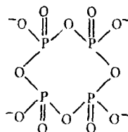
(PO_3)_4^{4-} тетраметафосфат-ион
