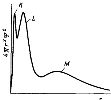
Рис. 11. Распределение электронной плотности в атоме аргона
