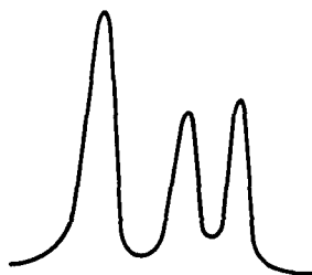
Рис. 95. Спектр ЯМР (протонов) этанола \text{C}_2\text{H}_5\text{OH}
