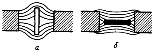
Р и с. 106. Поведение в магнитном поле диа- ( а ) и парамагнитных ( б ) веществ
