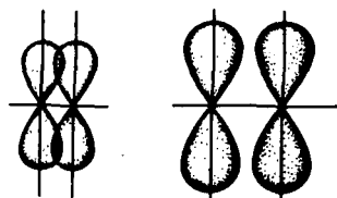
Р и с. 147. Влияние междядерного расстояния на степень перекрывания p\pi - p\pi -связей
