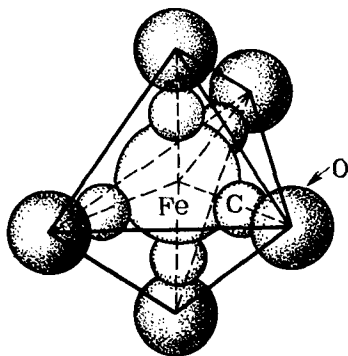
Р и с. 240. Структура молекулы пентакарбонила железа \text{Fe}(\text{CO})_5
