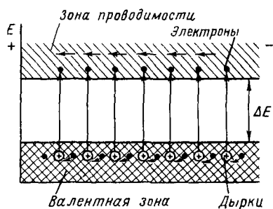
Р и с. 73. Зонная схема собственной проводимости полупроводников
