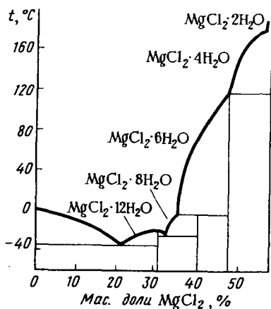
Р и с. 203. Диаграмма плавления системы H 2 O — MgCl 2
