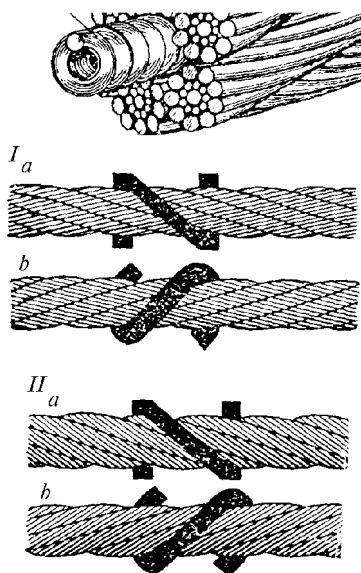
9-rasm. Har xil o'ramli po'lat arqon:
