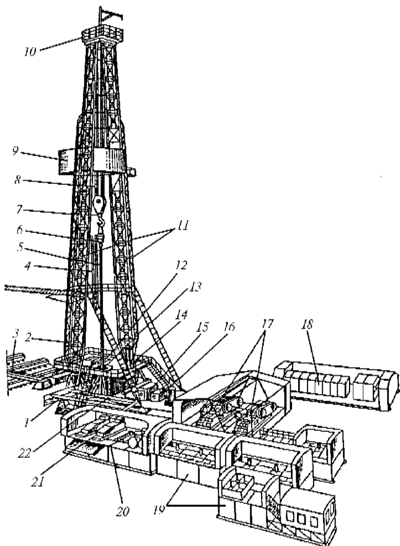
1-rasm. A-koʻrinishdagi burgʻilash minorasi:
