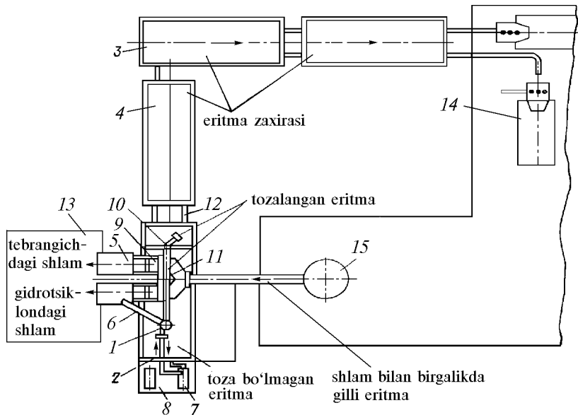
29-rasm. «Уралмаш 5Д» va «Уралмаш 6Е»GTS kompanovkasining sxemasi: 1 — gidrotsiklon; 2 — ( V = 30 \text{ m}^3 ) blok sig'imi; 3 — ( V = 30 \text{ m}^3 ) yarim silindrsimon buriluvchi sig'imi; 4 — ( V = 30 \text{ m}^3 ) yarim silindrsimon sig'im; 5 — nov; 6 — gidrotsiklonli
