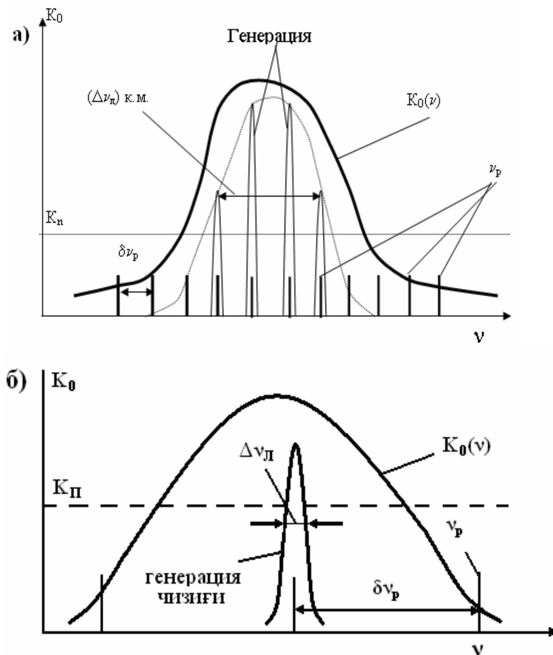
14-рasm. Кучайтириш K(\nu) чизигининг профили ва лазер генерациясининг кўп частотали (а) ҳамда якка частотали (б) спектрларининг графиги.
