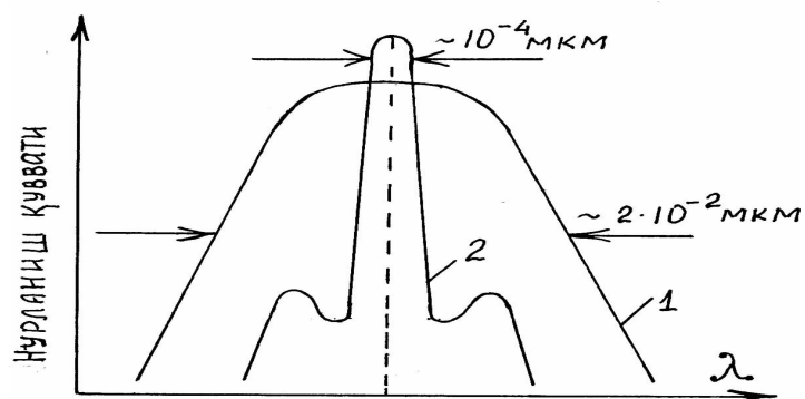
29-расм. Яримўтказгичли р–п ўтишда ишловчи инжекцияли лазернинг спектрал характеристикаси.
