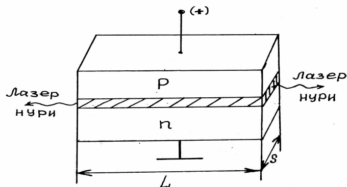
28-расм. Яримўтказгичли р–п ўтишда ишловчи инжекцияли лазернинг конструкцияси кўрсатилган.
