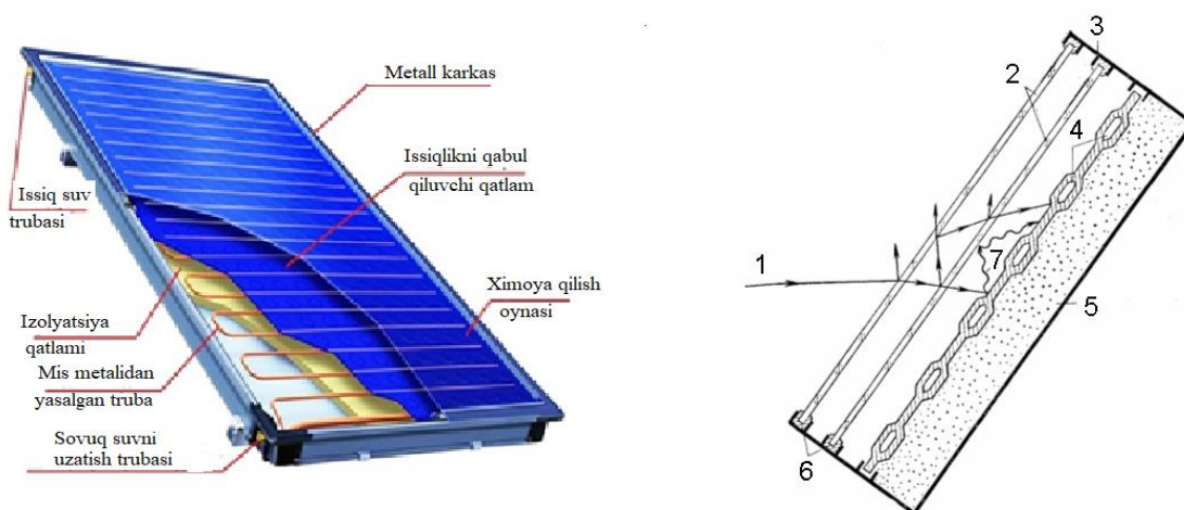
56-расм. Ясси қуёш коллекторининг конструктив тузилиши
