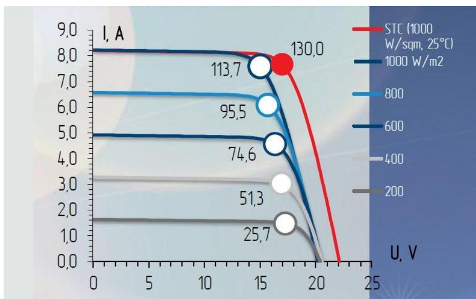
21-расм. Қуввати 130 Вт монокристалл турдаги фотоэлектрик модулниң ёритилганликка боғлиқлик ВАХ.
