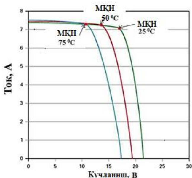
43-расм. Панел ҳароратига боғлиқ равишда максимал қувват нуқтасида қуёш панели кучланиши
