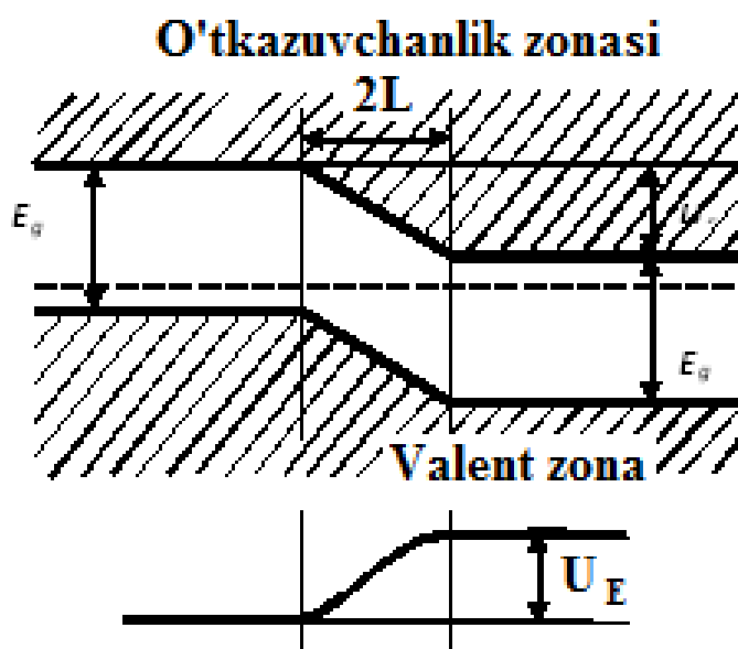
23-расм. Ёритилмаган p-n ўтишли ярим ўтказгичда энергетик зоналар структураси (а), электростатик потенциал тақсимоти (б). 2l – фазовий заряд соҳасининг кенглигини, U_E – p- ва n- соҳалар чегарасидаги мувозанат ҳол учун электростатик потенциал, E_g – ман қилинган соҳа кенглиги, штрихланган чизик – мувозанат ҳоли учун Ферми сатҳи.
