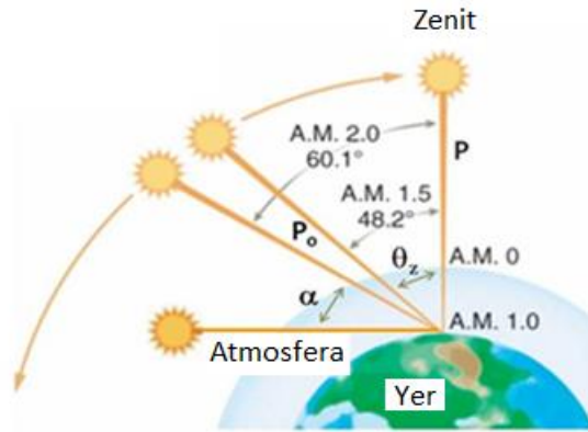
4-расм. Горизонтга нисбатан ҳар хил баландликларда Қуёш нурланишининг атмосферадан ўтиш масофаси
