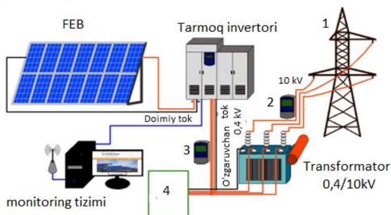
45-расм. Электр тармоғи билан интеграллашган ФЭС нинг структуравий схемаси
