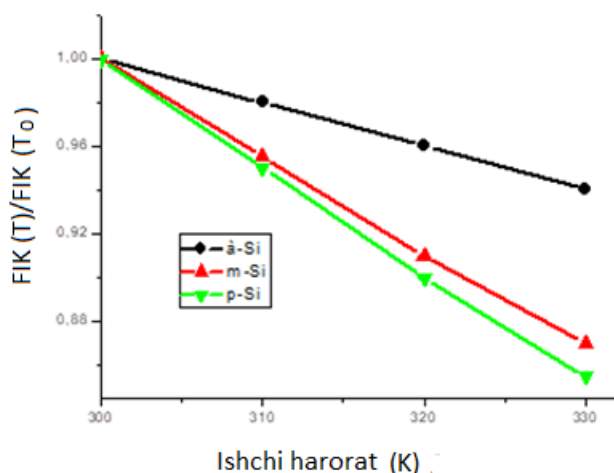
20-расм. Ҳар хил турдаги ҚЭ электрик самарадорлигининг ишчи ҳароратга боғлиқлиги
