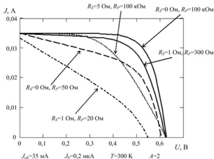
22-расм. Кетма-кетлик ( R_s ) ва параллеллик қашиликларининг ( R_p ) ҚЭ ВАХ га таъсири
