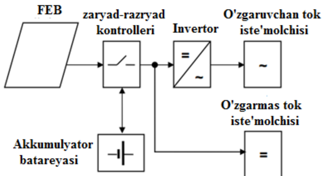
38-расм. АФЭС нинг соддалашган структуравий схемаси
