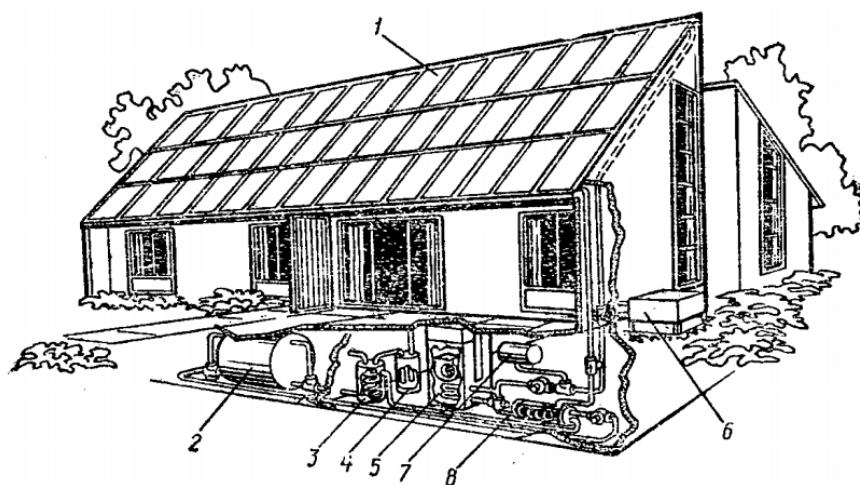
73-расм. Актив гелиотизимли иссиқлик таъминотида эга уй
