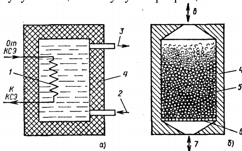
68-расм. Сифим туридаги иссиқлик аккумуляторлари— сувли (а) ва майда гранит тошли (б):
