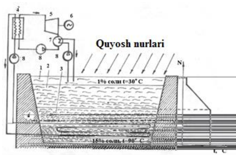
67-расм. Қуёш сунъий кўли (сув омбори) кесими энергиядан фойдаланиш таъминоти ва суюқликнинг кўл баландлиги бўйича ҳарорати ўзгариши.
