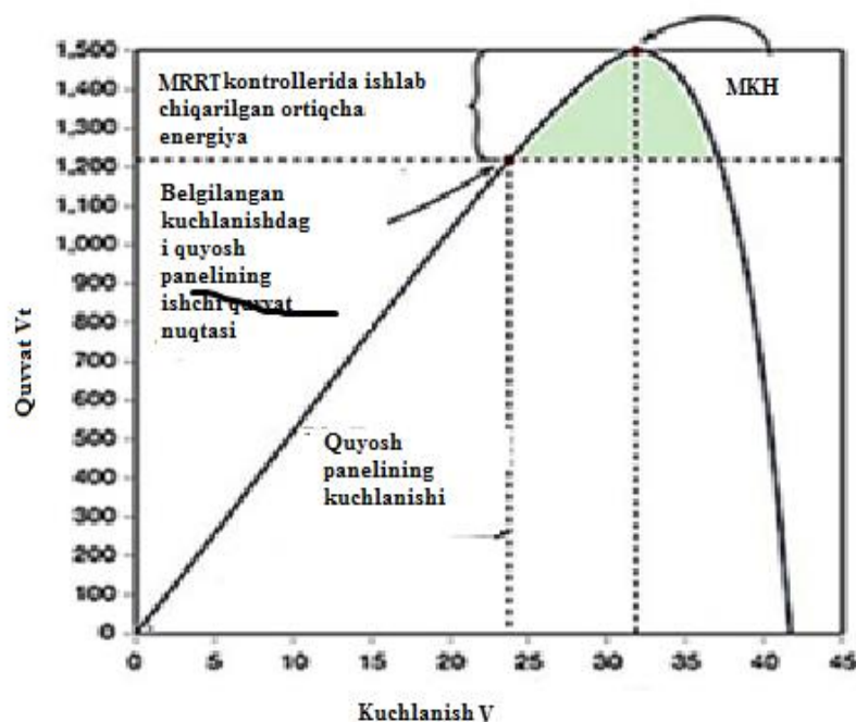
42-расм. МРРТ – контроллердан фойдаланганда қўшимча равишда олинган энергия миқдори
