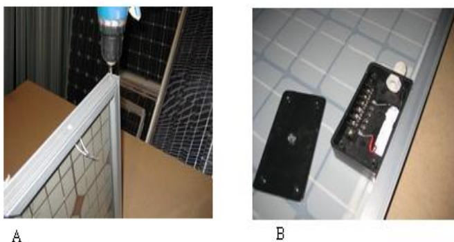
33-расм. А-алюминий каркасни монтаж қилиш; В-клеммали қутини ўрнатиш
