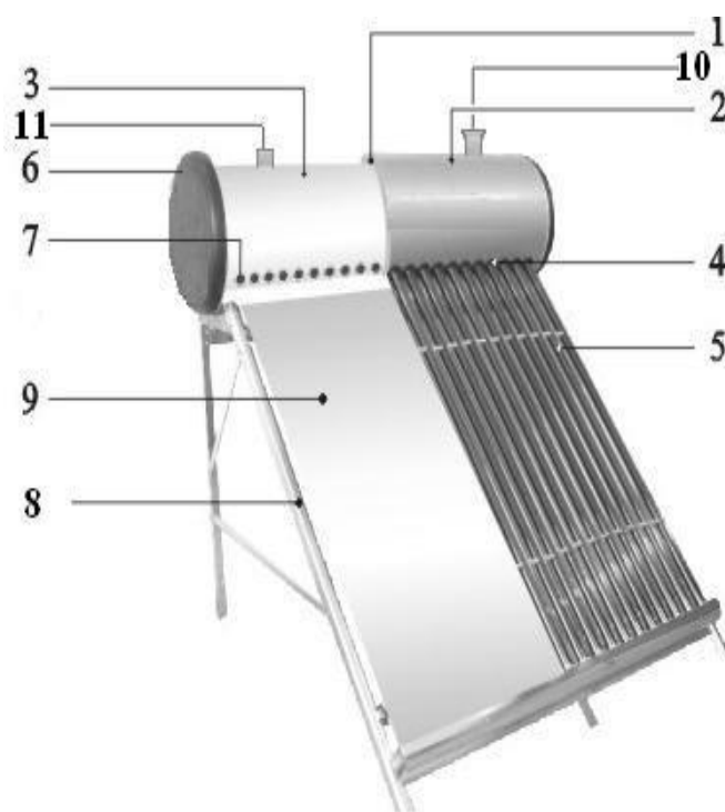
58-расм. Бутун турдаги вакуум трубкали коллектор
