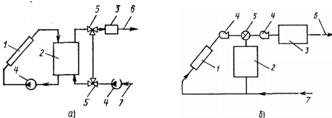
72-расм. Қуёший иситишнинг сувли (а) ва ҳаво асосидаги (б) актив тизимлари.
