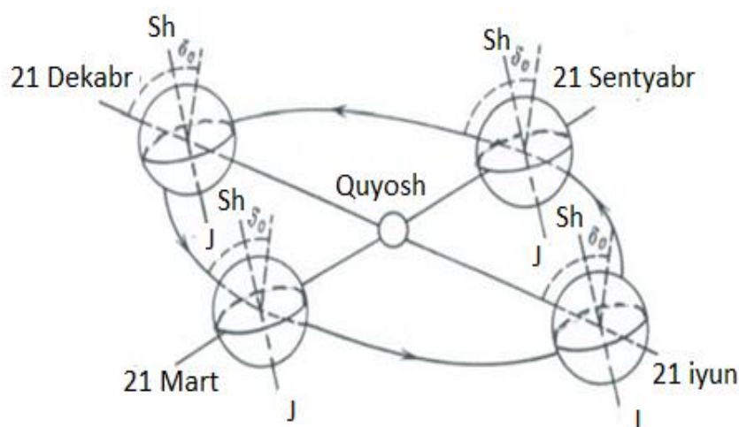
9-расм. Қуёш атрофида Ернинг айланиш схемаси. Ер юзасидаги ўрта чизик – экватор
