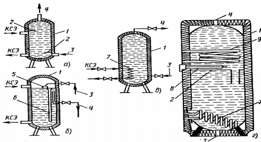
69-расм. Иссиқ сув аккумуляторлари - баклар
