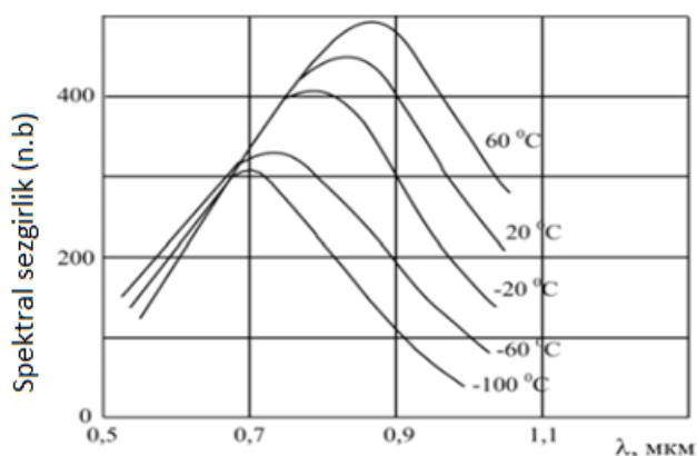
19-расм. Кремнийли ҚЭ спектрал сезгирлигининг ҳароратга боғлиқлиги
