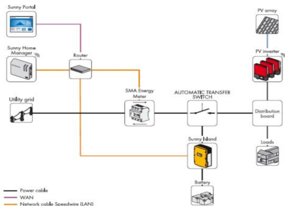
49-расм. Резерв истеъмол функциясига эга фотоэлектрик электр таъминот тизимининг структуравий схемаси
