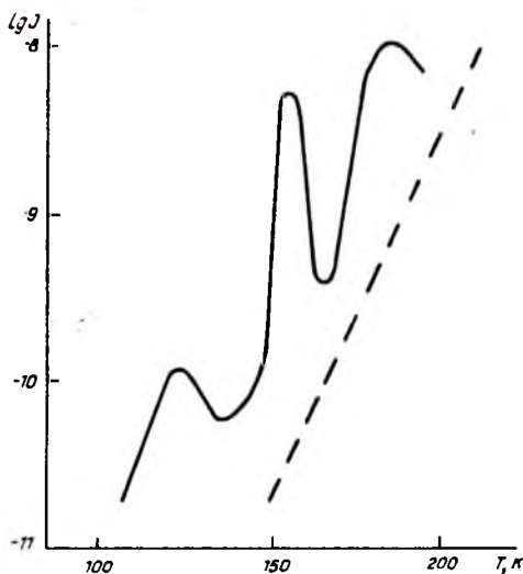
6.4- расм. Sb_2Se_3 намунасида иссиқлик билан кўзғатилган (индукцион) токнинг ҳароратга боғлиқлиги графиги.
