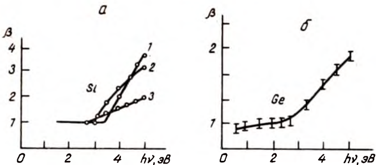
3.11- расм. а) Кремнийда фотоионланиш квант чиқишининг спектрал боғланиши: 1—100 К, 2—300 К, 3—400 К да; б) хусусий ютилиш соҳасида ёруғлик билан қўзғатилган германийда фотоионланиш квант чиқиши спектри.
