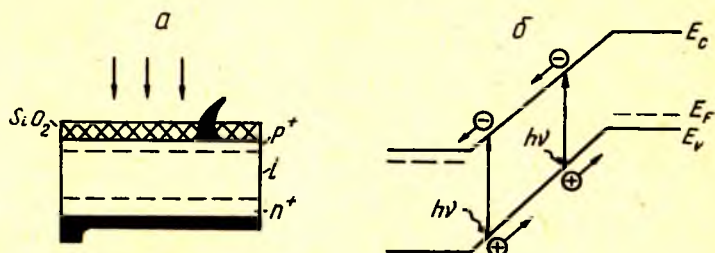
8.3- расм. Рўпарасидан ёритилган кремний p-i-n фотодиод (а) ҳамда тескари кучланиш берилган p-i-n диоднинг (б) энергетик зоналар диаграммаси.
