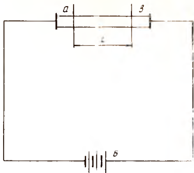
5.5- расм. Ҳаракатчанликни ўлчашнинг умумий схемаси.
