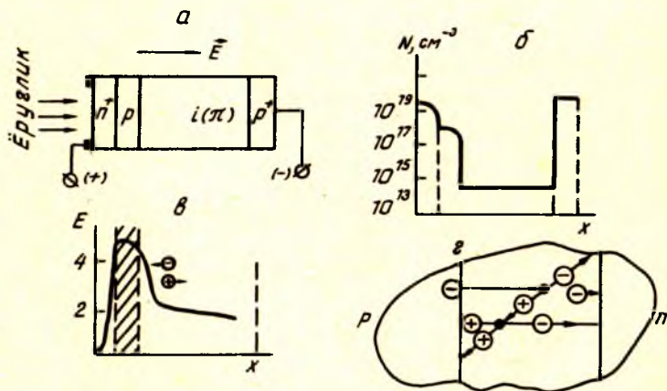
8.7- расм. Қўчкили — учма фотодиод тузилиши (а), киришмалар концентрациясининг x га боғланиши (б), электр майдон тақсимооти (в), p-n -ўтиш соҳасида зарбдан ионланиш жараёнининг ривожланиши (г).
