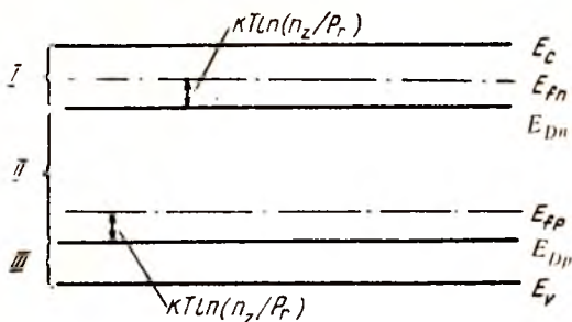
4.24- расм. Номувозанат ҳолатдаги яримўтказгичларда демаркацион сатҳлар:
