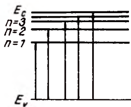
3.5- расм. Яримўтказгичда экситоннинг энергетик сатҳлари.
