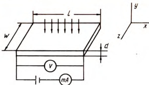
7.2- расм. Хусусий фотоўтаказувчанликни ҳисоблашга оид чизма.
