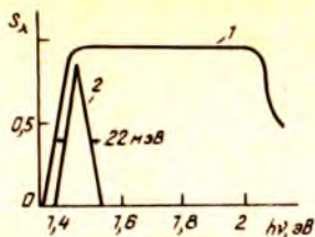
8.23- расм. p\text{Al}_x\text{Ge}_{1-x}\text{As} - n\text{GaAs} гетероўтишнинг (1) ёруғликни танловчан қабул қилгичнинг (2) спектрал тақсимооти.
