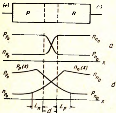
3.19- расм. p — n ўтиш соҳасида асосий ва асосий бўлмаган заряд ташувчиларнинг мувозанат ҳолатидаги (а), кучланиш тўғри йўналишда қўйилган ҳолати (б) тақсимоми.
