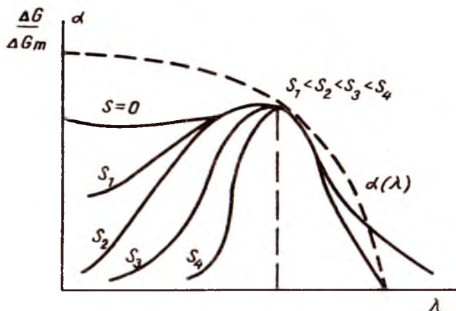
7.3- расм. Хусусий фотоўтказувчанликнинг ёруғликнинг тўлқин узунлигига боғлиқлиги.
