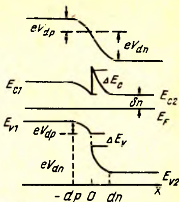
8.15- расм. Алоҳида-алоҳида олинган икки яримўтказгичнинг (а) ва бенуксон анизотип p-n гетероўтишнинг (б) Андерсон зоналар диаграммаси модели.
