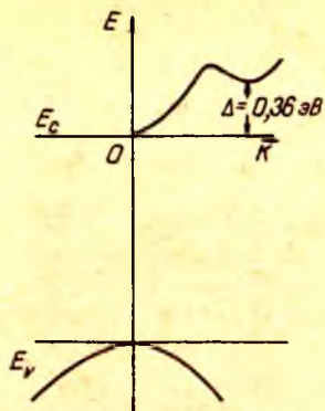
1.4- расм. GaAs ўтказув- чанлик зонаси модели.
