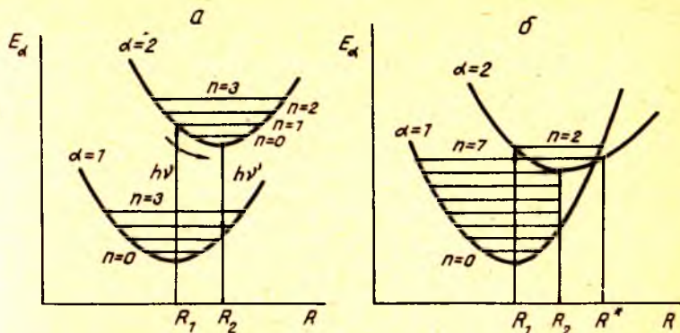
4.17- расм. Кристаллдаги нуқсон потенциал энергиясининг (тула электрон энергияси кирган ҳолда) конфигурацион координата E_s(R) га боғланиши:
