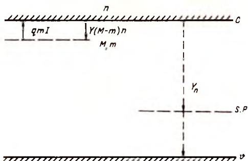
6.3- расм. Индукцияланган ток ходисасида электрон ўтишлар схемаси.
