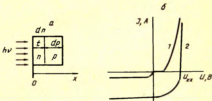
8.2- расм. Юпка p-n -ўтишли фотозэлемент (а) ва фотодиоднинг вольт-ампер характеристикаси (б).
