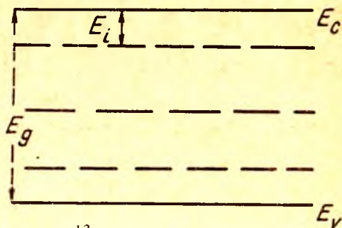
1.6- расм. Тақиқланган зонада нуқсонлар ҳосил қилган сатҳлар.
