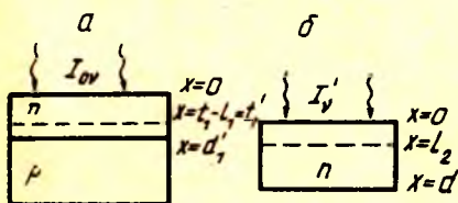
8.21-расм. Сирт қатламидаги (а) ва асос соҳасидаги (б) фототокни ҳисоблаш учун (гетероўтиш соҳасидаги) координаталар системаси ( x=t' ва x=l_2 чизиклар оралиғи билан гетероўтишнинг камбағаллашган соҳаси белгиланган).
