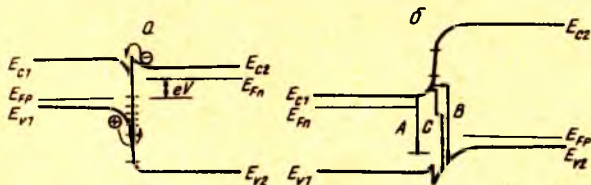
8.18- расм. Тўғри кучланиш қўйилган p-n гетероўтишнинг энергетик зоналар диаграммаси (а) ва p-n ўтишда зарядларнинг туннел рекомбинация жараёнлари орқали кўчишларининг турли йўллари (б).
