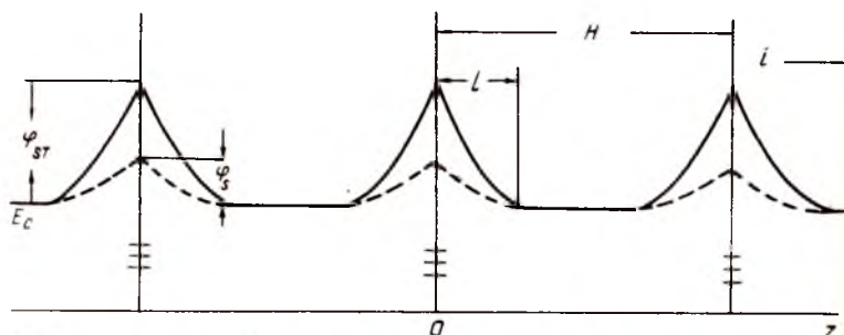
6.9- расм. p -тип яримўтказгичда нотекис тақсимланган акцептор ҳолатлар ҳосил қилган потенциаллар тақсимооти.
