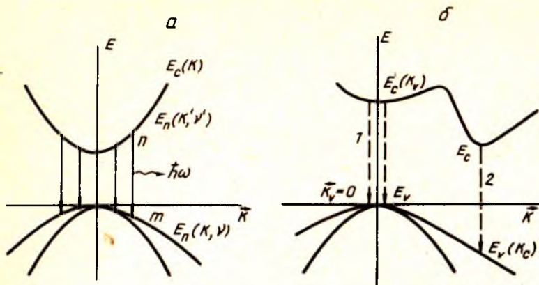
4.3- расм. а) зоналараро нурланишли рекомбинациядаги тўғри ўтишлар; б) нотўғри зонали яримўтказгичда нурланишли рекомбинациядаги тўғри ўтишлар.
