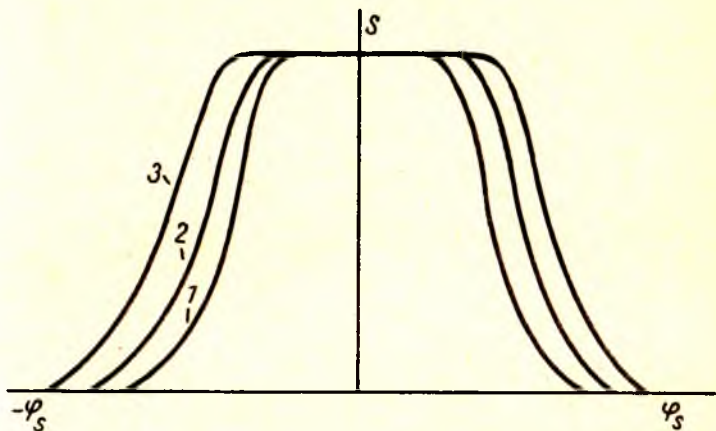
4.16- расм. E_s сатҳнинг ҳар хил қийматларида сирт рекомбинацияси тезлигининг сирт потенциалига боғланиши ( E_s(1) < E_s(2) < E_s(3) ).
