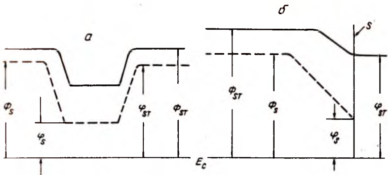
6.8- расм. Қолдиқ ўтказувчанликни тушунтирувчи нотекис жойлашган потенциал тўсиқлар модели:
