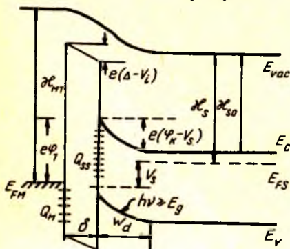
8.6- расм. МДЯ структурали куёш элементининг энергетик зоналар диаграммаси:
