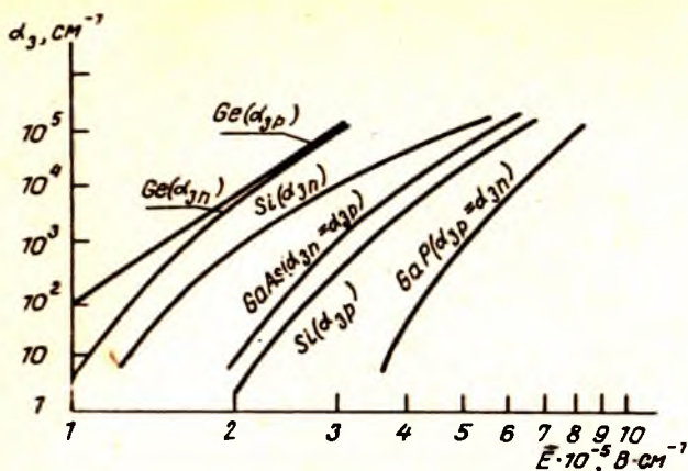
3.17- расм. Германий, кремний, галлий арсениди ва галлий фосфида зарбдан ионланиш коэффициентининг электр майдон кучланганлигига боғлиқлиги.
