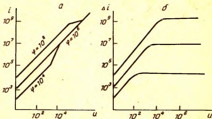
7.6- расм. Умумий ток (а) фототок (б)нинг назарий вольт-ампер характеристикаси.
