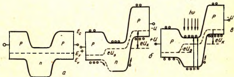
8.10- расм. Ташқи кучланиш бўлмаган (а) ва бўлган (б, в) ҳоллар учун фототранзисторнинг зонавий модели:
