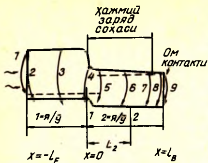
8.20- расм. Ёритилган гетероўтишда заряд ташувчиларнинг рекомбинация механизмлари.
