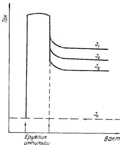
6.7- расм. Яримўтказгичда ёруғликнинг ҳар хил интенсивлигига мос келган қолдиқ ўтказувчанликлар.
