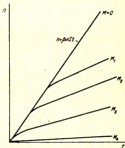
4.19- расм. Ҳар хил концентрацияли \alpha -типдаги ёпишиш маркази (сатҳи) бўлган намунада бошланғич босқичдаги релаксация ( M_1 < M_2 < M_3 < M_4 ).
