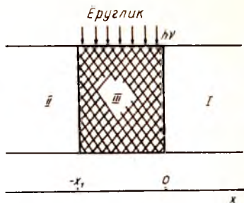
5.3- расм. Бикутбий ҳол учун намунани ёритиш схемаси.
