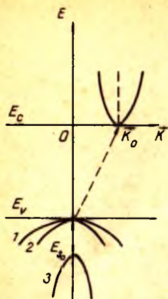
1.3- расм. Si ва Ge кристаллари зоналари тузилиши. \bar{k}_0 - E(k) функциянинг ўтказувчанлик зонаси тубини аниқлайдиган минимуми нуқтаси, валент зона шипи k=0 нуқтада, валент зонада E(\bar{k}) тармоқлари:
