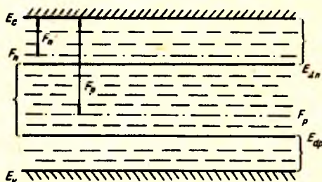
4.2- расм. Ферми квазисатҳлари ва демаркацион сатҳларнинг яримўтказгичнинг тақиқланган зонасида жойлашиши:
