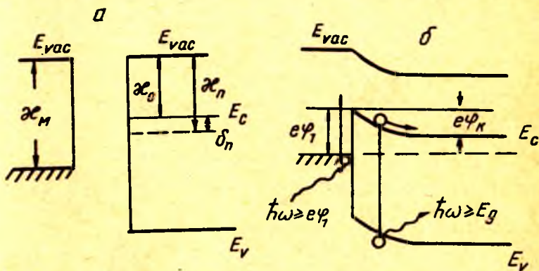
8.4- расм. Металл ва яримутказгичнинг контактлашишдан олдинги энергетик зоналар диаграммалари (а), металл ва яримутказгич контактлашганда ҳамда кучланиш бўлмаганда Шоттки потенциал тўсиғининг пайдо бўлиши (б).
