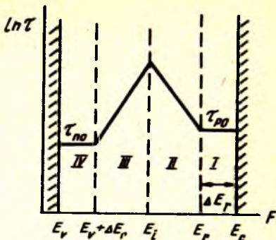
4.10- расм. Заряд ташувчилар яшаш вақтининг тақиқланган зонадаги Ферми сатҳига боғлиқлиги.
