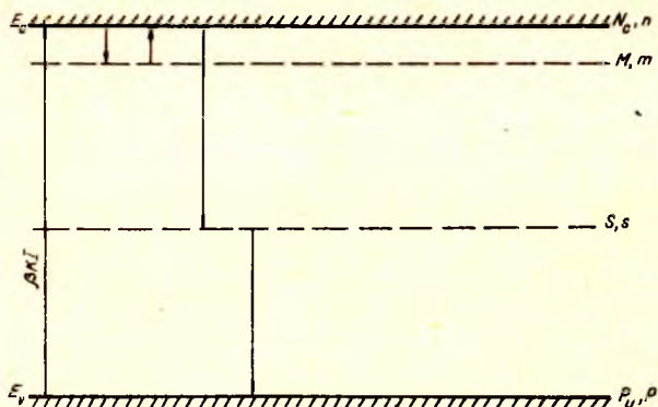
4.18- расм. Биттадан рекомбинация ( S ) ва ёпишиш ( M ) марказлари бўлган яримўтказгичда электрон ўтишлар схемаси.
