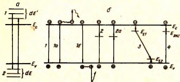
4.1- расм. E_c + dE' ва E_v + dE тўплам ҳолатлар орасидаги (а) ва ҳар хил рекомбинация механизмлари ҳолларида (б) электрон ўтишлар:
