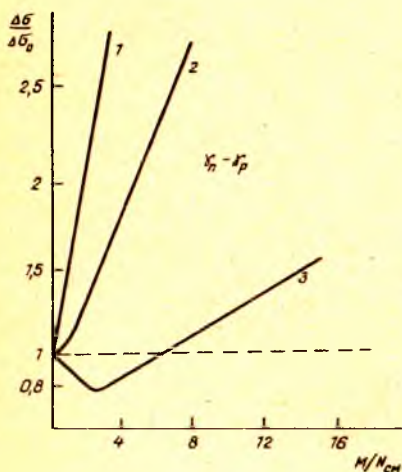
4.21- расм. Стационар фотоўтказувчанликнинг ёпишиш марказлари (сатҳлари) мавжуд бўлган ҳолда
