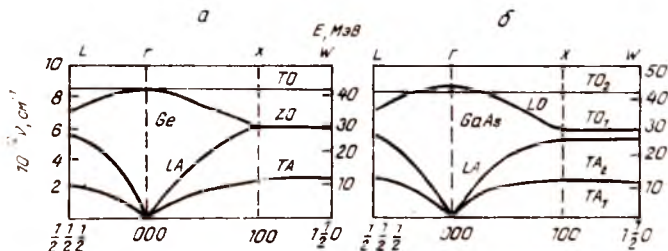
3.13- расм. Уч кристаллографик йўналишда германий (а) ва галлий арсениди (б) учун ҳисобланган фонон спектри.
