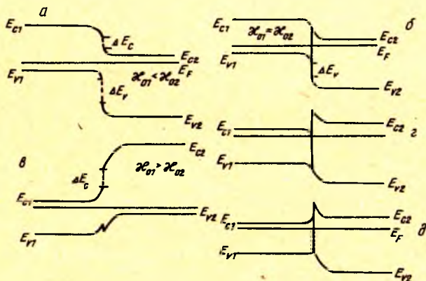
8.16- расм. x_{01} < x_{02} (а), x_{01} = x_{02} (б), x_{01} > x_{02} (в) бўлган ҳоллардаги p - n - гетероўтишнинг, бенуксон (г) ва акцептор чегаравий ҳолатлар (д) бўлгандаги p - n - гетероўтишнинг энергетик зоналар диаграммалари.
