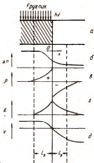
5.2-расм. Қисман ёритилган монокутбий ўтказувчанликни намуна (а) да номувозанат ҳолатдаги эркин заряд ташувчилар (б), ҳажмий заряд (в), электр майдон (г) ва потенциал (д) тақсимооти.
