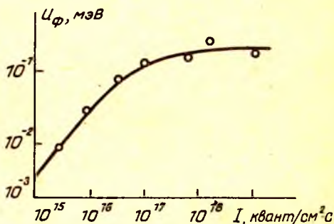
7.8- расм. Германийда фотомагнитик ЭЮКнинг ёруғлик интенсивлигига боғлиқлиги.
