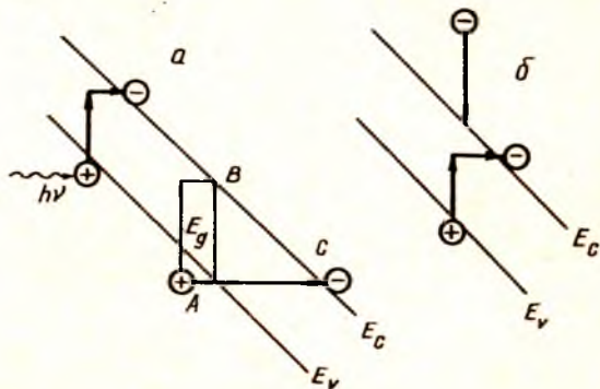
3.18- расм. Франц-Кельдиш эффектида электрон ўтишлар схемаси:
