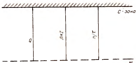
5.1- расм. Монокутбий ўтказувчанликда электрон ўтишлар схемаси.
