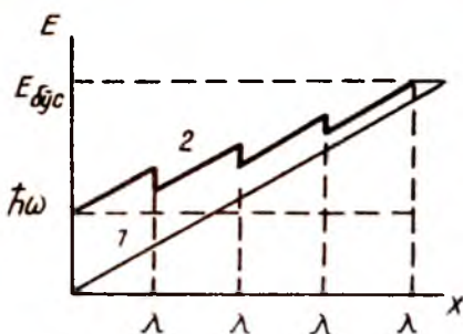
3.14-рasm. Зарбдан ионланишнинг шартли диаграммаси:
