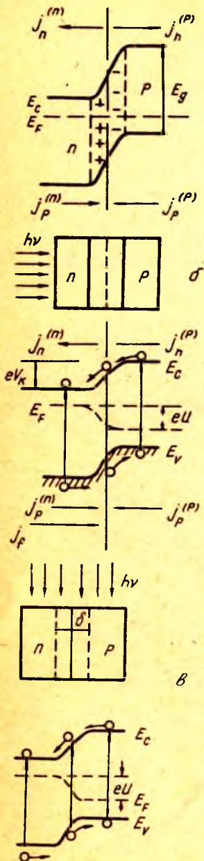
8.1-расм. p - n -ўтишнинг энергетик схемаси:
