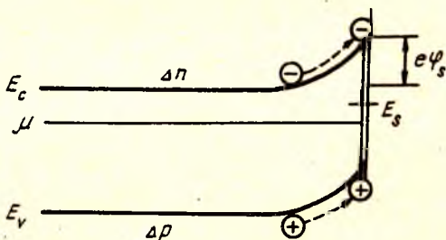
4.15- расм. Сирт ҳолатлари ( E_s сатҳлар) орқали кечадиган рекомбинация.
