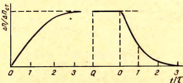
2.1- расм. Нормуванатий заряд ташувчилар релаксацияси:
