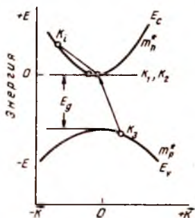
3.15- расм. Ўтказувчан ва валент зоналарнинг иккаласи ҳам параболик зоналардан иборат бўлган яримўтказгичда зарбдан ионланиш ҳодисаси схемаси ( E_{бўс} — электрон бошланғич ҳолати энергияси, \vec{k}_i — тўлқин вектор).
