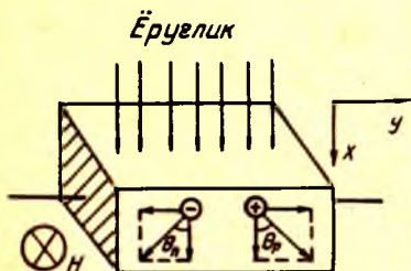
7.7- расм. Фотомагнит электр юритувчи куч (ЭЮК) нинг пайдо бўлишини тушунтиришга оид чизма (магнит майдон чизма текислигига тик йўналган).
