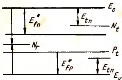
4.23- расм. Рекомбинация марказининг бир тури ва электрон, коваклар туткичи бўлганда яримўтказгичнинг зонали тузилиши.
