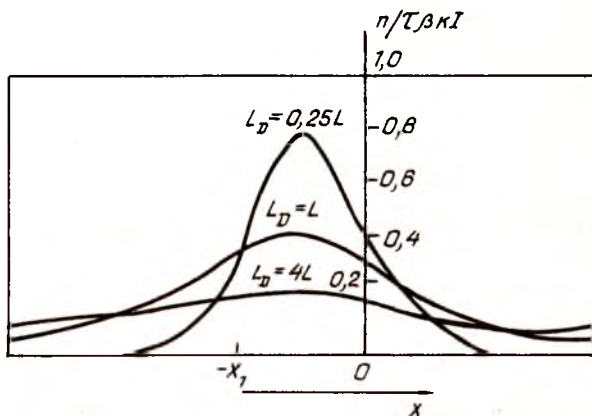
5.4- расм. Бикутбый ҳолда электр майдон бўлмаганда ( \vec{E}=0 ) номувозанат ҳолатдаги заряд ташувчиларнинг тақсимооти
