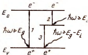
7.1- расм. Ёруғликнинг яримўтказгичда хусусий (1) ва киришмавий (2,3) ютилиши.
