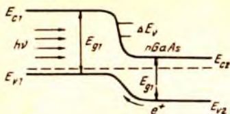
8.22- расм. p\text{Al}_x\text{Ge}_{1-x}\text{As} - n\text{GaAs} гетероўтишнинг энергетик зоналар диаграммаси.
