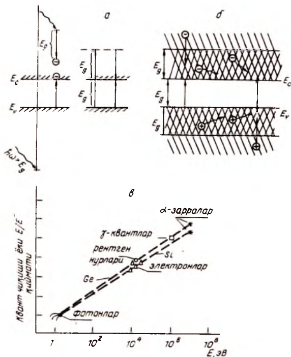
3.12- расм. Энергияси тақикланган зонадан катта бўлган фотон ютилишидаги электрон ўтишлар (а), энергияси катта бўлган заррачалар, квантлар билан ионланишда электрон-ковак жуфтini ҳосил қилиш энергиясининг тақикланган зона кенглигидан катта бўлиши (б). фотоионланишда квант чиқишининг энергияга боғлиқлиги (в).
