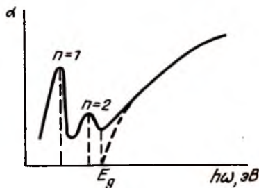
3.6- расм. Тўғри зонали яримўтказгичда ёруғликнинг экситоний ютилиш спектри.
