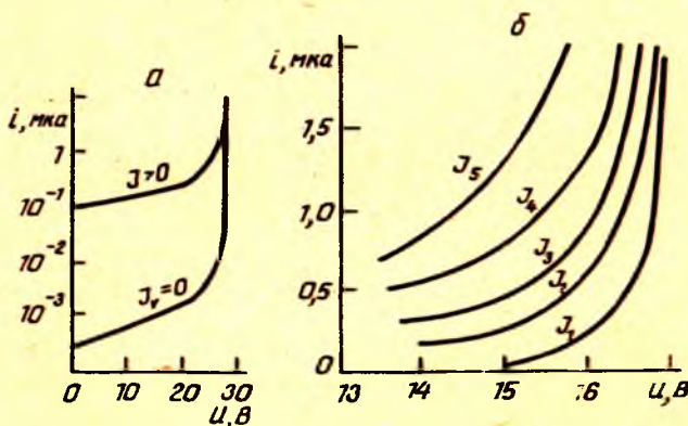
8.8- расм. Кремнийдан (а), германийдан (б) ясалган кўчкили-учма фотодиодларнинг ёруғликнинг ҳар хил интенсивлигида олинган вольт-ампер характеристикалари ( I_5 > I_4 > I_3 > I_2 > I_1 ; I_5/I_2 = 10^2 ).
