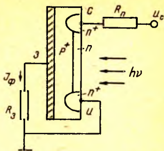
8.12- расм. Майдоний фототранзисторнинг тузилиши.
