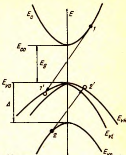
4.8- расм. Валент зонаси тармоқ- ларга парчаланган яримўтказгич- даги зоналараро Оже-рекомбина- ция жараёни схемаси.
