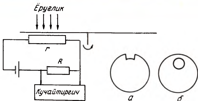
7.5- расм. Фотоўтказувчанликни ёруғлик окимини модуляциялаш (узиб-узиб ёритиш) усули билан ўлчаш:
