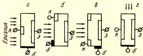
8.9- расм. Фототранзисторларнинг тузилиш схемаси.
