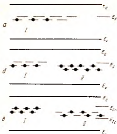
6.1- расм. Яримўтказгичнинг ёруғликка сезгирлигини оширишни тушунтириш модели:
