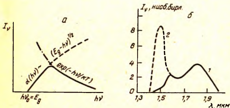
4.5- расм. Тўғри зонали яримўтказгичда зоналараро нурланиш рекомбинациясининг нурланиш спектри (а) ҳамда германийда зоналараро рекомбинация нурланишининг спектри (б):
