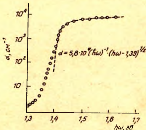
3.1-расм. Уй температурасида GaAs кристаллида хусусий ютилиш коэффиценти билан фотон энергияси орасидаги боғланиш (узлукли чизик — назарияга, нуқтали чизик — тажриба натижасига тааллуқли).
