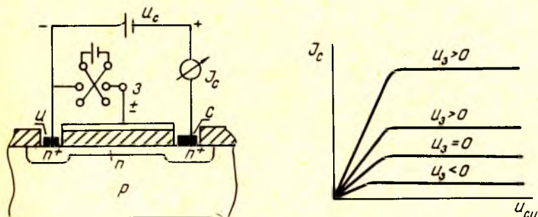
8.14- расм. Ташқи кучланиш қўйилган n - каналли МДЯ- транзистор (а), унинг вольт-ампер характеристикаси (б) ( I_c \sim U_g соҳа триод режими, I_c = \text{const} соҳа тўйиниш режими деб аталади).
