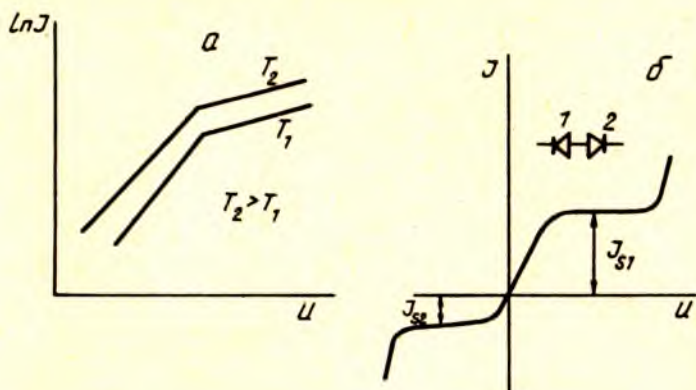
8.19- расм. Кескин анизотибли гетероўтишнинг (а) ва изотибли n - n гетероўтишнинг (б) вольт-ампер характеристикалари.
