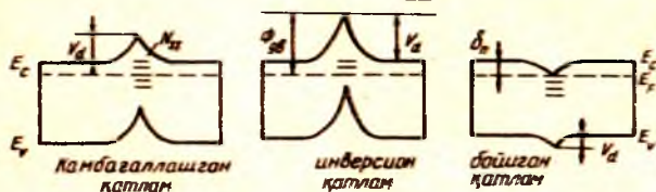
8.24- расм. Кристаллчалар чегарасидаги уч хил потенциал тўсиқ.
