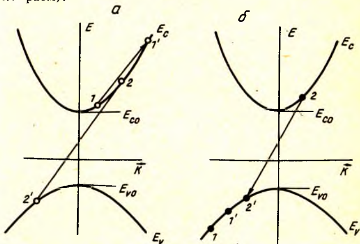
4.7- расм. Ўтказувчан ва валент зоналарнинг параболик моделидаги зоналаро зарбдан рекомбинацияланиш жараёни схемаси:
