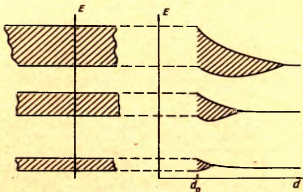
1.1- расм. Якка атомдаги электроннинг энергетик сатҳларидан кристаллдаги электронлар энергетик зоналари ҳосил бўлиши: d — қўшни атомлар ораллиги, d_0 — кристаллдаги қўшни атомлар ораллиги.
