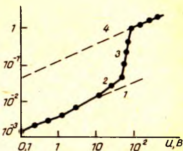
8.27- расм. Полистерен биндерига қўшилган \text{CdS} : \text{Cu} : \text{Cl} кукунда фототокнинг кучланишга боғлиқлиги.
