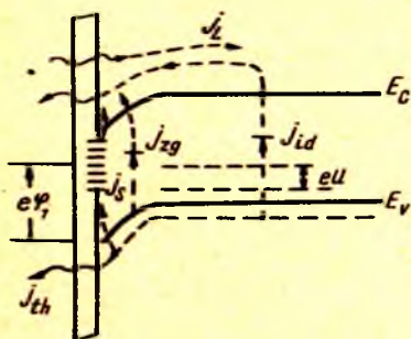
8.5- расм. n-тип кремний асосидаги МДЯ структурасида токнинг ҳар хил ташкил этувчиларининг йўналиши схемаси.
