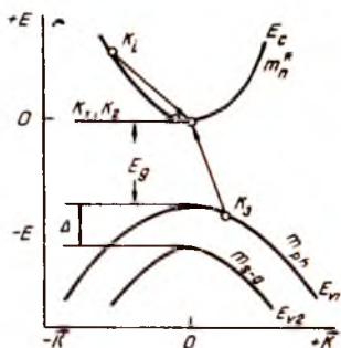
3.16- расм. Энергетик зоналар структураси ва электрон энергияси ионланишнинг бўсағавий энергиясига етганда зарбдан ионланиш ҳодисаси.
