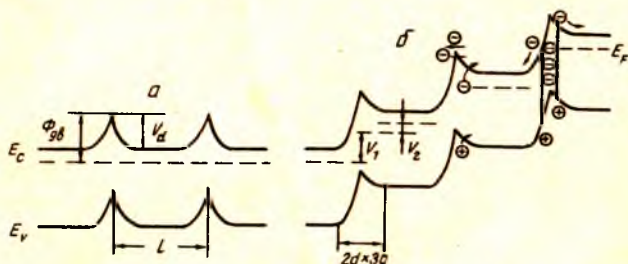
8.26- расм. Доналари орасида потенциал тўсиқ бўлган поликристалл материалларнинг бир ўлчовли зоналар модели:
