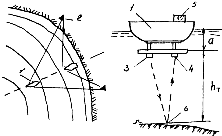
2.7-rasm. Exolot yordamida chuqurliklarni o'lchash:
