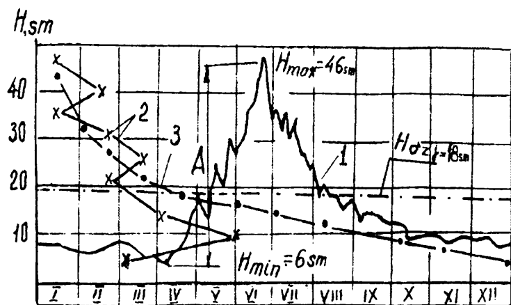
2.4-rasm. Suv sathining yillik grafigi:
