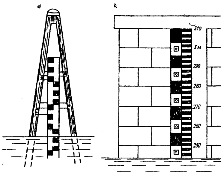
2.1-rasm. Reykali postlar:
