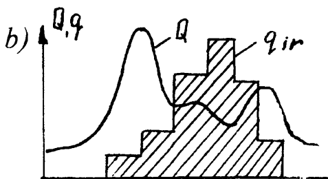
3.7. (b)-rasm. Oqimni murakkab rostlash gidrografi
