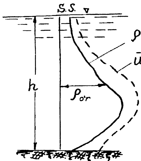
2.27-rasm. Oqiziqalarni chuqurlik bo'yicha taqsimlanishi: 1 – loyqalik epyurasi; 2 – gidravlik yiriklikgi epyurasi
