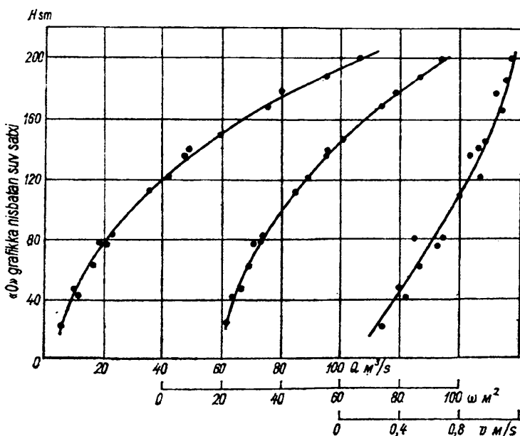
2.25-rasm. Suv sarfi, oqim jonli kesimi yuzasi va o'rtacha tezliklari egri chiziqlari
