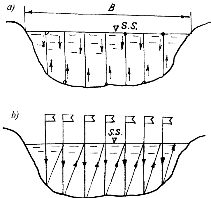
2.20-rasm. Integratsiya usuli bo'yicha oqim tezliklarini o'lchash a – vertushkani vertikkallar bo'yicha harakatlantirib tezlikni o'lchash; b – vertushkani oqim ko'ndalang kesim bo'yicha harakatlantirish; → – vertushkaning tezlik o'lchash mobaynida harakat yo'nalishi
