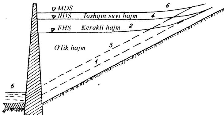
3.9-rasm. Suv omborining asosiy sathlari va hajmlari
