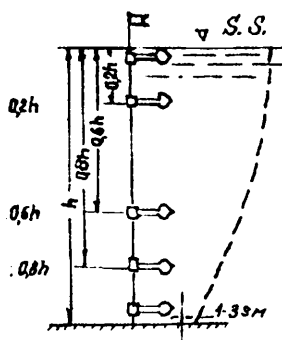
2.19-rasm. Batafsil usul bilan suvning o'rtacha tezligini aniqlash
