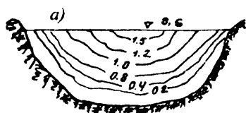
2.13-rasm. Izotaxa chiziqlarining ko'rinishi (a – ochiq havzada; b – muz ostida)
