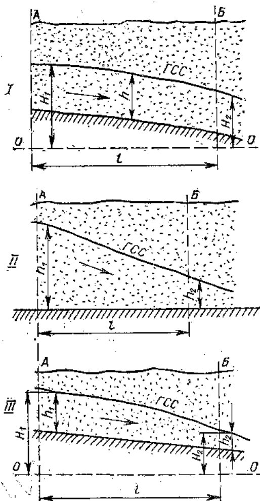
16.6- rasm. Grunt suvlari oqimining sarfini hisoblash sxemasi: I va II - suv o'tkazmaydigan qatlamning gorizontal vaziyati; III - qiya vaziyati
