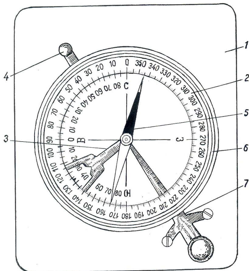
12.5-rasm. Tog' kompassi.
