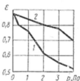
14.13-rasm. Oldindan ivitilgan (1) va tabiiy namlikdagi (2) lyossimon tog' jinsining zichlanish grafigi
