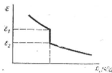
14.14-rasm. Lyossimon tog' jinsining zichlanishini ifodalovchi egri chiziq.
