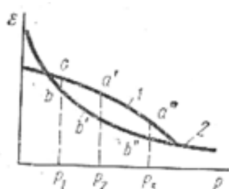
14.12-rasm. Suvga to'la to'yingan va tabiiy namlikdagi lyossimon jinslarning zichlanish grafigi .
