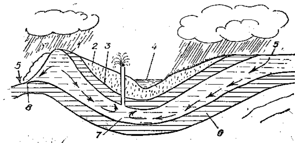
16.4 - rasm. Ateziyan havzaning qirqimi: 1- suv o'tkazmaydigan qatlam. 2-tuproq suvi, 3-grunt suvi, 4-daryo, 5- buloq, 6-qatlamlar orasidagi pastga tushuvchi yer osti suvi, 7-qatlamlar orasidagi ko'tariluvchi yer osti suvi, 8-suv o'tkazmaydigan qatlam
