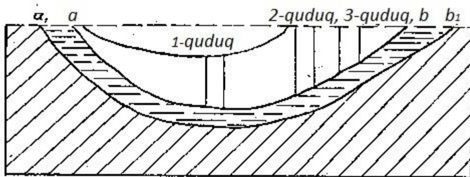
16.1 - rasm. Artezian suvining yer yuzasiga chiqishi. Yoy (mul'dasimon) shaklda bosimli suvli gorizontning yotishi, a_1a va bb_1 – suvli gorizontning yer yuzasiga chiqishi.
