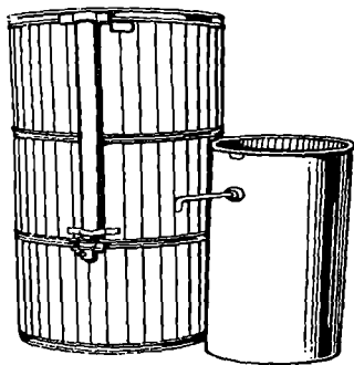
24-rasm. Ksilometrlar: chapda — o'zgaruvchan suv sathi bilan; o'ngda — o'zgarmas suv sathi bilan.
