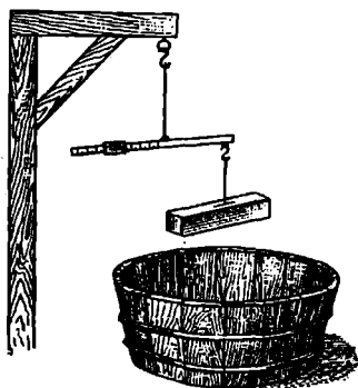
25-rasm. Oddiy gidrostatik tarozi.
