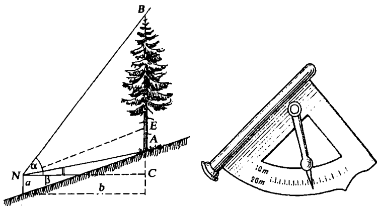
16-rasm. Daraxt balandligini Makarov ish qurolida o'lchash.
