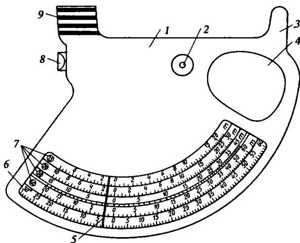
7-rasm. Blyume-Leyssanining daraxtlar balandlik o'lchagichi.
