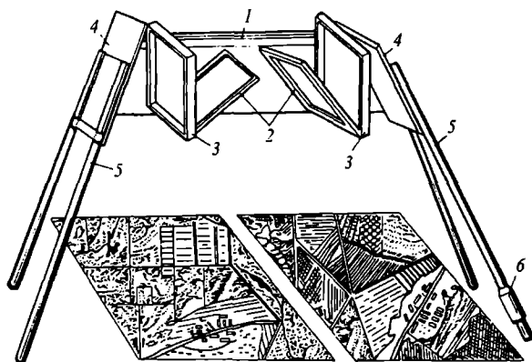
54-rasm. Oynali – linzali stereoskop:
