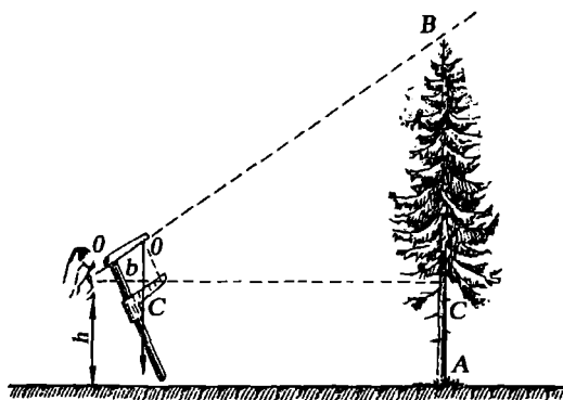
15-rasm. Daraxt balandligini qo'zg'aluvchi chizg'ich yordamida o'lchash (mernaya vilka).
