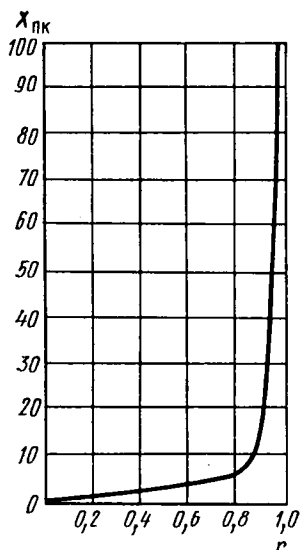
Рис. 15.6. Зависимость степени полимеризации ( \bar{x}_{\text{пк}} ) от коэффициента эквивалентности ( r )
