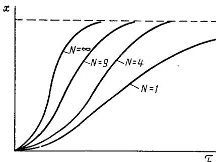
Рис. 3.15. Влияние на степень превращения числа реакторов N в каскаде
