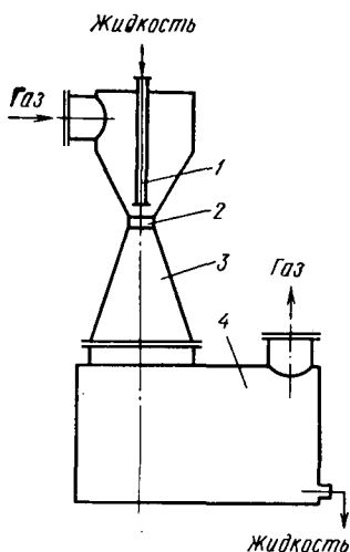
Рис. 3.11. Реактор полного смешения — абсорбер Вентури:
