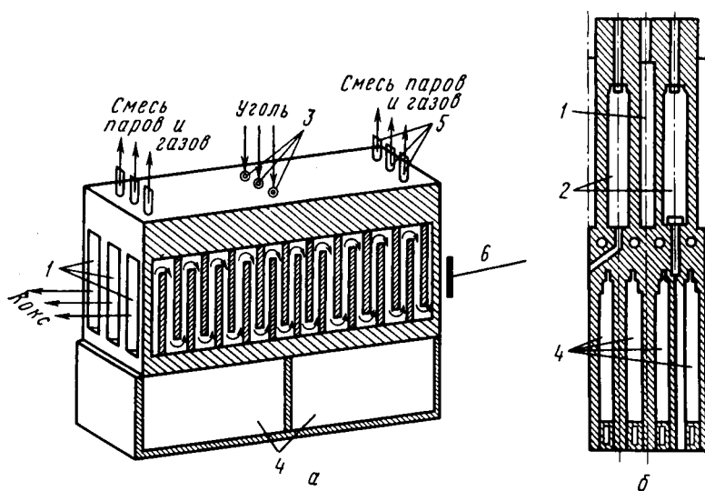
Рис. 9.15. Коксовая печь:
