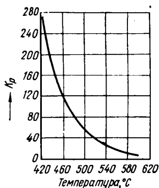
Рис. 11.4. Зависимость константы равновесия K_1 от температуры при нормальном давлении
