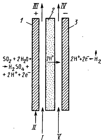
Рис. 13.3. Схема электрохимической стадии комбинированной системы производства водорода:
