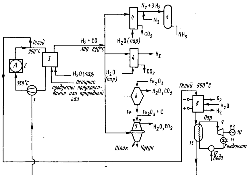
Рис. 9.5. Принцип создания энерготехнологических систем с включением атомного реактора:
