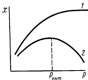
Рис. 2.9. Зависимость выхода продукта от давления для обратимой газовой реакции ( \tau, t, c_A, c_B = \text{const} ): 1 — \Delta n < 0 ; 2 — \Delta n > 0
