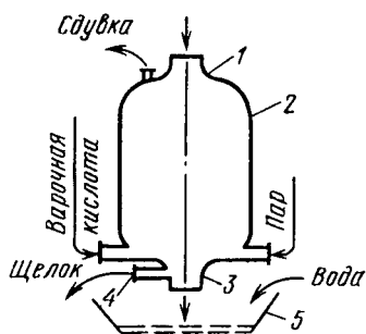
Рис. 15.7. Схема котла для варки целлюлозы:
