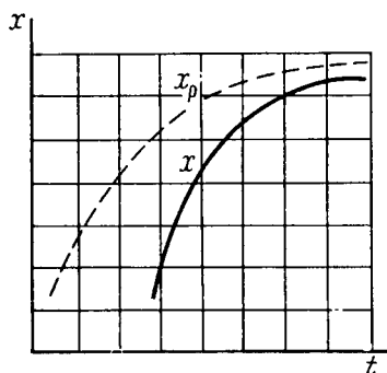
Рис. 2.13. Зависимость выхода продукта от температуры для эндотермических обратимых реакций ( t, P, c_A, c_B = \text{const} )
