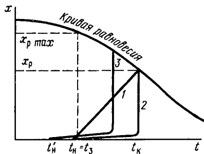
Рис. 3.19. Сравнение режимов адиабатических реакторов вытеснения и изотермических реакторов смешения:
