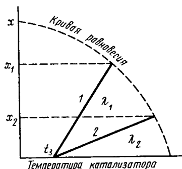
Рис. 5.7. Влияние адиабатического коэффициента \lambda на выход продукта для однослойного аппарата без теплообмена
