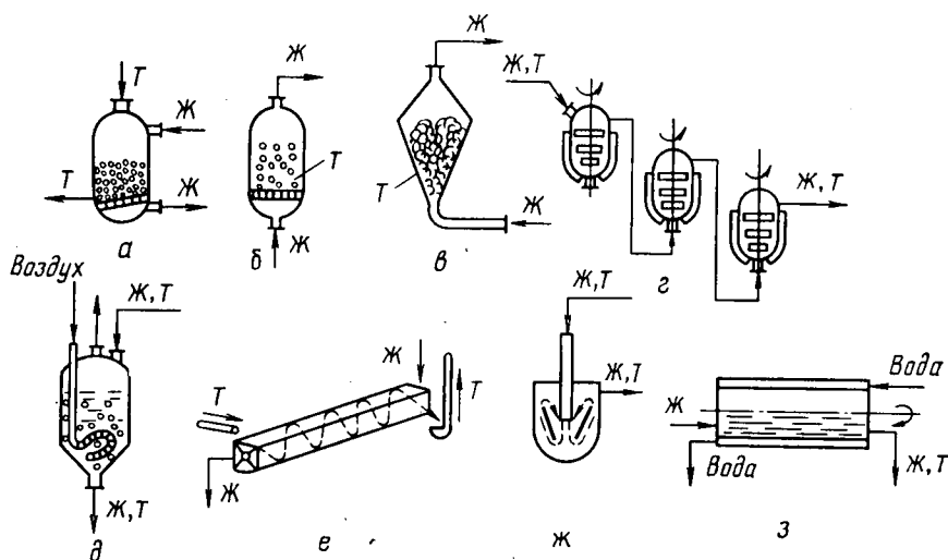
Рис. 4.20. Типы реакторов для процессов с участием твердых и жидких реагентов (Т—Ж):
