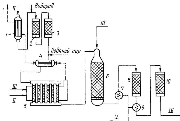
Рис. 9.20. Энерготехнологическая схема конверсии метана природного газа:
