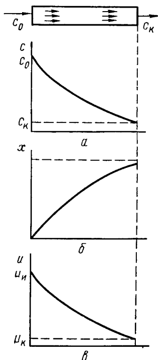
Рис. 3.5. Изменение концентрации реагентов (а), степени превращения (б) и скорости реакции (в) в реакторе идеального вытеснения
