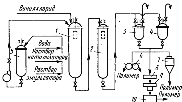
Рис. 15.17. Схема установки для производства поливинилхлорида непрерывным эмульсионным способом:
