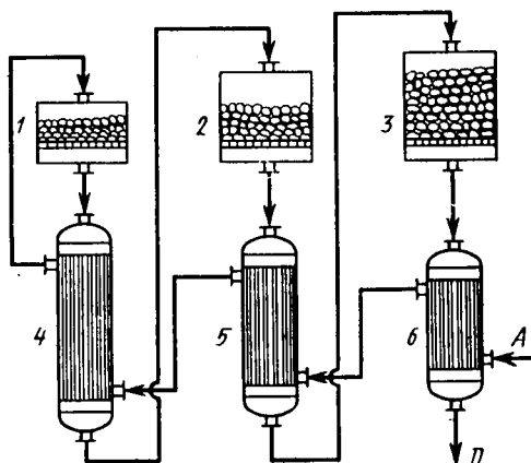
Рис. 5.8. Система контактных аппаратов с внешними теплообменниками:
