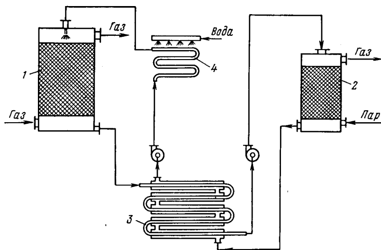
Рис. 8.11. Схема установки для абсорбционно-десорбционного метода разделения газов:
