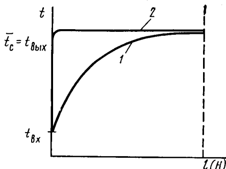
Рис. 3.20. Характер изменения температуры по длине (высоте) реактора идеального вытеснения (1) и полного перемешивания (2) при осуществлении экзотермических процессов без теплообмена
