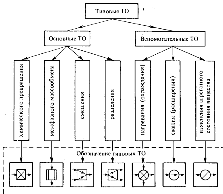
Рис. 6.2. Классификация типовых технологических операторов
