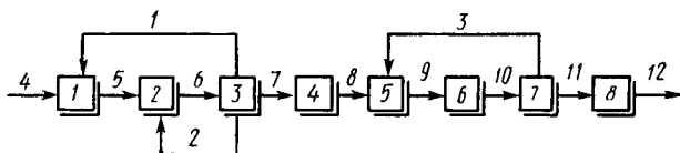
Рис. 6.11. Замкнутая схема
