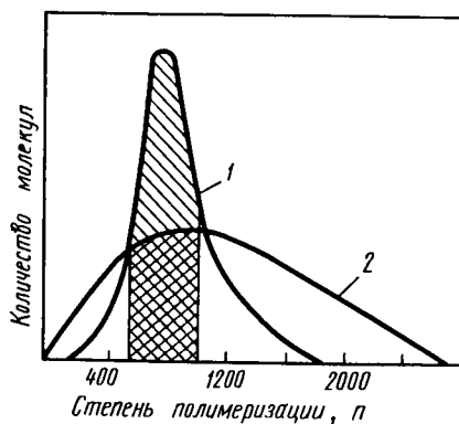
Рис. 15.1. Распределение молекул по степени полимеризации: 1 — нитроцеллюлоза; 2 — полистирол
