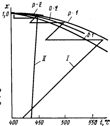
Рис. 11.6. Диаграмма x-t для пятислойного аппарата системы ДК с промежуточным теплообменом и абсорбцией \text{SO}_3 после третьего слоя:
