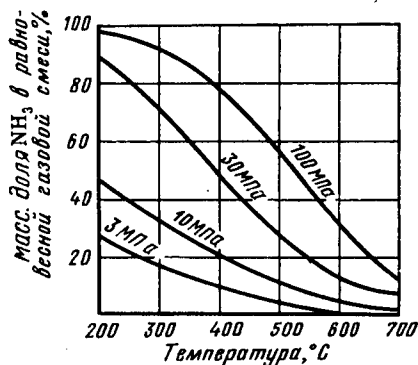
Рис. 10.2. Зависимость равновесного выхода аммиака от температуры для различных давлений
