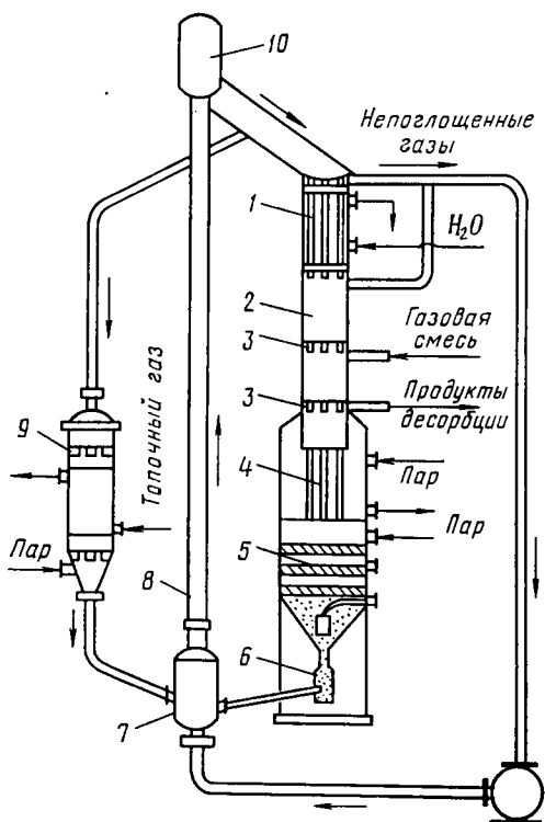
Рис. 7.7. Адсорбер с движущимся слоем сорбента:
