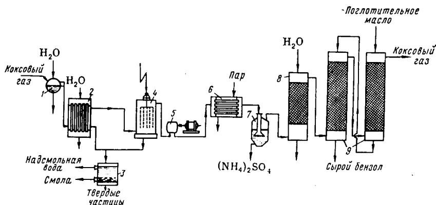
Рис. 9.17. Схема переработки прямого коксового газа:
