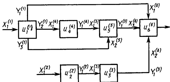
Рис. 6.10. Разомкнутая схема:
