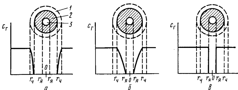
Рис. 4.12. Изменение концентрации газообразного реагента c_r в ходе взаимодействия со сферической твердой частицей: 1 — газовая ламинарная пленка; 2 — слой продуктов реакции; 3 — непрореагировавшее ядро. Лимитирующие стадии: а — внешняя диффузия; б — внутренняя диффузия; в — химическая реакция
