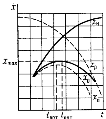
Рис. 2.12. Зависимость выхода продукта от температуры для экзотермических процессов ( \tau, P, c_A, c_B = \text{const} ):
