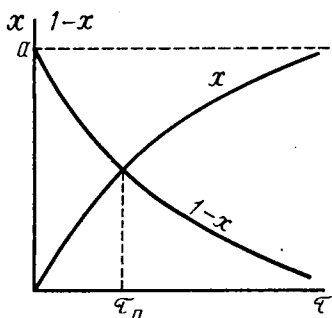
Рис. 4.1. Зависимость выхода продукта x и количества оставшегося вещества (1-x) от времени для необратимой реакции первого порядка
