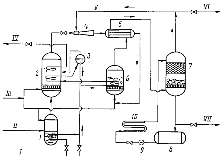
Рис. 8.1. Рециркуляционная энерготехнологическая система производства серной кислоты:
