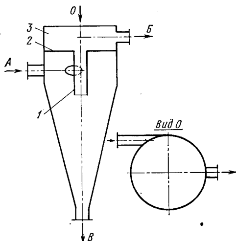
Рис. 7.2. Схема гидроциклона:
