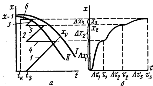
Рис. 5.9. Зависимость степени превращения от температуры (а) и от времени (б) для трехступенчатого контактирования (по рис. 5.8):
