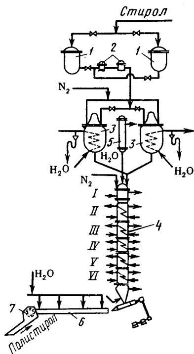
Рис. 15.16. Схема установки для непрерывной полимеризации стирола в массе:
