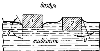
Рис. 7.4. Влияние смачивания
