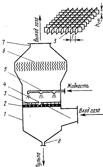
Рис. 4.11. Пенный аппарат: 1 — корпус; 2 — решетка; 3 — стабилизатор пены; 4 — вход газа; 5 — подача жидкости; 6 — брызгоуловитель; 7 — выход газа; 8 — выход пульпы
