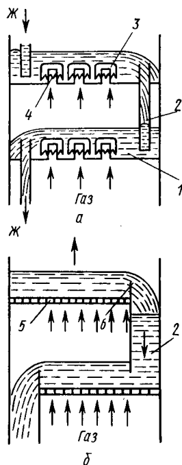
Рис. 4.9. Схема устройства барботажного реактора с внутренними переливами (а) и ситчатыми тарелками (б): 1 — колпачковая тарелка; 2 — переливная труба; 3 — колпачок; 4 — патрубок для газа; 5 — ситчатая тарелка (решетка); 6 — сливной порог
