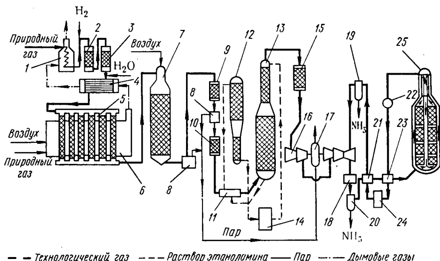
Рис. 10.6. Принципиальная схема синтеза аммиака под средним давлением:
