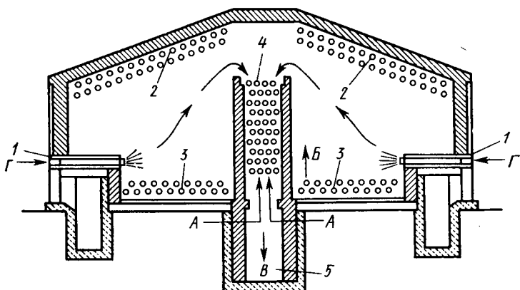
Рис. 9.7. Двухкамерная трубчатая печь с наклонным сводом:
