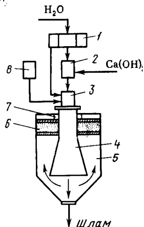
Рис. 7.9. Схема известково-содового способа умягчения воды:
