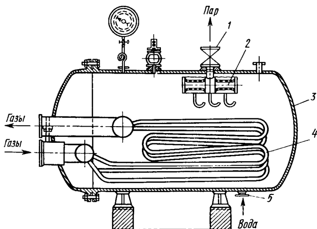
Рис. 9.3. Котел-утилизатор:
