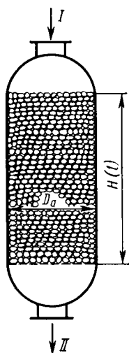
Рис. 5.6. Каталитический реактор (конвертор) шахтного типа с режимом работы, близким к идеальному вытеснению (при H > D_0 )
