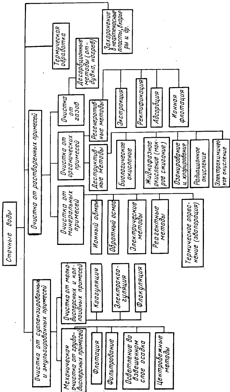
Рис. 8.2. Классификация основных методов очистки сточных вод химических производств
