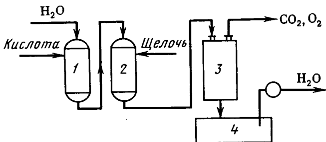
Рис. 7.10. Схема установки для обессоливания воды ионитами:
