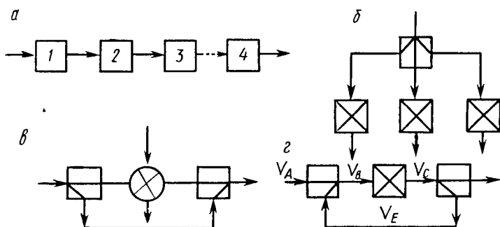
Рис. 6.4. Типы технологических связей:
