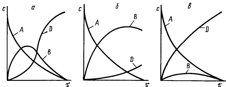
Рис. 2.3. Изменение концентрации в последовательных необратимых реакциях A \xrightarrow{k_1} B \xrightarrow{k_2} D a - k_1 \simeq k_2 ; б - k_1 \gg k_2 ; в - k_1 \ll k_2
