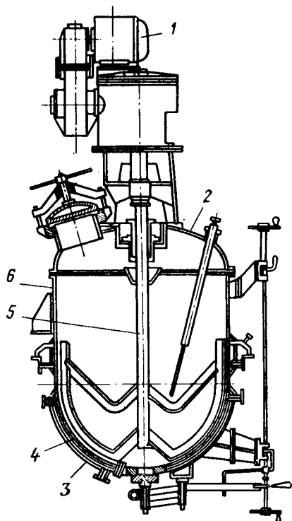
Рис. 15.18. Схема реактора для получения поликонденсационных смол:
