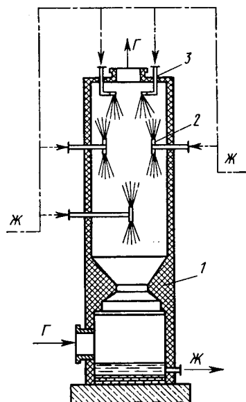
Рис. 4.10. Полая башня с разбрызгиванием жидкости: 1 — корпус; 2 — двойной распылитель жидкости; 3 — одинарный распылитель жидкости
