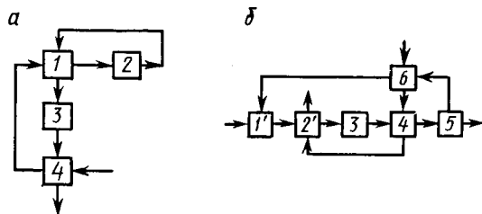
Рис. 6.5. Замкнутая ХТС:
