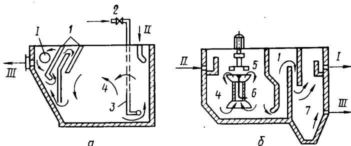
Рис. 8.7. Схема аэротенков-смесителей с пневматической аэрацией (а) и с механической аэрацией (б):
