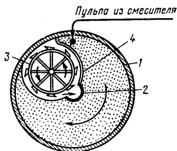
Рис. 12.3. Суперфосфатная камера непрерывного действия (план):
