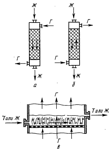
Рис. 2.6. Направление движения потоков в двухфазной системе Г—Ж:
