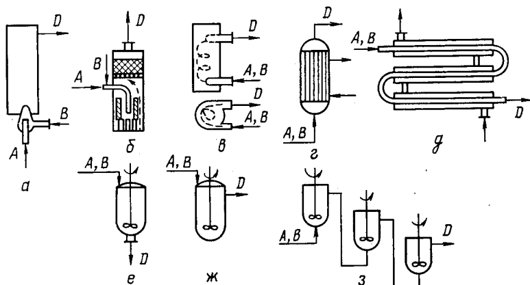
a, б — камерные реакторы с горелками ( a — режим идеального вытеснения; б — промежуточный); в — камерный реактор с сильным перемешиванием, изотермический; г, д — трубчатые реакторы вытеснения, политермического режима; е, з — реакторы с мешалками, режим полного смешения ( е — одиночный периодического действия; ж — одиночный непрерывного действия; з — каскад реакторов); A, B — исходные реагенты; D — продукты реакции
