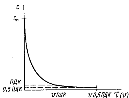
Рис. 1.1. Снижение концентрации поглощаемого компонента в необратимом процессе
