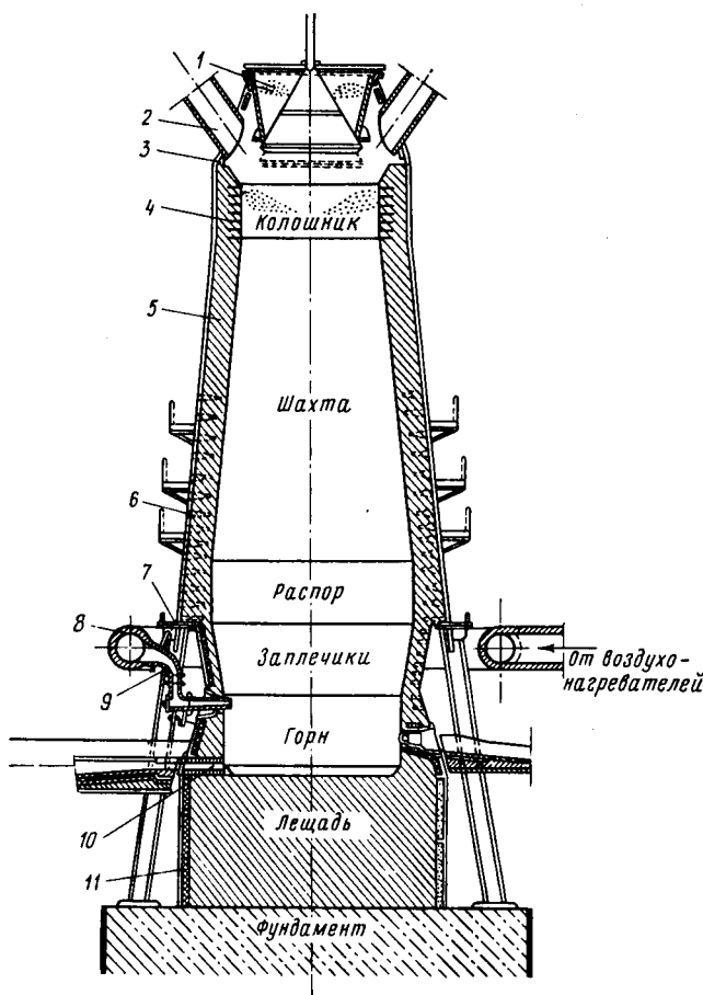
Рис. 4.15. Доменная печь:
