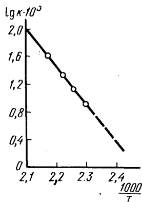
Рис. 15.4. Зависимость константы скорости поликонденсации гексаметилендиамина с себаценовой кислотой ( E=100 кДж/моль) от температуры
