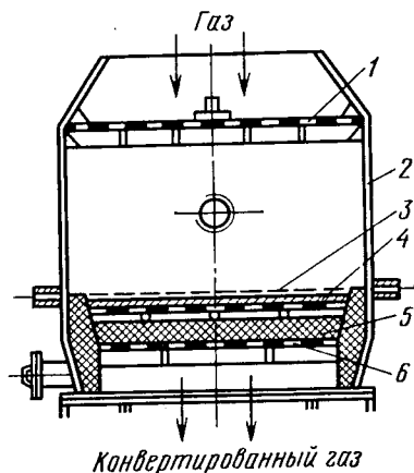
Рис. 10.10. Контактный аппарат:
