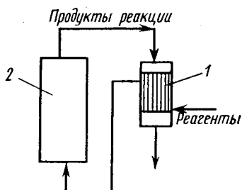
Рис. 9.1. Принцип рекуперации теплоты продуктов реакции или отходящих газов:
