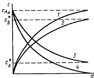
Рис. 2.1. Типичные кривые изменения концентраций реагентов во времени для простых реакций типа A \rightarrow D в реакторах вытеснения:
