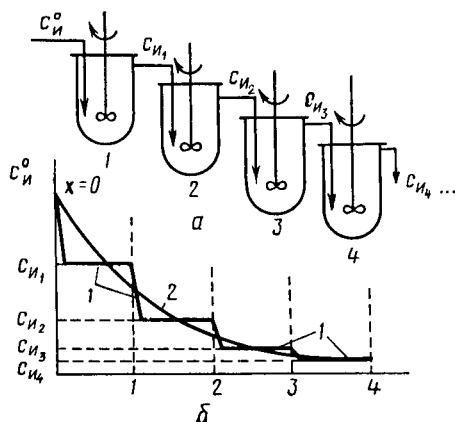
Рис. 3.14. Каскад реакторов смешения:
