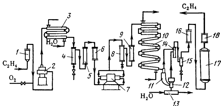
Рис. 15.15. Схема установки для получения полиэтилена непрерывным методом при высоком давлении:
