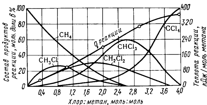
Рис. 14.8. Зависимость состава продуктов хлорирования и теплоты реакции от молярного соотношения хлора к метану
