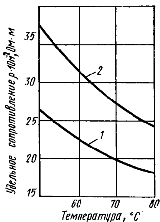
Рис. 13.1. Зависимость удельного сопротивления щелочного электролита от температуры:
