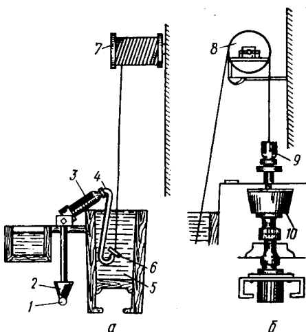
Рис. 15.11. Схема прядения:
