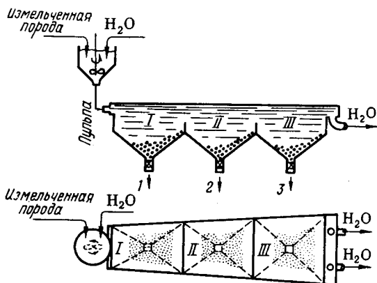
Рис. 7.1. Принципиальная схема мокрого гравитационного обогащения:
