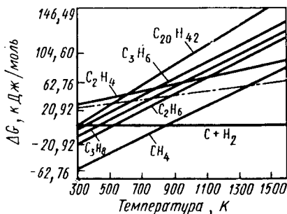
Рис. 9.10. Зависимость свободной энергии образования углеводородов (на 1 моль C) от температуры
