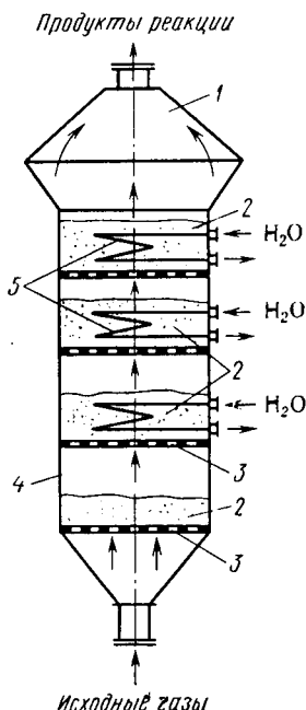
Рис. 5.13. Многослойный контактный аппарат с кипящими слоями катализатора:
