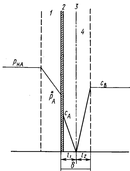
Рис. 4.6. Схема распределения концентраций в системе Г—Ж для модельной реакции A_r + B_{ж} \rightarrow D_{ж} , при высокой скорости химической реакции в жидкой фазе:
