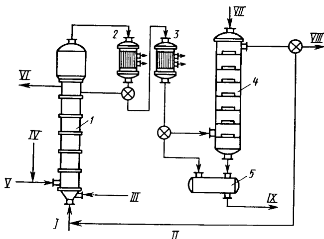
Рис. 14.15. Схема получения ацетальдегида гидратацией ацетилен в жидкой фазе:
