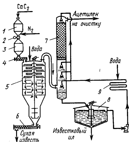
Рис. 14.12. Схема производства ацетилена из карбида кальция:
