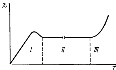
Рис. 6.16. Кривая интенсивности отказов
