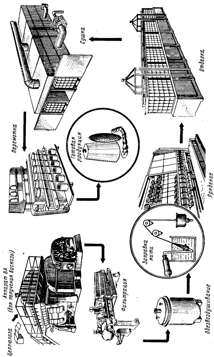
Рис. 15.10. Схема производства вискозного волокна
