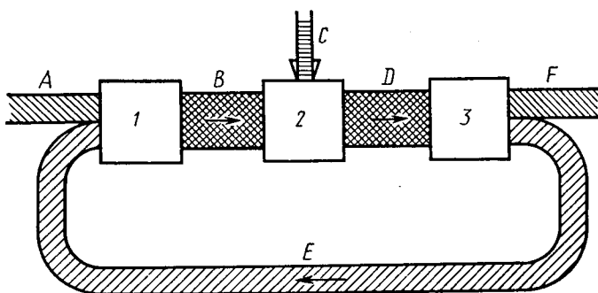
Рис. 6.14. Диаграмма материального баланса простой замкнутой ХТС
