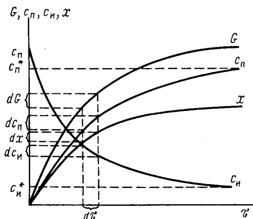
Рис. 2.5. Изменение кинетических характеристик процесса во времени для простой обратимой реакции в режиме, близком к идеальному вытеснению
