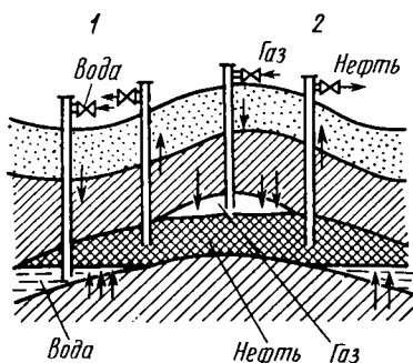
Рис. 9.6. Схема нефтедобычи путем поддержания пластового давления:
