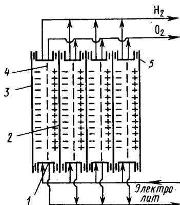
Рис. 13.2. Схема элемента биполярного фильтпрессного электролизера:
