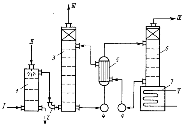
Рис. 8.12. Схема абсорбционной очистки газов от \text{CO}_2 с получением товарного диоксида углерода:
