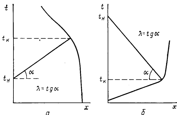
Рис. 3.16. Зависимость конечной температуры процесса t_k от степени превращения x для экзотермической (а) и эндотермической (б) реакций в адиабатическом реакторе идеального вытеснения
