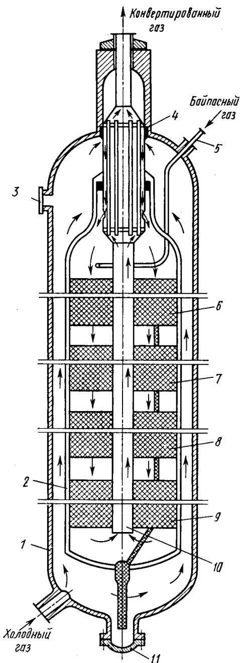
Рис. 10.7. Схема четырехполочной колонны синтеза аммиака под средним давлением:
