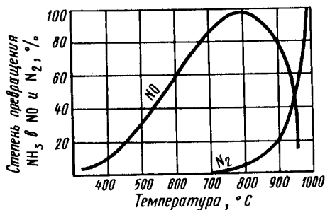
Рис. 10.8. Зависимость степени превращения аммиака от температуры ( \tau = \text{const} , катализатор \text{Pt—Pd—Rh} )
