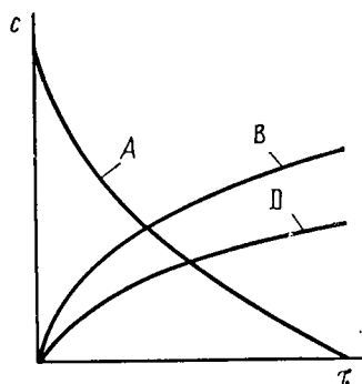
Рис. 2.2. Изменение концентраций в бинарнопараллельной необратимой реак-
