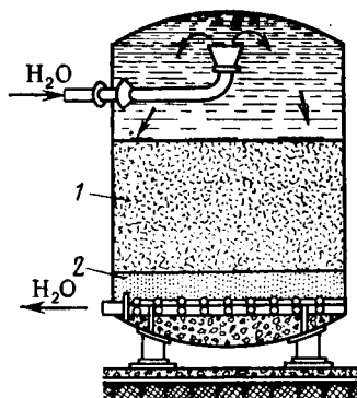
Рис. 7.11. Катионитовый фильтр:
