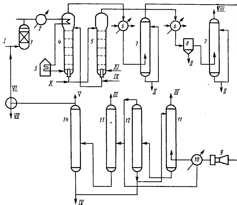
Рис. 14.7. Технологическая схема дегидрирования бутиленов:
