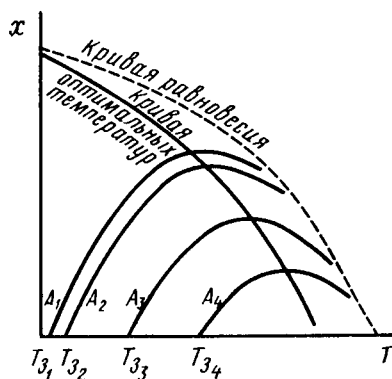
Рис. 5.4. Зависимость выхода продукта от температуры для катализаторов различной активности A_1 > A_2 > A_3 > A_4 (экзотермический процесс)
