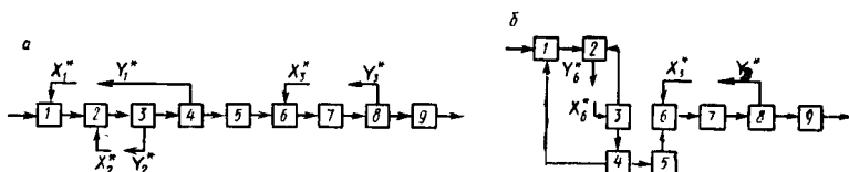
Рис. 6.12. Варианты разомкнутой схемы, соответствующей замкнутой схеме, приведенной на рис. 6.10
