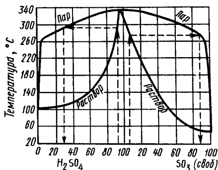
Рис. 11.2. Диаграмма кипения системы \text{H}_2\text{O} — \text{H}_2\text{SO}_4 — \text{SO}_3 при нормальном давлении
