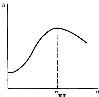
Рис. 3.12. Зависимость скорости процесса u от числа оборота мешалки в реакторе полного смешения
