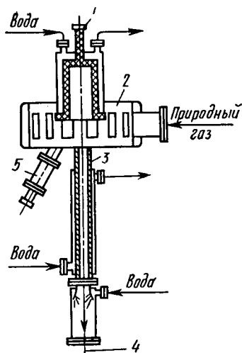
Рис. 14.13. Электродуговая печь для крекинга углеводородов:
