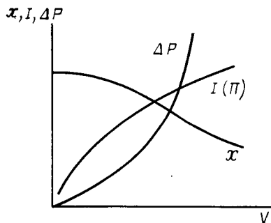
Рис. 3.4. Зависимость выхода продукта x , сопротивления аппарата \Delta P и его интенсивности I от объемной скорости V
