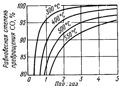
Рис. 9.19. Зависимость равновесной степени превращения оксида углерода (CO) от соотношения объемов пар: газ и температуры
