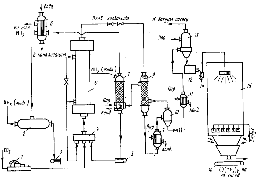
Рис. 12.8. Упрощенная схема производства мочевины с жидкостным рециклом: 1 — компрессор подачи \text{CO}_2 ; 2 — сборник жидкого аммиака; 3 — насос; 4 — смеситель; 5 — колонна синтеза; 6 — конденсатор; 7 — промывная колонна; 8 — ректификационная колонна; 9, 11 — подогреватели; 10 — сепаратор; 12 — сборник плава; 13 — вакуум-выпарной аппарат; 14 — насос подачи плава; 15 — грануляционная башня; 16 — транспортер готовой продукции
