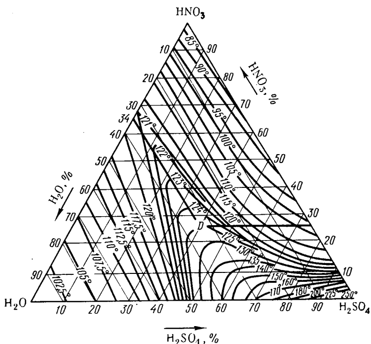
Рис. 4.5. Диаграмма фазового состояния состав — температура кипения для трехкомпонентной системы \text{H}_2\text{O} — \text{HNO}_3 — \text{H}_2\text{SO}_4
