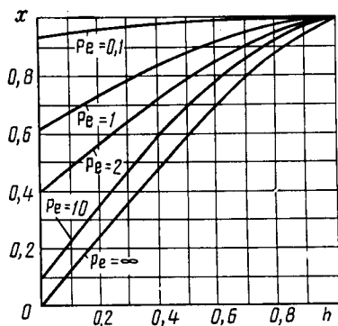
Рис. 3.21. Зависимость изменения степени превращения вещества x по высоте изотермического реактора при различных значениях критерия Pe
