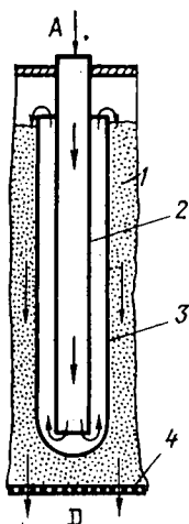
Рис. 5.11. Двойная теплообменная трубка:
