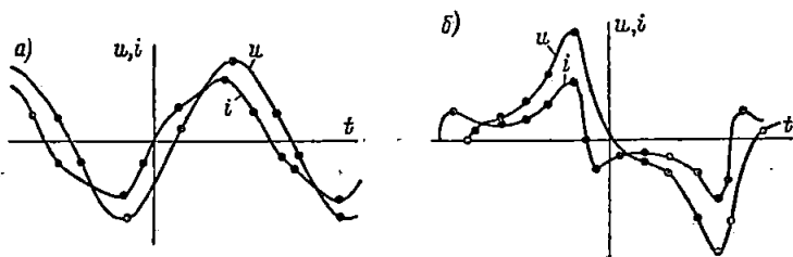
Рис. 7-5. Кривые напряжения и тока в цепи через тело человека при синусоидальном (а) и несинусоидальном (б) напряжении
