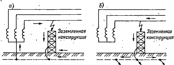
Рис. 10-1. Схема протекания тока при повреждении изоляции на территории подстанции
