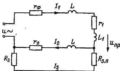
Рис. 9-4. Эквивалентная схема с двумя сосредоточенными заземлителями
