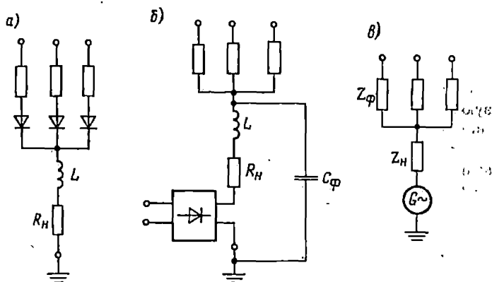
Рис. 8-5. Схемы, работающие на выпрямленных токах
