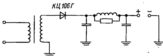
Рис. 8-2. Схема испытания изоляции электрооборудования, проводов и кабелей напряжением ниже 1000 В
