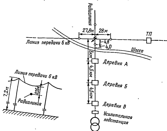
Рис. 4-8. Общая схема пересечки ЛЭП с проводами радиотрансляционной сети ТП — трансформаторная подстанция
