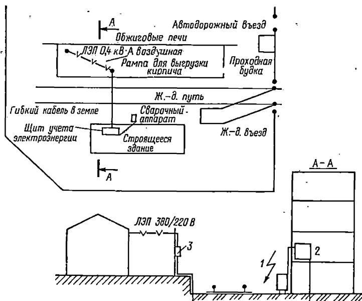
Рис. 13-1. Электрическая сеть и оборудование на месте гибели мальчика у сварочного трансформатора
