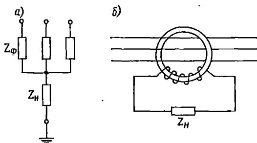
Рис. 8-4. Схема, работающая на токах нулевой последовательности
