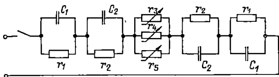
Рис. 6-8. Полная эквивалентная схема электрического сопротивления тела человека по В. Е. Мацойлову (параметры цепи — активные)
