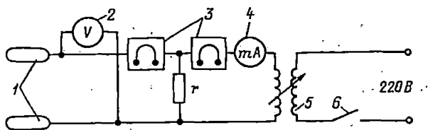
Рис. 7-6. Электрическая схема экспериментальной установки для определения пороговых значений ощутимых токов
