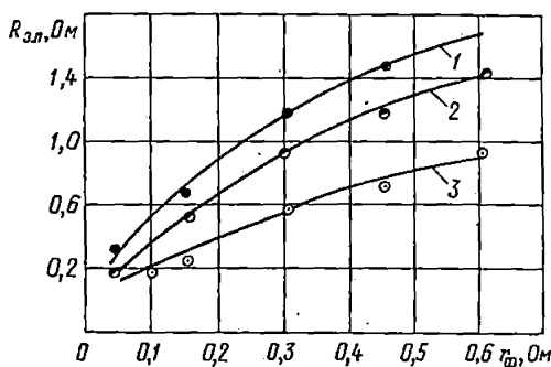
Рис. 9-7. Изменение сопротивления заземления повторного заземлителя R_{з.п} в зависимости от активного сопротивления фазного провода r_{ф} при заданных значениях прикосновения 1 — u_{пр} = 36 \text{ В} ; 2 — u_{пр} = 40 \text{ В} ; 3 — u_{пр} = 50 \text{ В}
