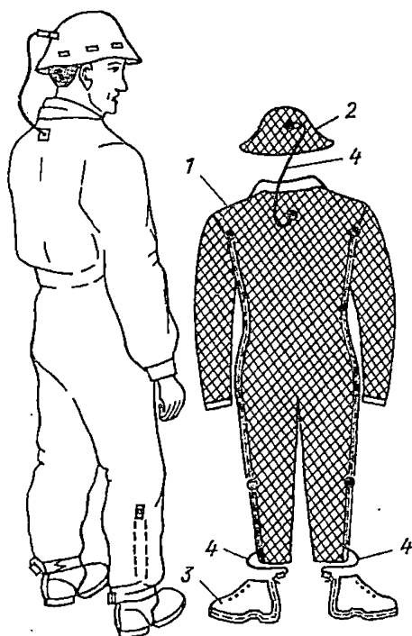
Рис. 11-2. Экранирующая одежда
