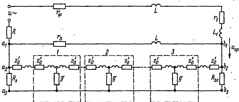
Рис. 9-8. Эквивалентная схема зануляющей системы с распределенными повторными заземлителями
