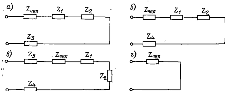
Рис. 6-1 Схемы поражения электрическим током при однополюсном (а, б, в) и двухполюсном (г) прикосновении к токоведущим частям оборудования
