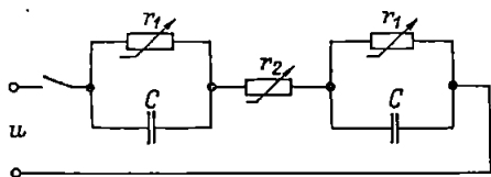
Рис. 6-9. Упрощенная эквивалентная схема
