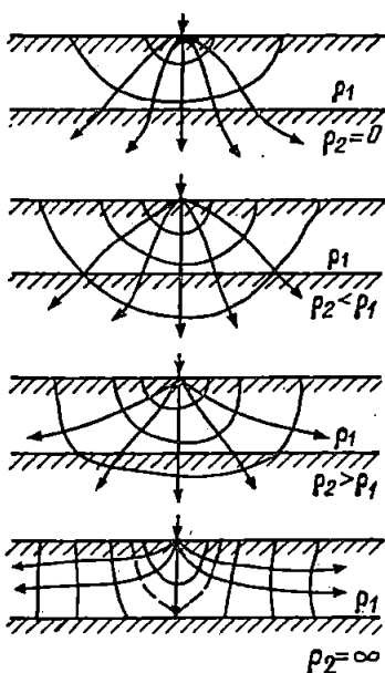
Рис. 10-6. Электрическое поле вокруг точечного электрода при различных значениях удельного сопротивления почвы \rho_1 и подпочвы \rho_2
