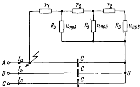
Рис. 4-10. Эквивалентная расчетная схема
