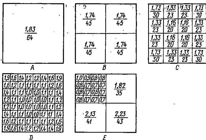
Рис. 10-3. Примеры различных типов выравнивающих сеток Цифры в числителях — произведение коэффициентов k_i k_m , в знаменателях — напряжение по отношению к земле внутри контура в процентах от полного напряжения заземления заземлителя относительно земли
