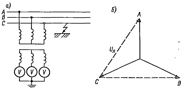
Рис. 8-3. Схема непрерывного контроля за состоянием изоляции в сети напряжением выше 1000 В с изолированной нейтралью (а) и векторная диаграмма к ней (б)
