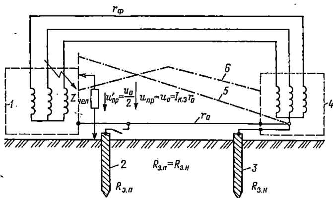
Рис. 9-3. Принципиальная схема зануления для защиты людей от напряжения, возникающего на корпусе оборудования при повреждении изоляции
