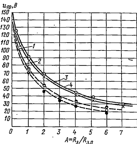
Рис. 9-5. Изменение напряжения прикосновения u_{пр} в зависимости от A — соотношения сопротивлений заземлителей R_z и R_{з.п} при постоянном значении сопротивления заземления повторного заземлителя
