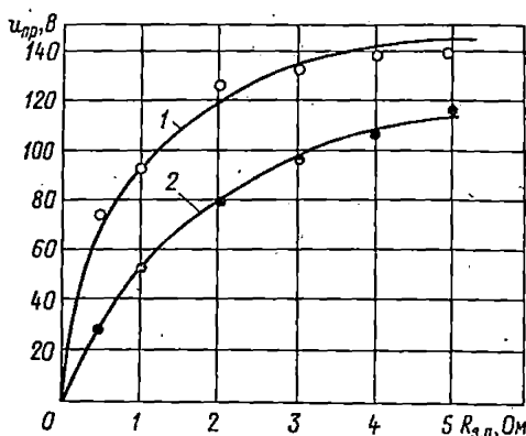
Рис. 9-6. Изменение напряжения прикосновения u_{пр} в зависимости от сопротивления заземления повторного заземлителя R_{з.п} при постоянных параметрах сети 1 — R_3 = 0,5 \text{ Ом} ; 2 — R_3 = 2 \text{ Ом}
