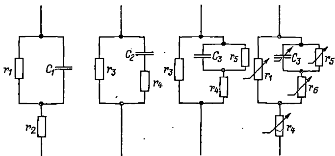
Рис. 6-7. Эквивалентные схемы электрического сопротивления человека по Д. Л. Рубинштейну
