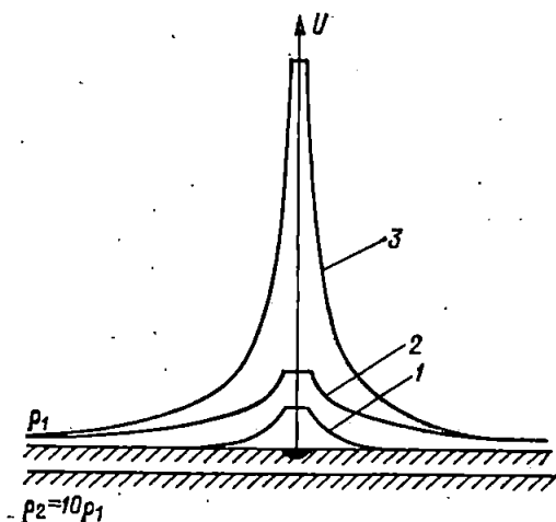
Рис. 10-7. Потенциал вокруг заземляющего электрода
