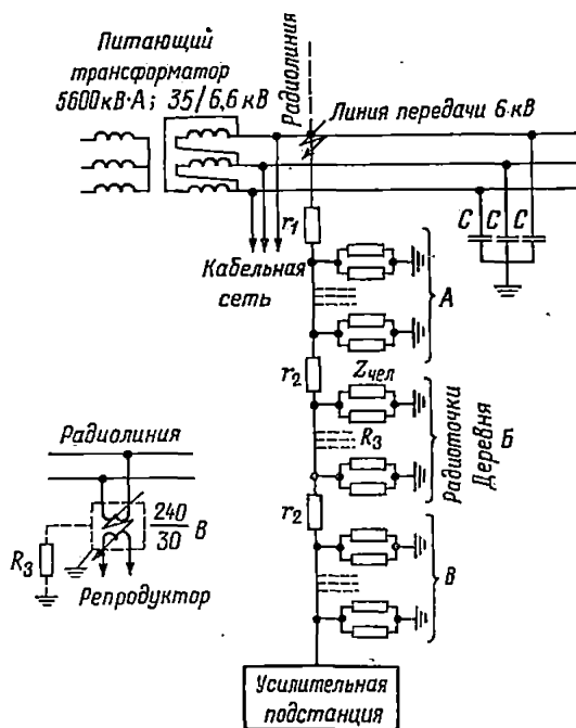
Рис. 4-9. Электрическая схема пересечки
