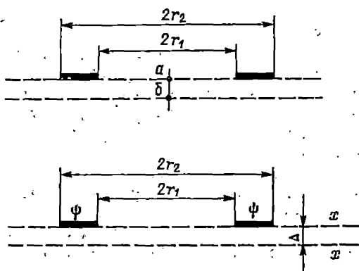
Рис. 7-3. Расчетная схема
