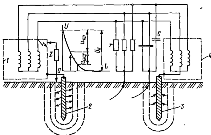
Рис. 9-2. Принципиальная схема заземления для защиты от напряжения, возникшего на корпусе оборудования
