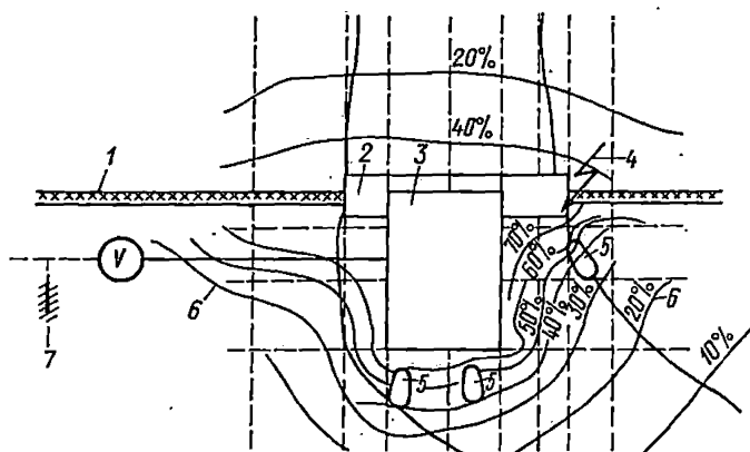
Рис. 4-7. Эквипотенциальные кривые, полученные опытным путем для определения поражающего напряжения 1 — кабель, 2 — металлический лист, наложенный на кабель; 3 — тележка; 4 — место короткого замыкания; 5 — места расположения пострадавших; 6 — эквипотенциальные кривые; 7 — переносные зонды для определения эквипотенциальных областей
