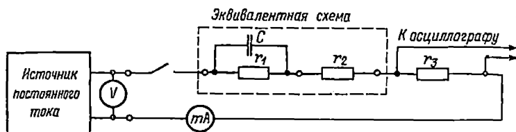
Рис. 6-10. Схема измерения переходного процесса
