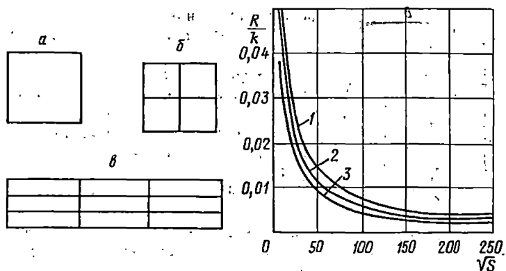
Рис. 10-5. Зависимость сопротивления заземления от площади S , занимаемой заземлителями
