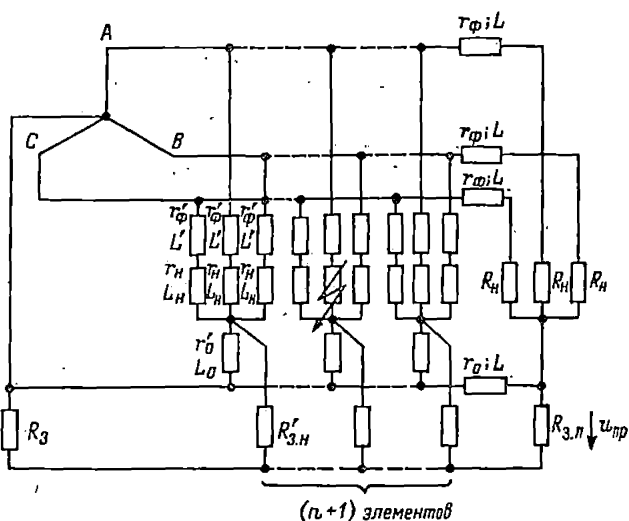
Рис. 9-9. Эквивалентная схема четырехпроводной сети, в которой одновременно используются трех- и четырехжильные кабели
