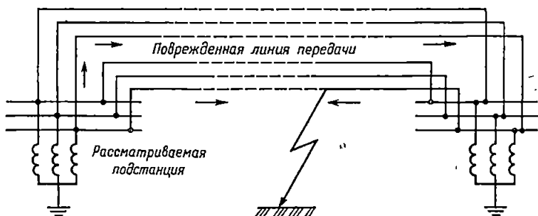
Рис. 10-2. Схема протекания тока при повреждении изоляции вне территории подстанции
