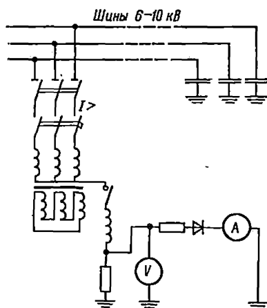
Рис. 8-1. Принципиальная схема испытания электрооборудования и кабелей под нагрузкой
