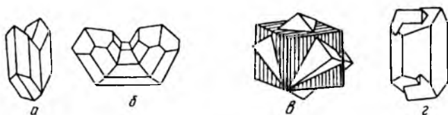
9-расм. Кристалларнинг қўшилиш турлари: a — гипс қўшалоғи; б — рутил уч қўшалоғи, ушиб кириш турлари; в — флюорит қўшалоғи; г — калийли дала шпати қўшалоғи.
