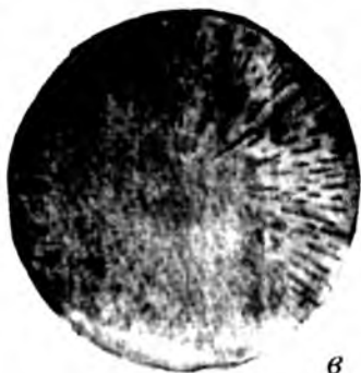
14-расм. Пирит кристаллари: a — донатор массадаги кристаллар; б — турли шаклдаги айрим кристаллар; в — марказнинг радиал шўъласимон конкрецияси.
