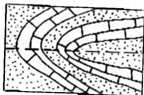
56-рasm. Ётиқ бурма.
