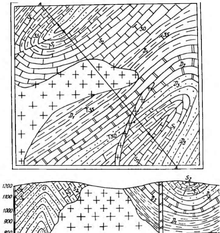
43-расм. Геология харитаси. Масштаб 1 : 1000
