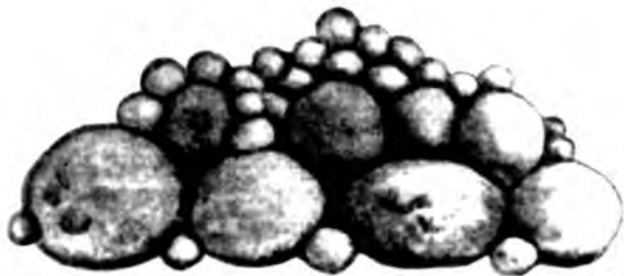
11-расм. Конкреция шакллари. Шарсимон кум конкрецияси.
