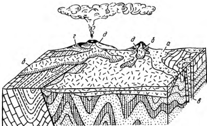
32-расм. Эффузив тоғ жинсларининг жойлашиш шакллари: а — қопламлар; б — оқиқлар; в — некклар; г — сумма; д — конуслар; тўқ чизиқ-бурмалардаги узилмалар.
