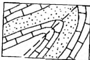
55-рasm. Ағдарма бурма.
