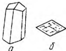
23-рasm. Роговая обманка кристаллари:
