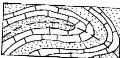
57-рasm. Тункарилган бурма.
