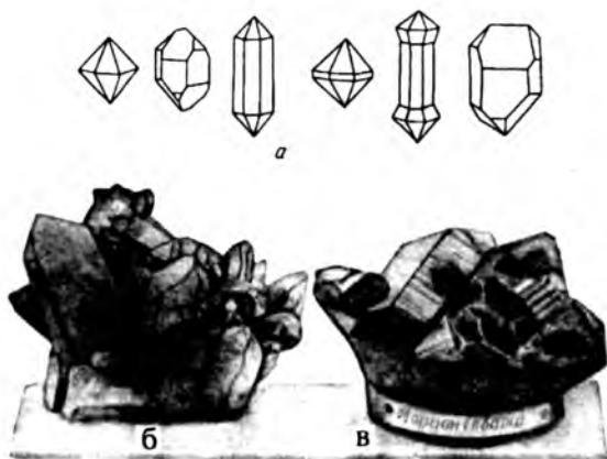
15-рasm. а — кварц кристаллари, кварц друзалари: б — оқ ва в — қора (морион).
