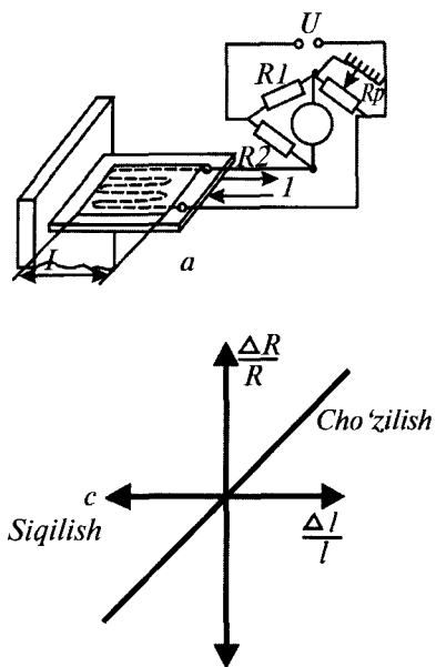
7.5- rasm. Tenzoo'lchagich: a — tenzodatchikning o'rnatilish sxemasi; b — muvozanatlashadigan ko'priq sxemasi; c — tenzoo'lchagichning statik xarakteristikasi.
