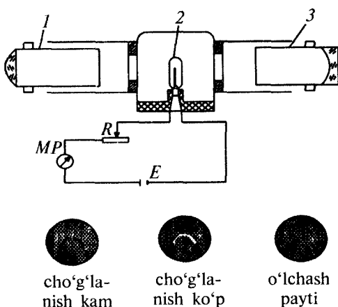
2.24- rasm. Optik pirometrning prinsipial sxemasi.
