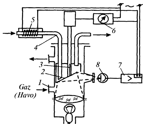
6.50-rasm. Kondensatsion namlik o'lgagichning tuzilish sxemasi.
