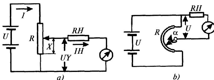
7.1- rasm. Siljishni o'lchaydigan bir tokli potensiometr. a — to'g'ri chiziq bo'yicha surilgichli potensiometr; b — burchak bo'yicha surilgichli potensiometr.
