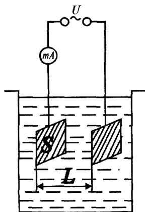
6.18-rasm. Konduktometrning ikki elektrodli o'lchash sxemasi.
