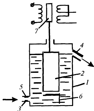
6.32-rasm. Suzib yuruvchi qalqovichli zichlik o'lchagich sxemasi.
