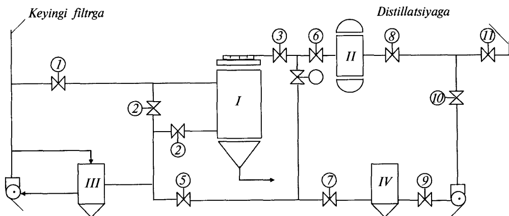
19.3-rasm. Filtrlash jarayonining texnologik sxemasi:
