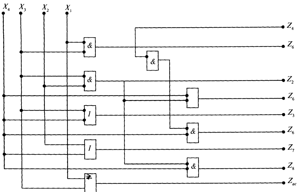
19.8- rasm. Filtrlash davriy jarayonini boshqarish uchun kombinatсион avtomatning prinsipial sxemasi.
