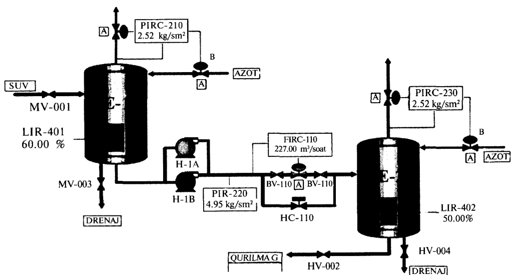
22.2-rasm. „Nasos va klapan“ texnologik uzelingning sxemasi.
