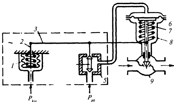
20.2-rasm. Pozitsioner.
