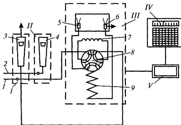
6.16-rasm. Gaz-absorbsion xromatografning sxemasi.
