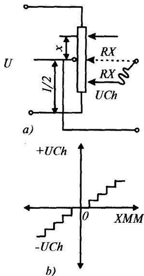
7.2- rasm. Ikki taktli potensiometrlik datchik: a — prinsipial sxemasi; b — yuklamasiz rejimdagi statik xarakteristikasi.
