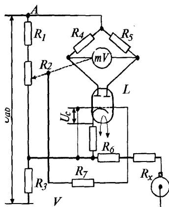
6.52-rasm. Ko'priqli o'lchash sxemasiga ega bo'lgan avtomatik namlik o'lchagich.
