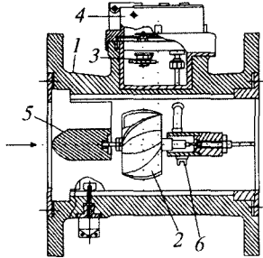
4.14- rasm. Spiralsimon parrakli suyuqlik hisoblagichi.
