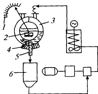
6.43- rasml. Halqali viskozimetr.
