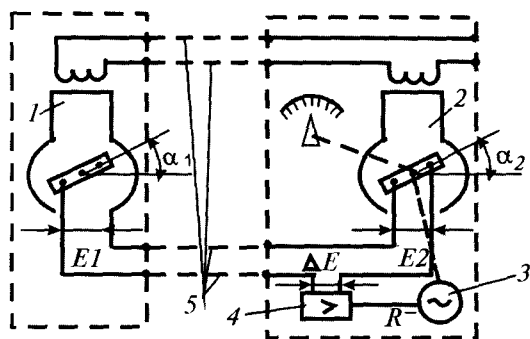
8.5- rasm. Masofaga uzatish ferrodinamik tizimning prinsipial sxemasi.
