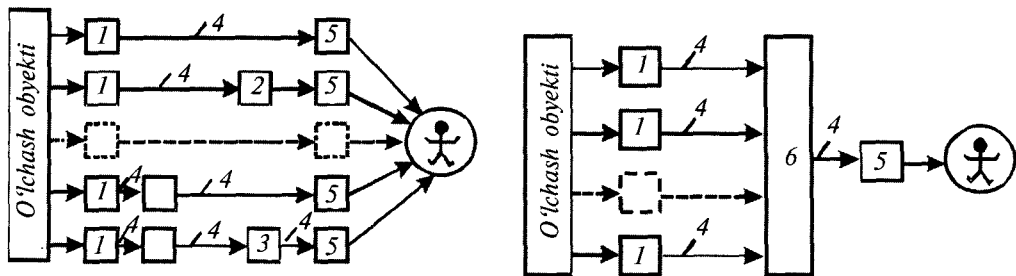
9.6-rasm. O'lchov tizimlarining struktura sxemalari.
