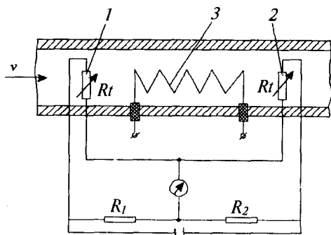
4.10- rasm. Kalorimetrik sarfo'lashgich sxemasi.
