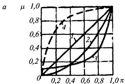
20.5-rasm. Klapaning konstruktiv tavsiflari (a) va diafragmali (b) hamda shlangli (d) klapanlar:
