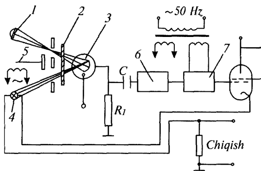
2.25-rasm. Fotoelektr pirometrning prinsipial sxemasi.
