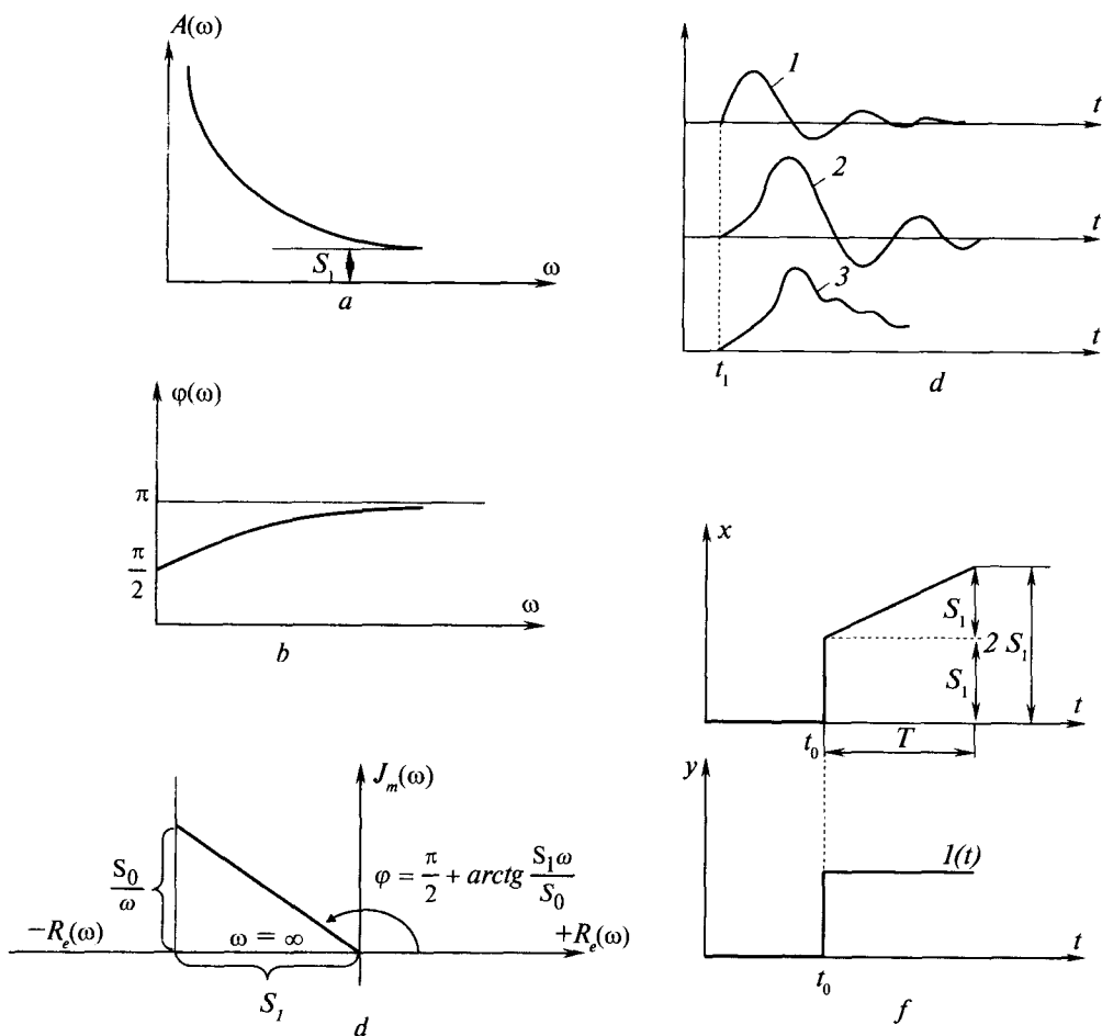
14.3-rasm. PI-rostlagich xarakteristikalar:
