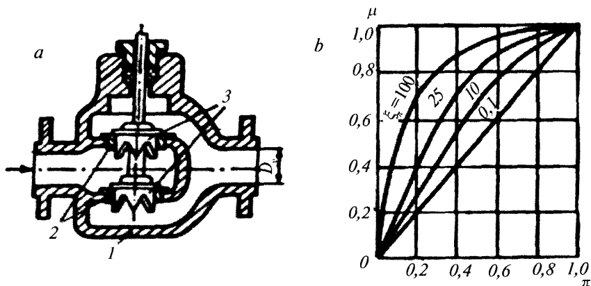
20.4-rasm. Ikki egarli rostlash klapani:
