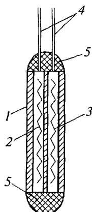
2.14- rasm. Platinali qarshilik termometrlarning sezgir elementi.
