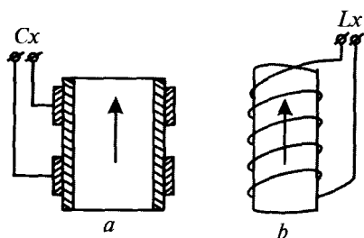
6.22-rasm. Kontaktsiz yuqori chastotali konduktometrning o'zgartkichlari: a — sig'imli; b — induktivli.
