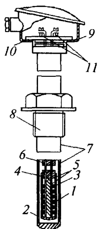
2.15- rasm. Qar- shilik termo- metrlarning tuzilishi.
