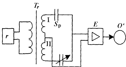
5.10- rasm. Sathni o'lchash elektron indikatorini (EI) ning prinsipial sxemasi.
