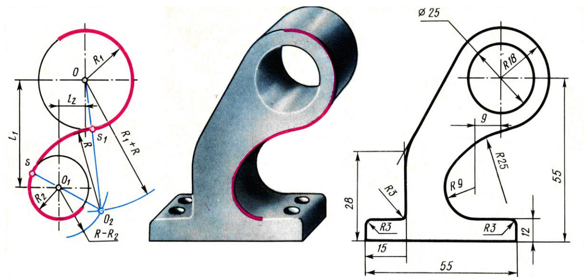
qo‘shiladi va R_1+R radius bilan O_1 markazdan yoy chiziladi (2.30-shakl, a); 2) berilgan O_1 markazli aylana radiusi R_2 ga R radiusni qo‘shiladi va R_2+R radius bilan O_2 markazdan yoy chiziladi. Shunda ular kesishib izlanayotgan tutashma markazi O ni hosil qiladi (2.30-shakl, a); 3) endi, O ni O_1 va O_2 ni O bilan tutashtirib o‘tish nuqtalari A va B larni aniqlanadi (2.30-shakl, b). Sirkul ignasini O nuqtaga qo‘yib A va B larni R radiusli yoy bilan tutashtiriladi (2.30-shakl, b). 2.31-shaklda bu tutashma turlariga misollar keltirilgan.
