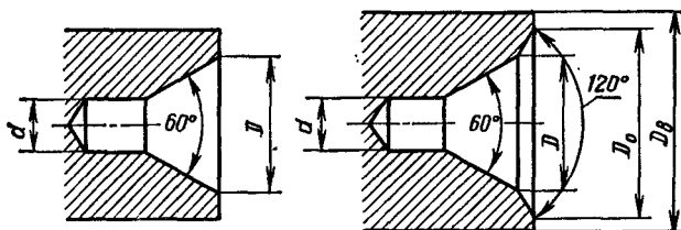
9.3-rasm. Markaziy teshiklar.
