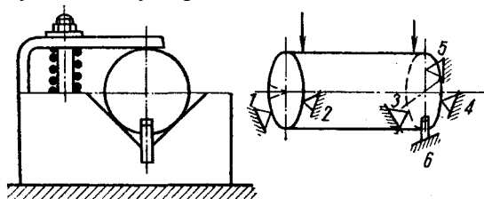
2.3-rasm. TSilindrik Detalning prizmada bazalash sxemasi:
