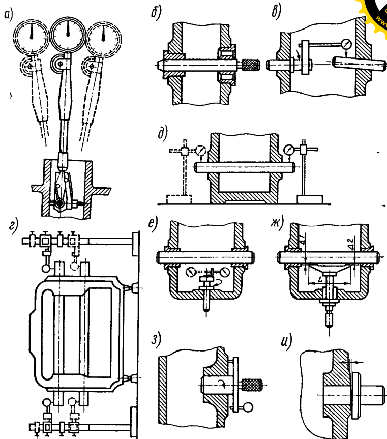
8.9-rasm. Qutisimon detallarni nazorat qilish usullari:
