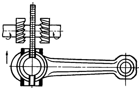
11.2-rasm. SHatun qopqog'ini qirqib olish hamda bolt va gayka osti Yuzalarini frezerlash
