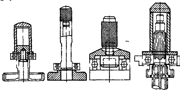
14.1-rasm. SHarikli podshipniqlarni vallarga presslash uchun opravka va stakanlar
