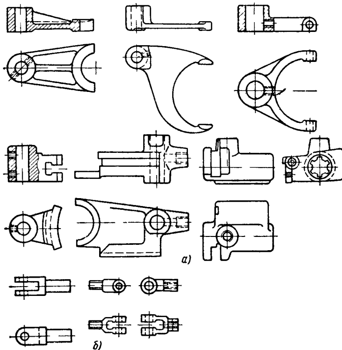
10.1-rasm. Ilgaklar turidagi detallar.
