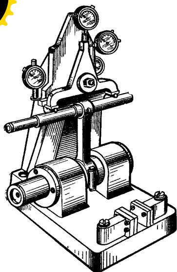
11.6-rasm. SHatunning krivoship va porshen kallaklaridagi teshiklarini o'qlararo masofasi hamda o'qlarning o'zaro parallelligini nazorat qilish moslamasi
