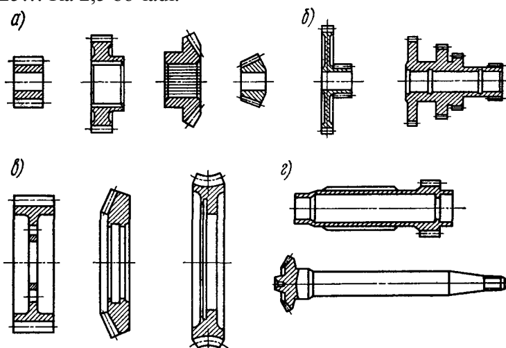
12.1-rasm. Tishli qildiraklarning turlari.
