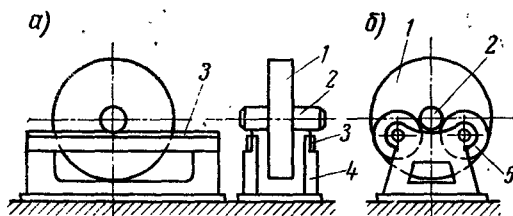
14.5-rasm. Detallarni statik muvozanatlash uchun qurilma:
