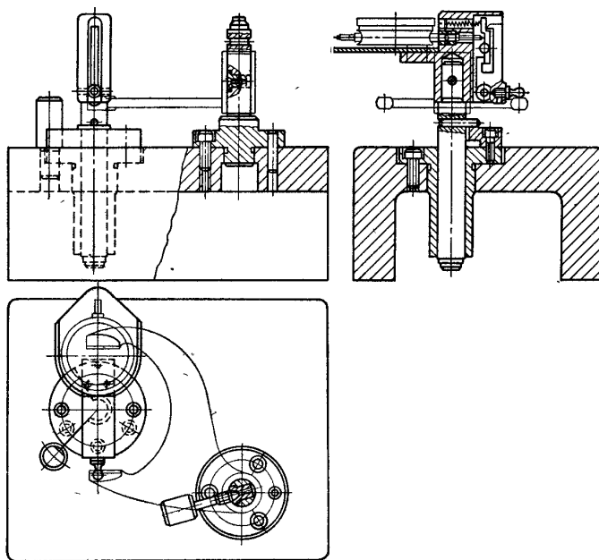
10.2-rasm. Ilgakning ishchi Yuzalarini o'zaro joylashishini nazorat qilish.
