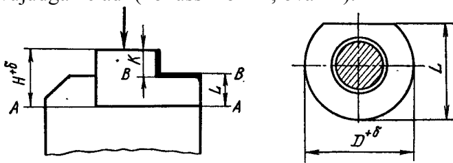
3.1-rasm. Detallarni tekis va tsilindrik Yuzalari bo'yicha o'rnatish
