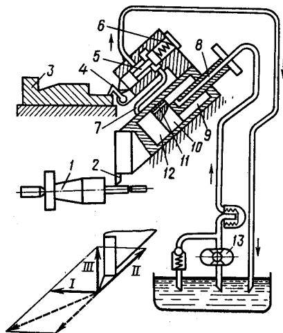
9.5-rasm. Tokarlik-gidrokopirlash dastgohlarida shpindel pog'onalariga ishlov berish jarayoni.
