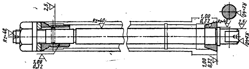
9.6-rasm. Bo'ylama yo'nalishda ochiq teshiklarga ega bo'lgan shpindel uchun ikki konusli asos (opravka).
