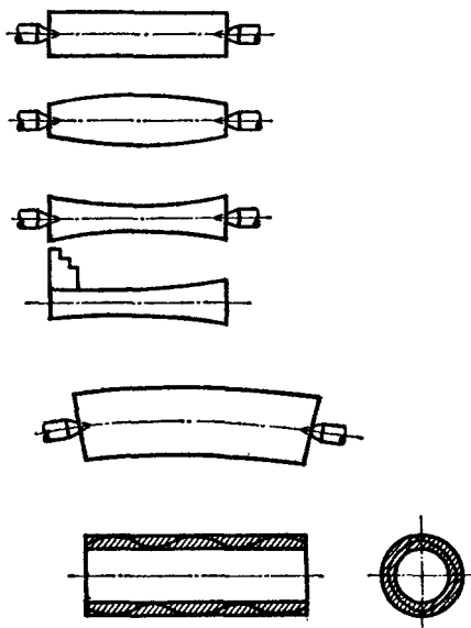
3.2-rasm. TIBT ning deformatsiyasi natijasida to'g'ri geometrik shakldan og'ishi hollari.
