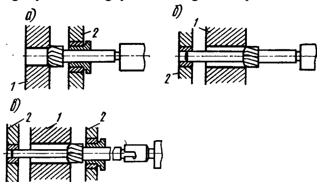
8.6-rasm. Qutisimon detallarni teshiklariga ishlov berish jarayonida kesuvchi asboblarni yo'naltirish usullari:
