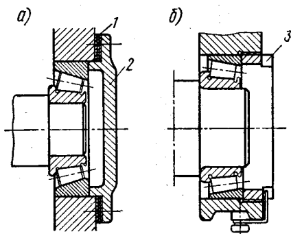
14.2,a-rasm. Konussimon rolikli podshipniklarda radial oraliqni moslash usullari: a) prokladkalar yig'masi yordamida (qo'zg'almas kompensator); b) halqasimon gayka yordamida (qo'zg'aluvchan kompensator)
