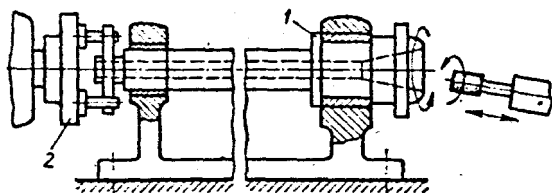
9.7-rasm. SHpindelni konus teshigini ichki Yuzalarini jilvirlash dastgohida ishlov berish jarayoni: 1-o'ratish halqasi; 2- povodokli qurilma.
