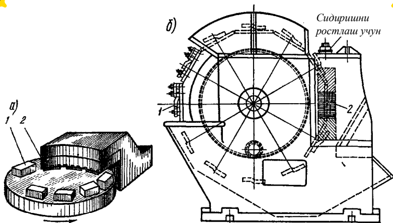
8.4-rasm. Tekis Yuzalarni uzluksiz sidirish usullari:
