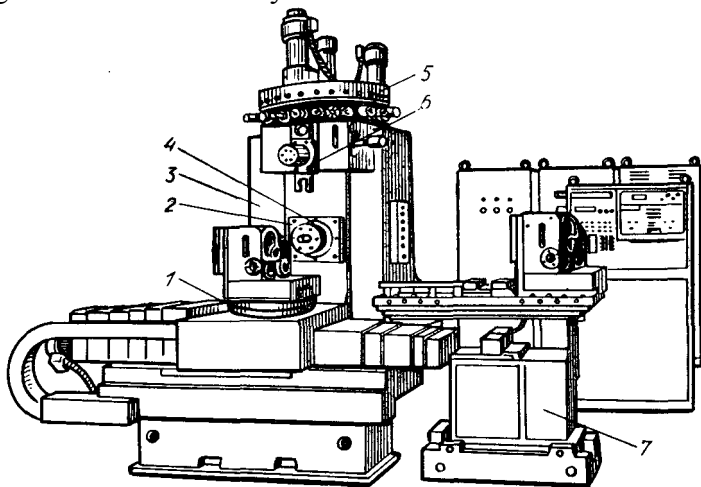
8.7-rasm. Ko'p vazifali dastgox (ishlov berish markazi)ning IR500MF4 modeli:
