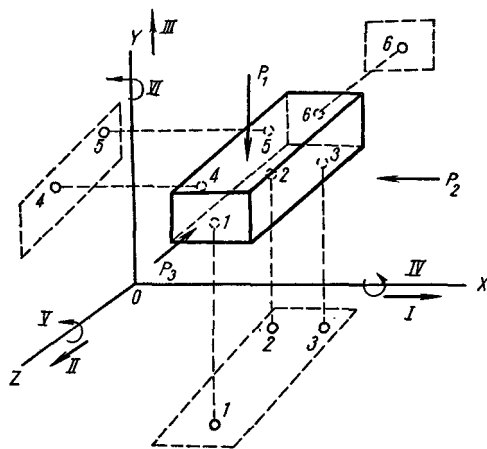
2.2-rasm. Detailarni bazalash sxemasi (olti nuqta qoidasi): R1,R2,R3- Detailning bazalashda ta'sir etuvchi kuchlar.
