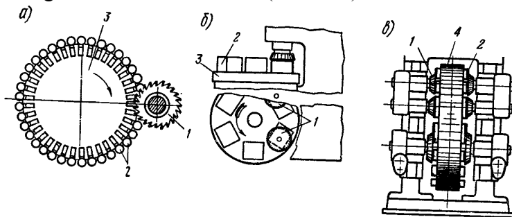
8.3-rasm. YUzalnarni uzluksiz frezerlash jarayonlari:
