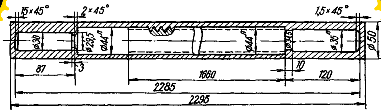
5.3-rasm. Prokatdan olingan vint xomashyosi.
