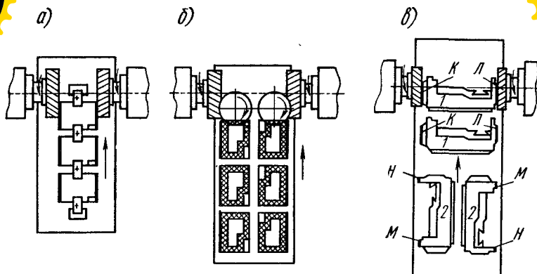
8.2-rasm. Bo'ylama- frezerlash dastgohlaridan Yuqori unumli ishlov berish usullari.
