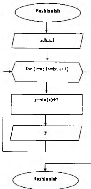
6.16-rasm. Dastur blok sxemasi.
