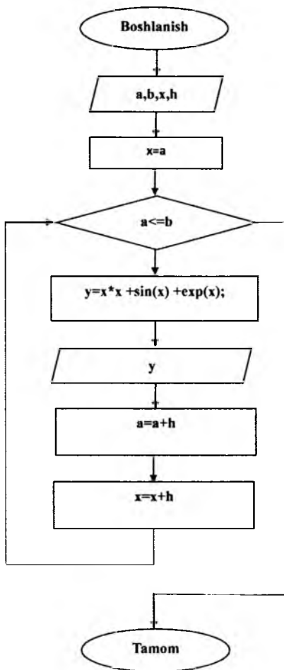
6.4-rasm. Dastur blok sxemasi.
