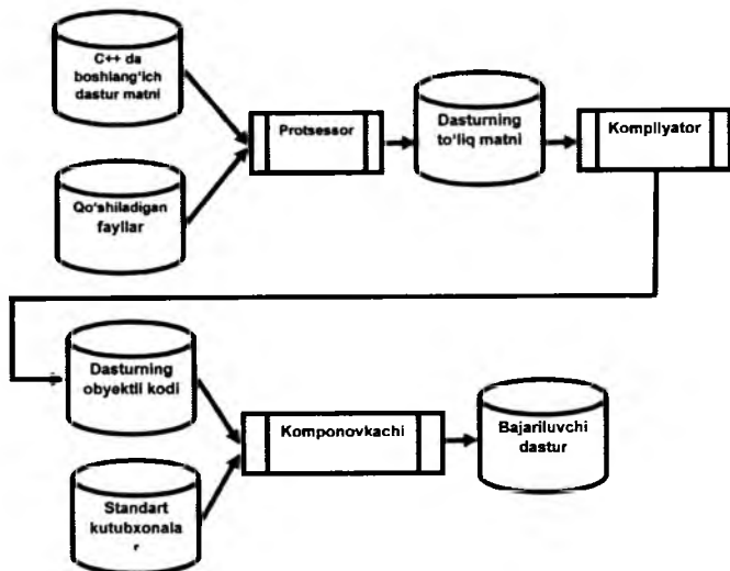
3.1-rasm. Dasturni qayta ishlash jarayonlari.
