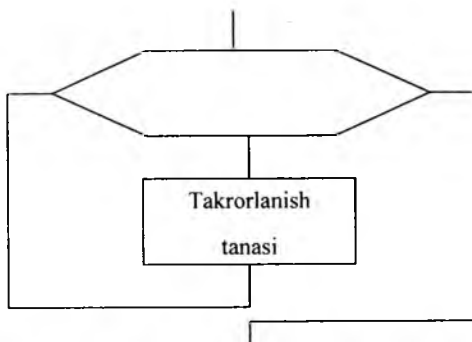
6.12-rasm. Parametrli takrorlanish algoritmi.
