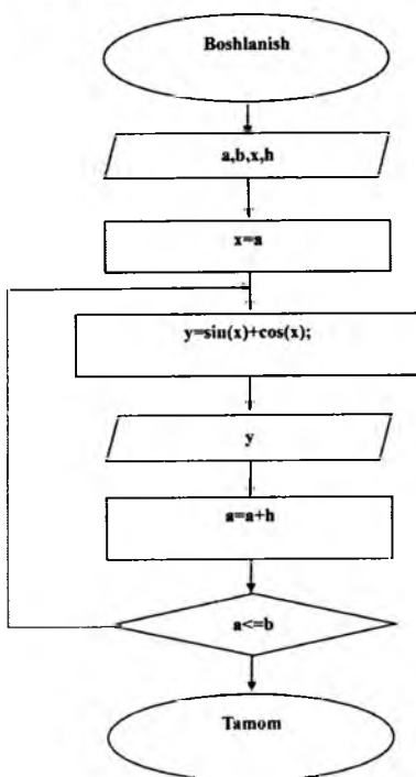
6.9-rasm. Dastur blok sxemasi.
