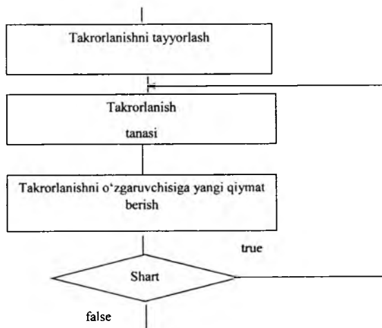
6.7-rasm. Sharti keyin tekshiriladigan takrorlanish algoritmi.
