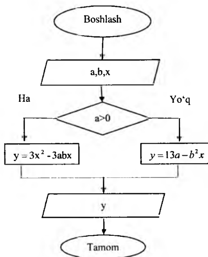
5.2-rasm. Dastur blok shemasi.
