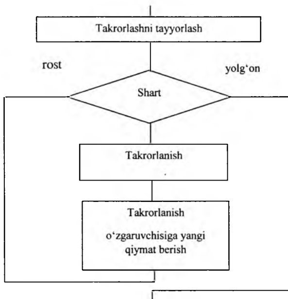
6.1-rasm. Avval sharti tekshiriladigan takrorlanish algoritmi.
