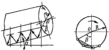
6-rasm. Barabanli elaklarning sxemasi.
