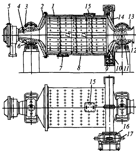
20-rasm. Markaziy bo'shatiluvchi sharli tegirmon:
