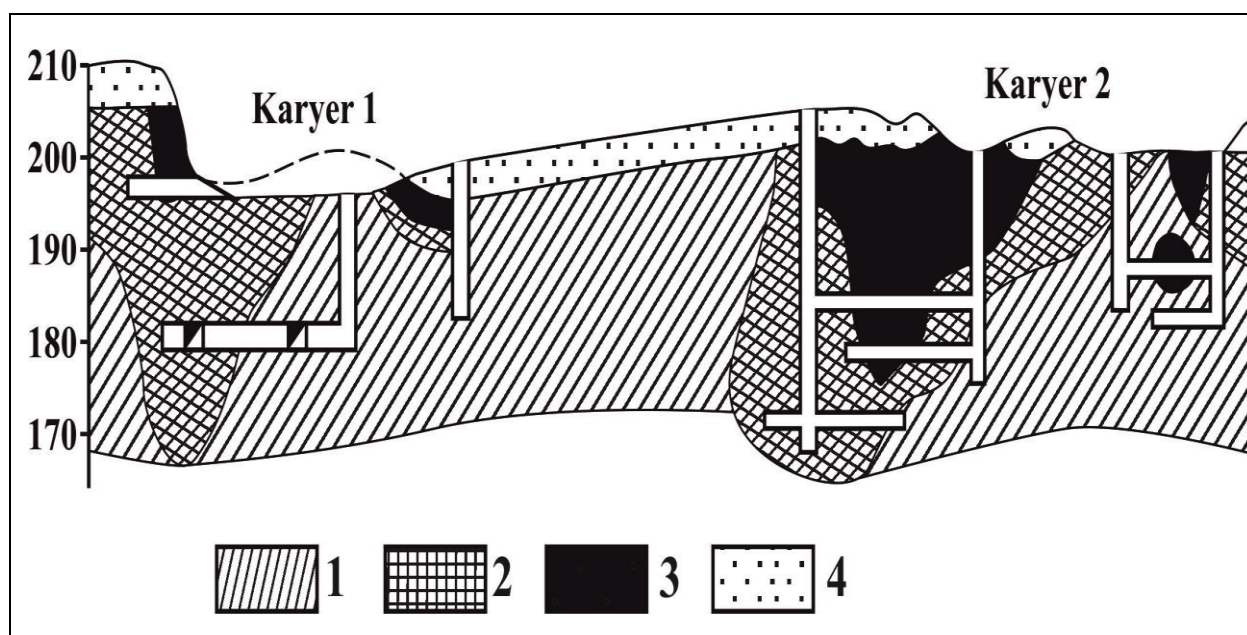
6.2-rasm. Rassehkali qidirish shurflari tizimi. 1-ikkilamchi kvarsit; 2-andaluzitli tog‘ jinslari; 3-korund uyumlari; 4-delyuviy.
