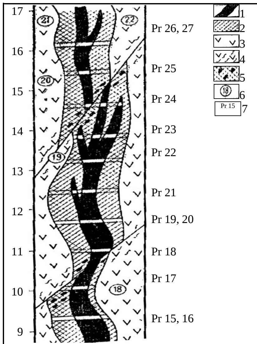
7.4-rasm. Yuqoriga yo'nalgan tog' inshooti devorining chizmasi. 1-ma'dan tomiri; 2- o'zgargan ma'danli tog' jinslari; 4-brekkchiyalashgan tog' jinslari; 5-brekkchiyalashgan ma'dan zonasi; 6-kichik namunacha olingan joy; 7-namunalarning tartib raqami.
