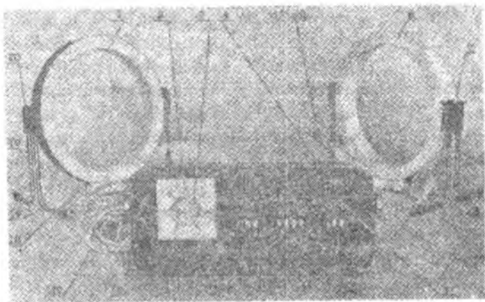
3.30-rasm. Apparatning ish holatidagi umumiy ko'rinishi: 1 – induktor «2»; 2 – muolaja soati; 3 – muolaja soatining tarmoq dastagi; 4 – tarmoq indikatori; 5 – elektron bloki; 6 – induktor «1»; 7 – solenoid aylanish kuchlanishini rostlovchi vint; 8 – induktor «1» ning kabeli; 9 – induktor chiqish kabeli uchun himoya qopqog'i; 10 - fiksator; 11 – induktor «2» ning magnit maydon indikatori; 12 – «INDUKTOR» pereklyuchateli; 13 - induktor «1» ning magnit maydon indikatori; 14 – «INTENSIVLIK» pereklyuchateli; 15 – ish tartibi (rejimi) pereklyuchateli; 16 – apparatni olib yurish dastagi; 17 – tarmoq shnuri; 18 – induktor «2» kabeli; 19 – solenoid oyoqchalari; 20 – kolodka
