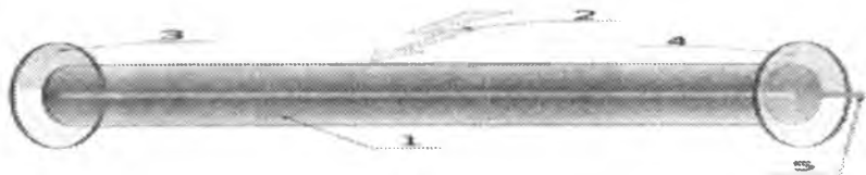
3.7-rasm. Geliy – neonli lazerning kvartsl gaz razryadli trubkasining umumiy ko'rinishi: 1- ishchi muhit, 2- lazer nurini hosil qiluvchi energiya, 3-tiniqmas ko'zgu, 4- yarim tiniq ko'zgu, 5-lazer nuri
