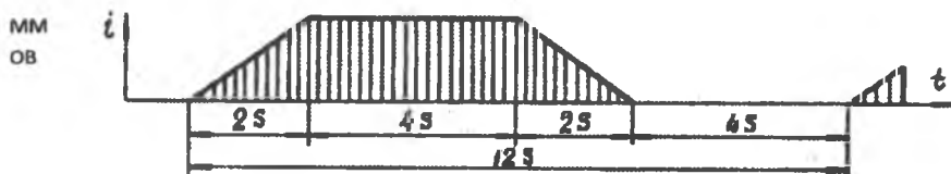
3.20-rasm. Bir yarim davrli to'liqinli (OB) – OH ko'rinishidagi tok impulslari seriyasi, egiluvchan bo'lib noldan maksimal darajagacha ko'tarilib, bu qiymatni ma'lum vaqtgacha saqlaydi, so'ngra yana qaytib nolgacha tushadi
