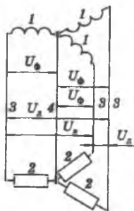
2.4-rasm. Uch fazali tok sistemasini ulash sxemasi: 1 – bitta generatorning faza o'ramlari, ularda o'zgaruvchan kuchlanish induksiyanadi; 2 – nagruzkalar (iste'molchilar); 3 – chiziqli simlar (ular generatorni iste'molchi bilan birlashtiradi); 4 – neytral (nol) simi
