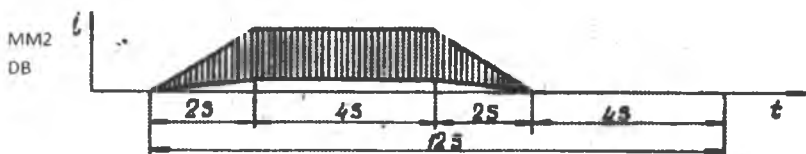
3.21-rasm. Ikki yarimdavrlı to'liqinli (DB) – DH ko'rinishidagi tok impulslari seriyasi, egiluvchan bo'lib qaysiki noldan maksimal darajagacha ko'tarilib, bu qiymatni malum vaqtgacha saqlaydi, so'ngra yana qaytib nolgacha tushadi
