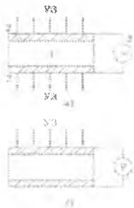
2.34-rasm. Teskari (a) va to'g'ri (b) pyezoelektrik effektga asoslangan elektromexanik nurlantirgich va priyomnik sxemasi
