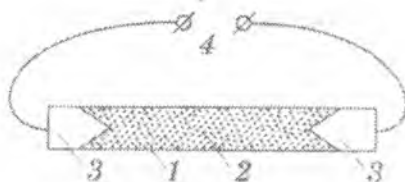
2.11-rasm Rezistivli oddiy – nafas olish datchigining sxematik ko'rinishi
