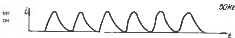
3.15-rasm. Bir yarim davrli uzluksiz (OH) - 50 Gts chastotali eksponensial qirqimli sinusoidal formadagi tok impulsarlari
