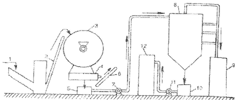
2.3-расм. Ўсимликларнинг вегетатив массасидан озуқа учун оксил концентрациялари олиш технологиясининг чизмаси
