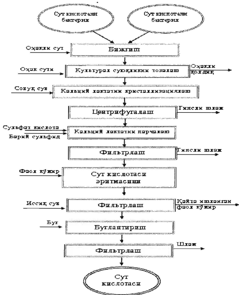
5.5-расм. Сут кислотаси олишнинг технологик чизмаси
