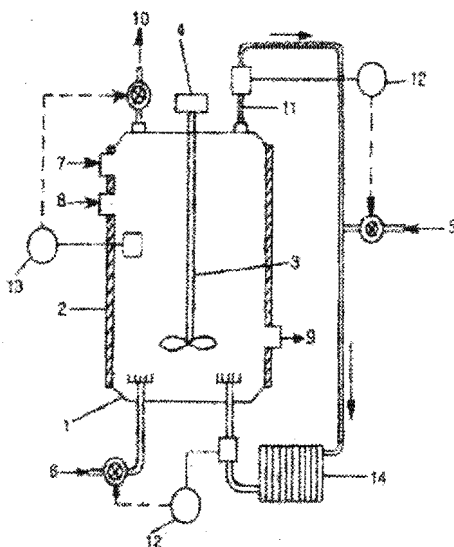
6.2-расм. Газсимон углеводородларда микроорганизмлар ўстириш учун ферментёр
