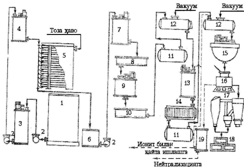
5.3-расм. Меласса сақловчи муҳитда лимон кислота олишининг технологик чизмаси
