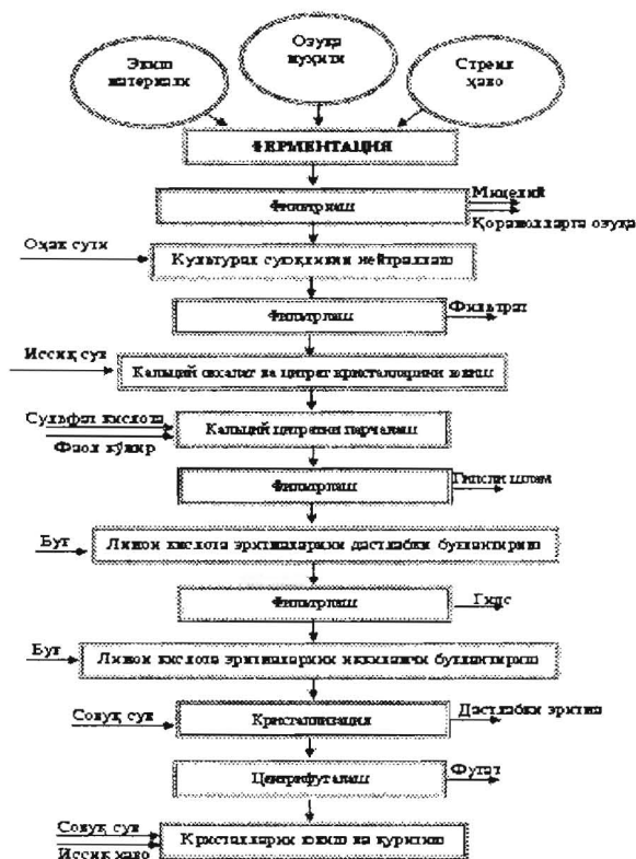
5.3-расм. Лимон кислота ишлаб чиқаришнинг технологик чизмаси
