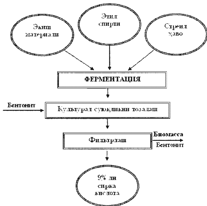
5.1-расм. Сирка кислота ишлаб чиқаришнинг технологик чизмаси
