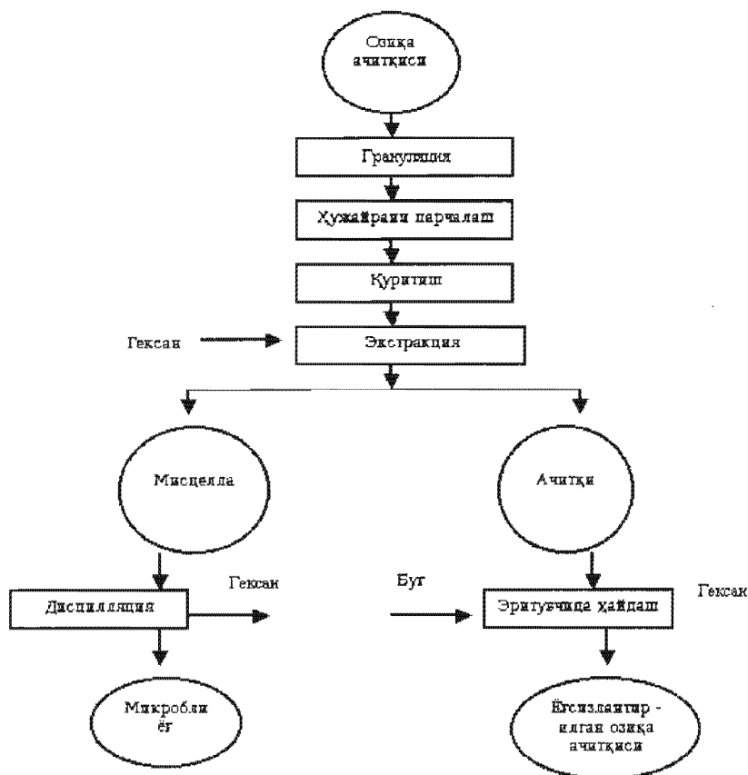
7.4-чизма. Липид олиш технологиясининг чизмаси
