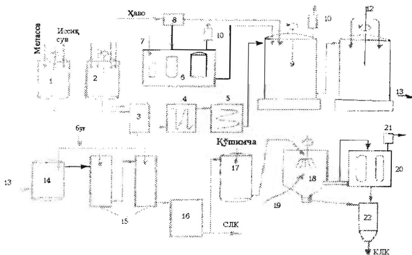
6.5-расм. Лизин концентрати ишлаб чиқариш технологиясининг чизмаси:
