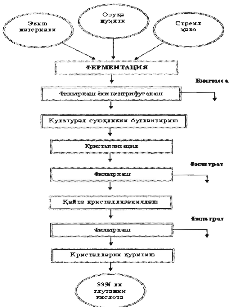
4.3-расм. Глутамин кислота ишлаб чиқаришнинг технологик чизмаси
