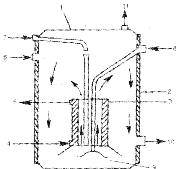
6.1-расм. Ачитқи замбуруғини суюқ муҳитда ўстириш учун ферментёр
