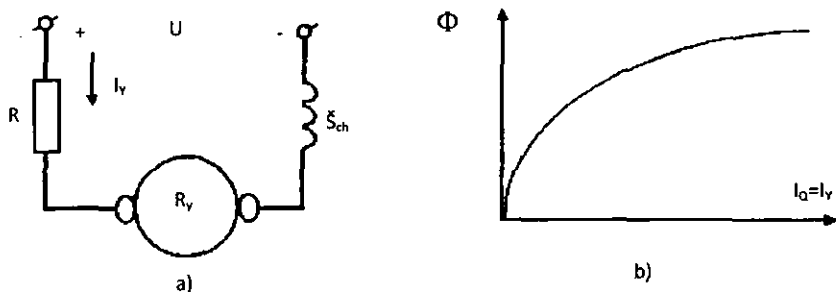
5.12-rasm. Ketma-ket qo'zg'atkichli O'TM:
