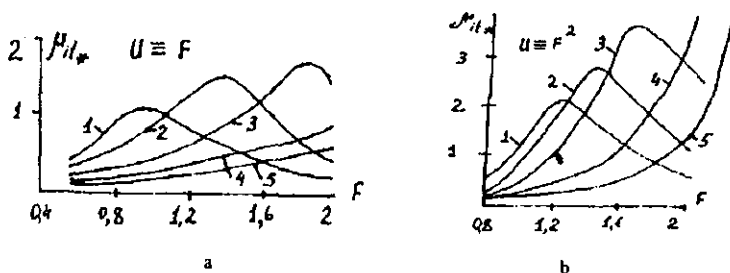
6.22-rasm. BΦKAMning ishga tushirish momentlari:
