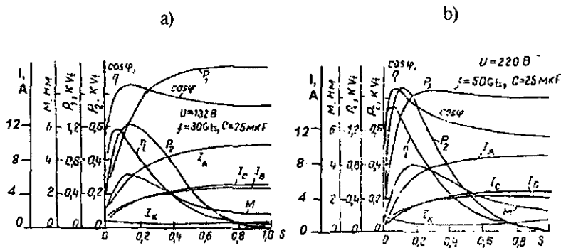
6. 20-rasm. Uchburchak sxemada ishlovchi BFKAM ishchi tavsiflari: a— f = 30 Gts da b— f = 50 Gts da.
