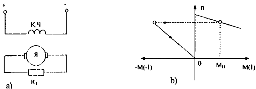
7.3-rasm. O'TMni elektrodinamik tormozlash:
