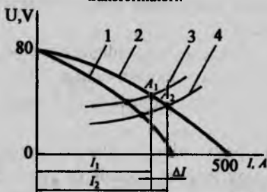
3.5-rasm. Ta'minlovchi manbalarning volt-ampér tavsifi (1 va 2) va flyus ostida payvandlash turida uzunlikdagi (3 va 4) payvandlovchi yoyning tavsifi.
