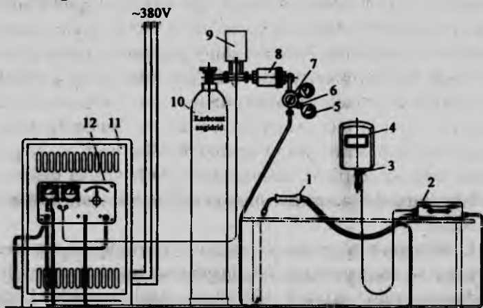
6.1-rasm. Karbonat angidrid gazi muhitida ingichka elektrod sim bilan yarimavtomatik payvandlash postining sxemasi: 1 – tutqich, 2 – uzatuvchi mexanizm, 3 – ishga tushirish tugmasi, 4 – ihota shchitchasi, 5 – 6 atmgga mo'ljallangan manometr, 6 – manometrni o'rnatish uchun o'tish shtutseri, 7 – yuqori bosim manometri bilan birga kislorod reduktori, 8 – gaz quritgich, 9 – gaz isitkich, 10 – karbonat angidridli ballon, 11 – payvandlash to'g'rilagichi (yoki generatori) 12 – boshqarish pulti.
