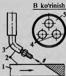
8.6-rasm. “Yuvish” yordamida kesish sxemasi:
