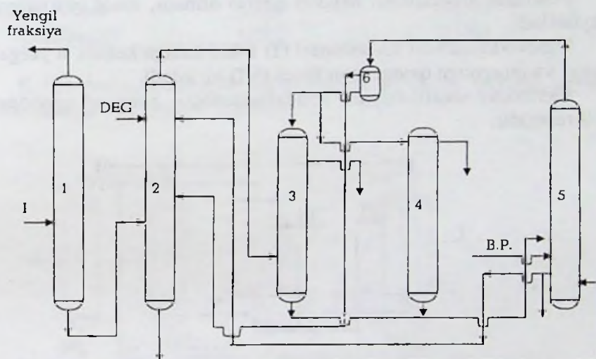
9-rasm. Riforming katalizatidan aromatik uglevodorodlarni dietilenglikol (DEG) yordamida ekstraksiyalash prinsipial sxemasi: 1-xomashyo tayyorlash rektifikatsion kolonnasi; 2-ekstraksiyon kolonna; 3-dearomatizatsiyalangan katalizatni yuvish kolonnasi; 4-dearomatizatsiyalangan katalizat kolonnasi; 5-bug'latish kolonnasi; 6-haydab ajratib olingan mahsulotlar priemnigi.
