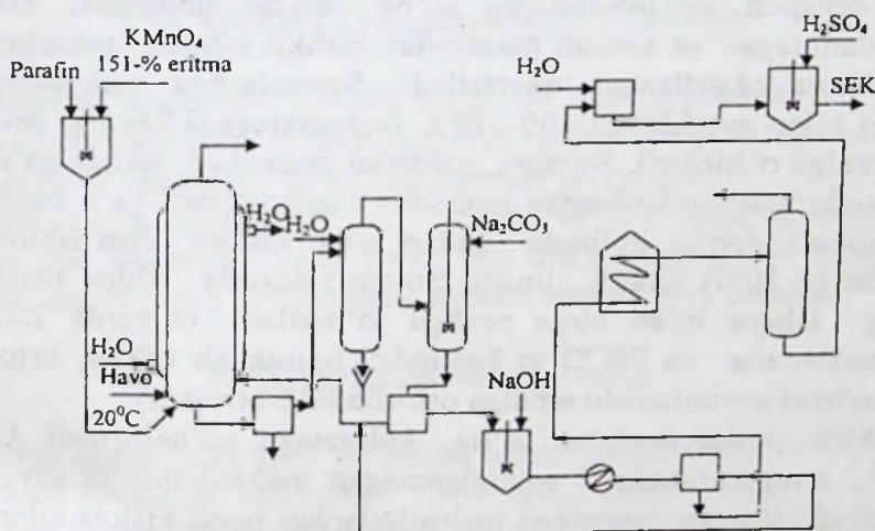
13-rasm. Sintetik yog' kislotalarini olish prinsipial texnologik sxemasi.
