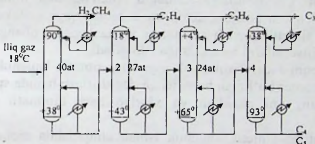
7-rasm. Gazlarni quyi temperaturali rektifikatsiya yo'li bilan ajratishni prinsipial sxemasi:
