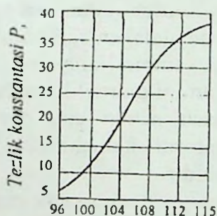
1-rasm. Fosfat kislotasining konsentratsiyasi, % Propilenning polimerlanish reaksiyasi tezligining fosfat kislota konsentratsiyasiga bog'liqligi.
