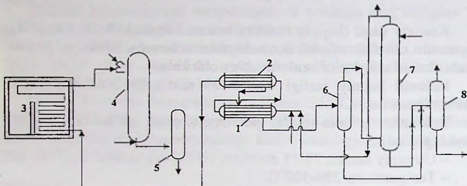
15-rasm. Etilenni to'g'ridan-to'g'ri gidratatsiyalab etil spirti ishlab chiqarish prinsipial texnologik sxemasi.
