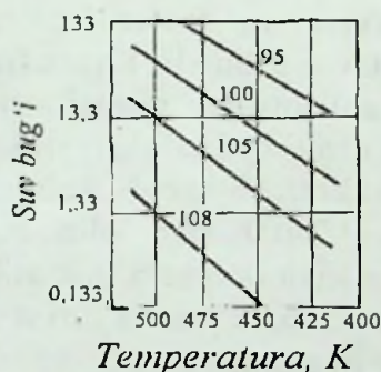
2-rasm. Fosfat kislotasi eritmasiga ustidagi to'yingan suv bug'ining bosimining temperaturaga bog'liqligi. To'g'ri chiziqlardagi raqamlar- kislotaning konsentratsiyasi.
