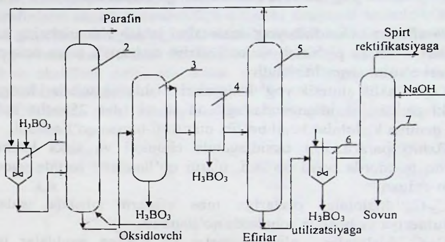
12-rasm. Suyuq parafinlarni oksidlab spirtlar ishlab chiqarish prinsipial texnologik sxemasi.
