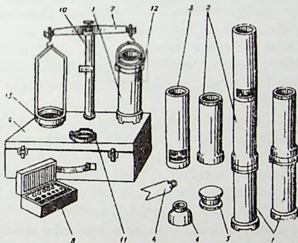
36-rasm. Donning asl og'irligini aniqlaydigan litrli purka:
