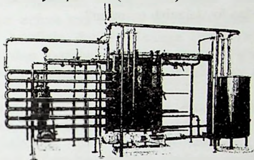
25-rasm. Tindirilgan olma sharbatini pasterizatsiyalovchi qurilma
