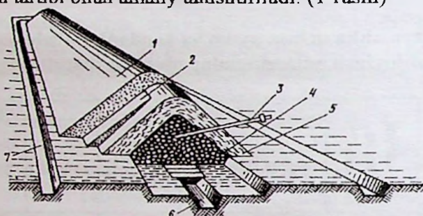
1-rasm. Kartoshka saqlanadigan uyumni tashkil qilish sxemasi:
