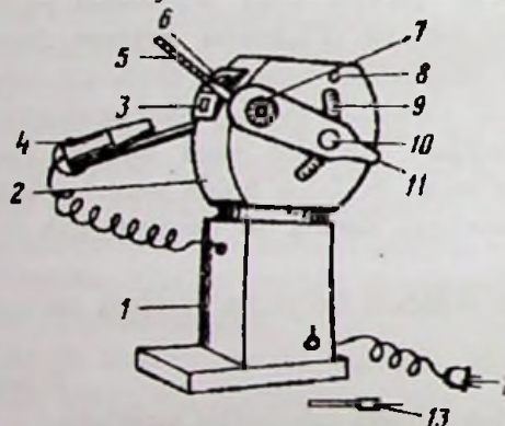
11- usm. Refraktometr: 1-asosi; 2-korpus; 3-quyi linzaning oynasi; 4-yoritgich; 5-termometr; 6- yuqori linza oynasi; 7-linb; 8-nol- punkt o'rnatish kaliti tirgishi; 9- shkala; 10-okulyar; 11-okul-yarni burish ushlagichi; 12-shtepsel; 13- nol-punktini tuzatish kaliti.
