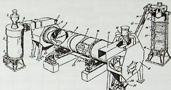
39-rasm. SZSB-8 don quritgichining umumiy ko'rinishi:
