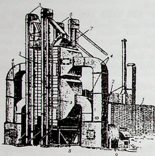
37-rasm. SZSh-8 don qurtgichi (umumiy ko‘rinishi):
