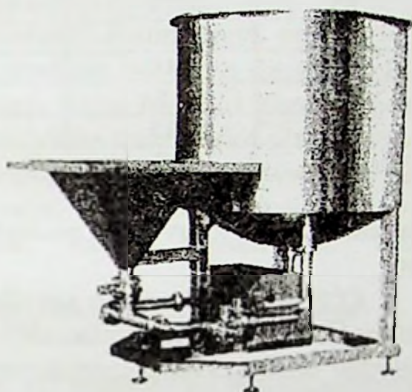
15-rasm. Marinad suyuqligi tayyorlanadigan uskuna
