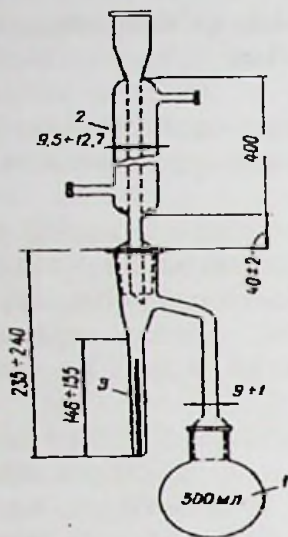
45-rasm. Din va Stark apparati:
