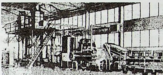
22-rasm. Tomat halimi ishlab chiqariluvchi texnologik tizim
